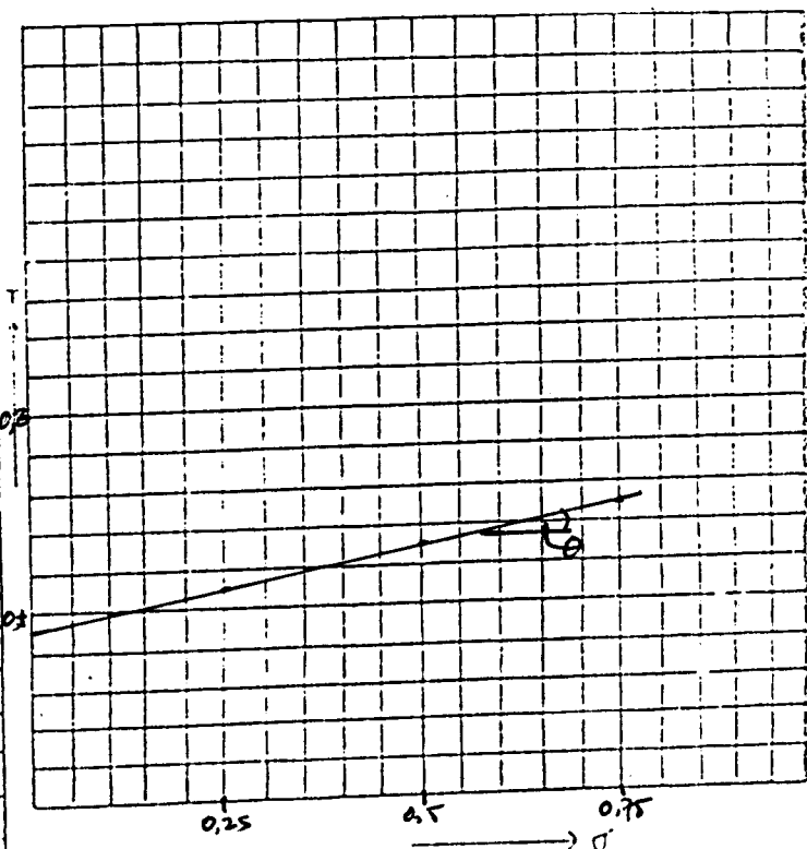
KEKUATAN GESER LANGSUNG (DIRECT SHEAR)
