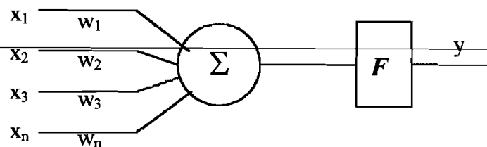
Gambar 2.4 Informasi pemrosesan pada artificial neural network
