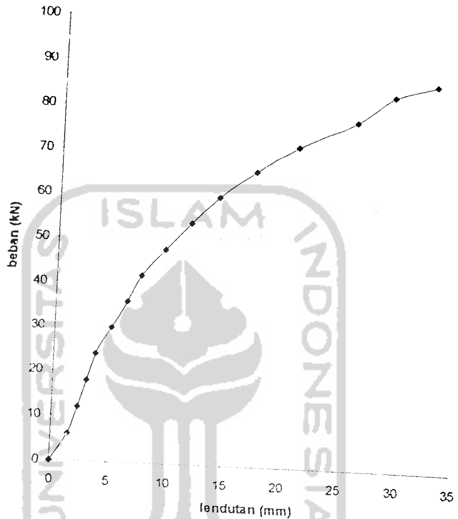
Gambar I.3.2 Grafik hubungan beban-lendutan sample 2
