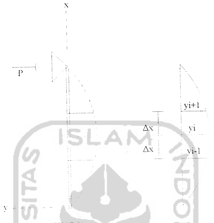
Gambar 3.13 Penurunan yang terjadi akibat beban (P)
