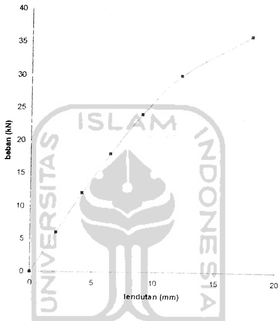
Gambar L3.8 Grafik hubungan beban-lendutan sample 4
