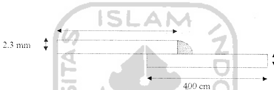
Gambar 4.7 Benda Uji Untuk kuat Tarik Las
