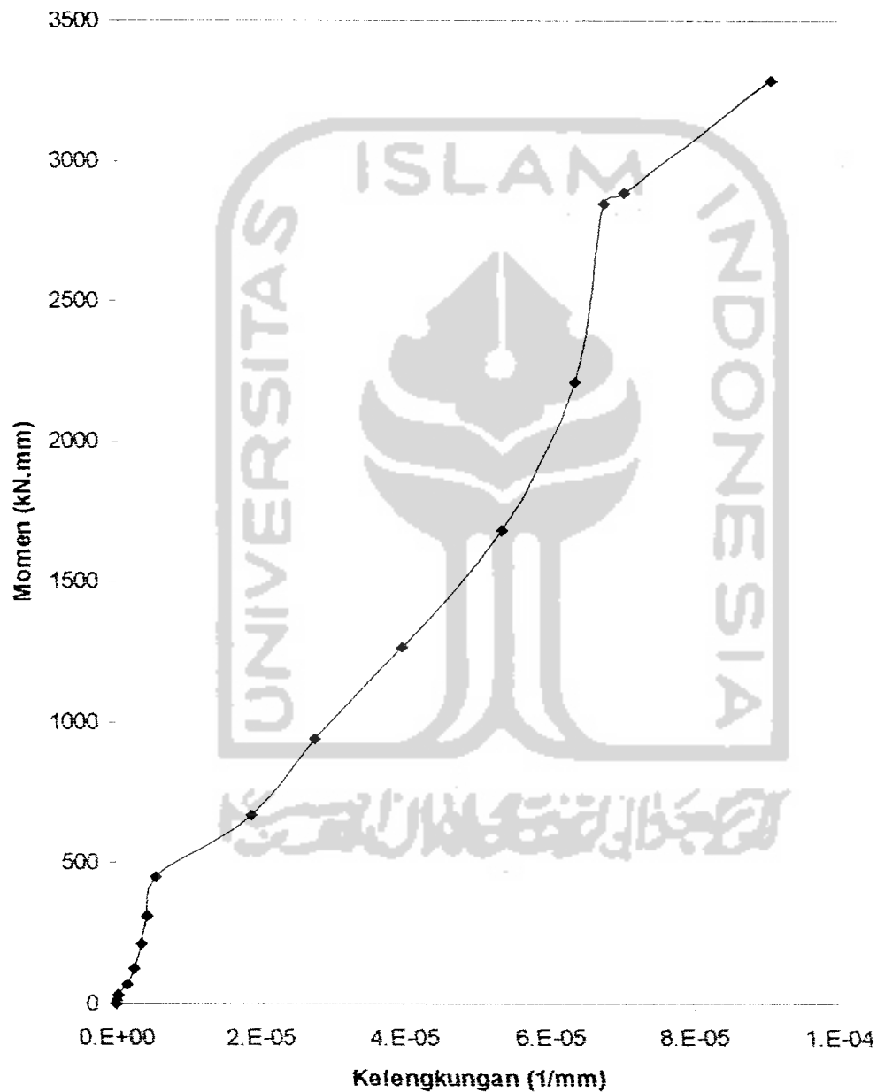
Gambar 5.9 Grafik perbandingan momen-kelengkungan pada sampel I
