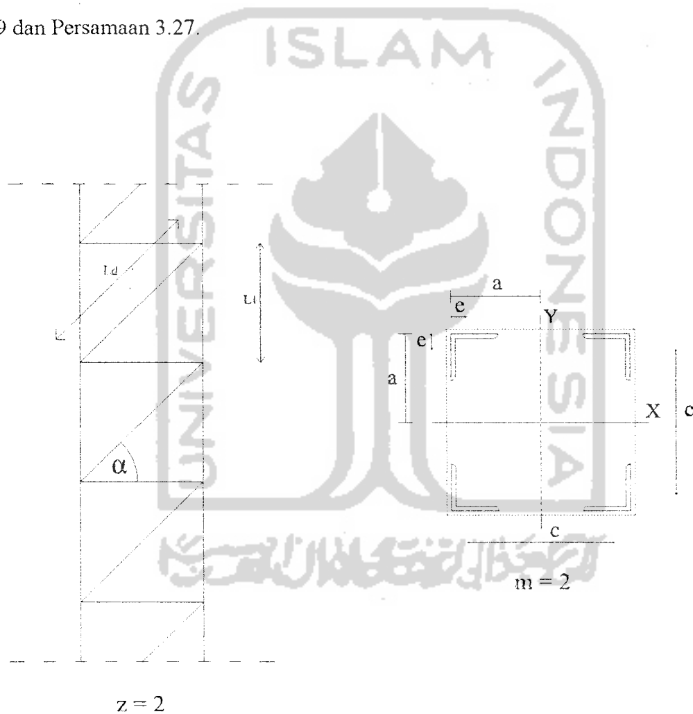
Gambar 3.9 kolom tersusun yang dihubungkan dengan perangkat transversal dan diagonal
