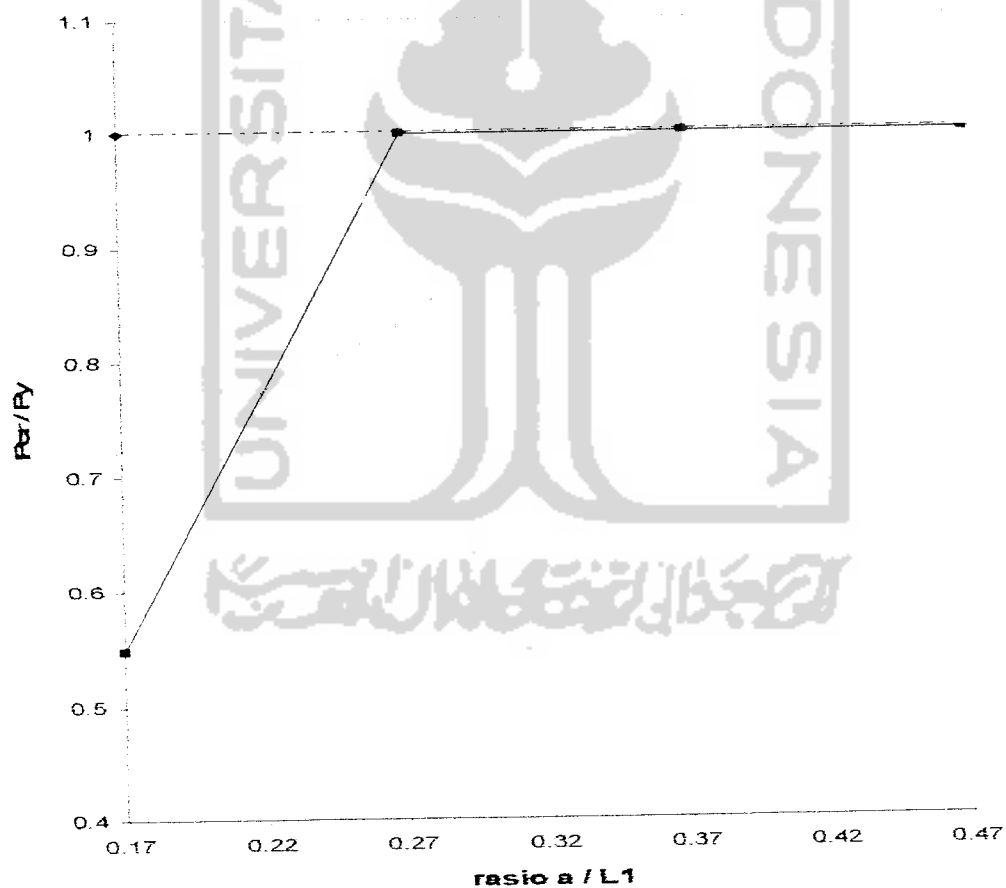
Gambar 5.1 Grafik perbandingan beban kritis versus rasio a/L_1 hasil pengujian dengan beban kritis teoritis.
