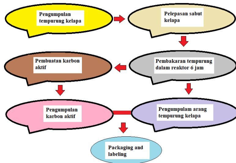
Gambar 2. Bagan alir cara kerja
