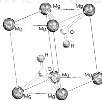
Gambar 3.2 Struktur senyawa brucite
