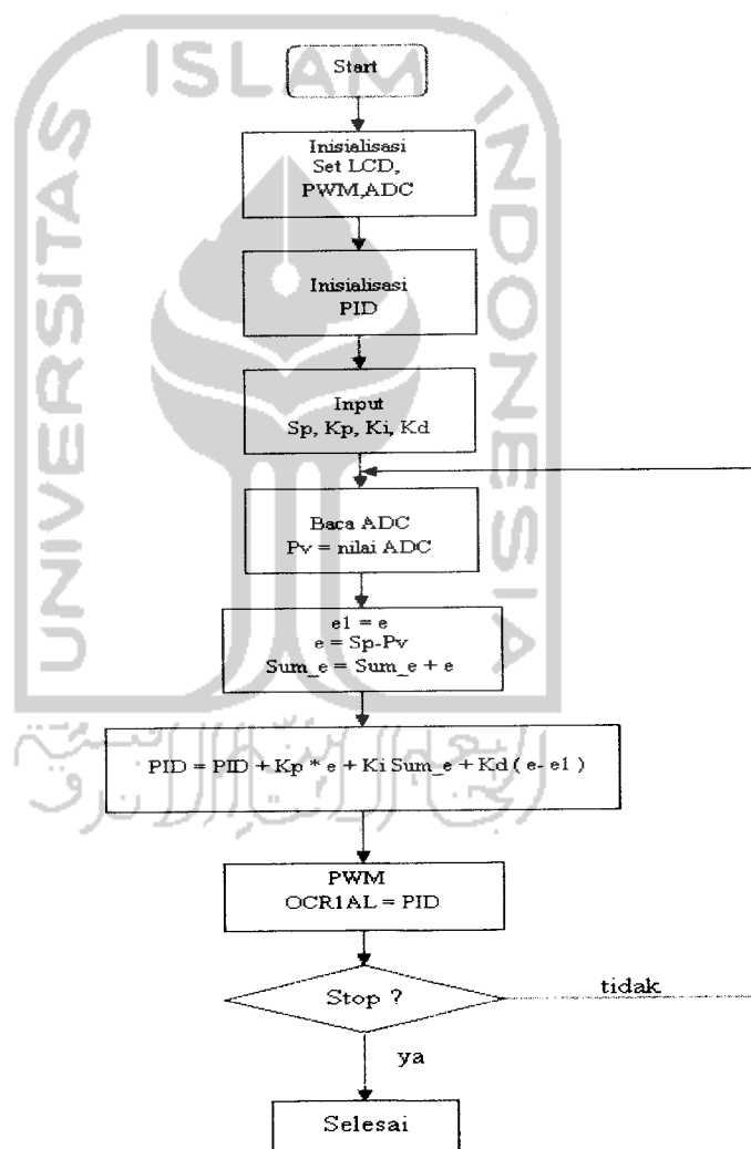
Gambar 3.8. Diagram alir maglev dengan kendali PID
