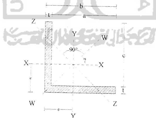
Gambar L.1.2 Momen Inersia Profil Siku
