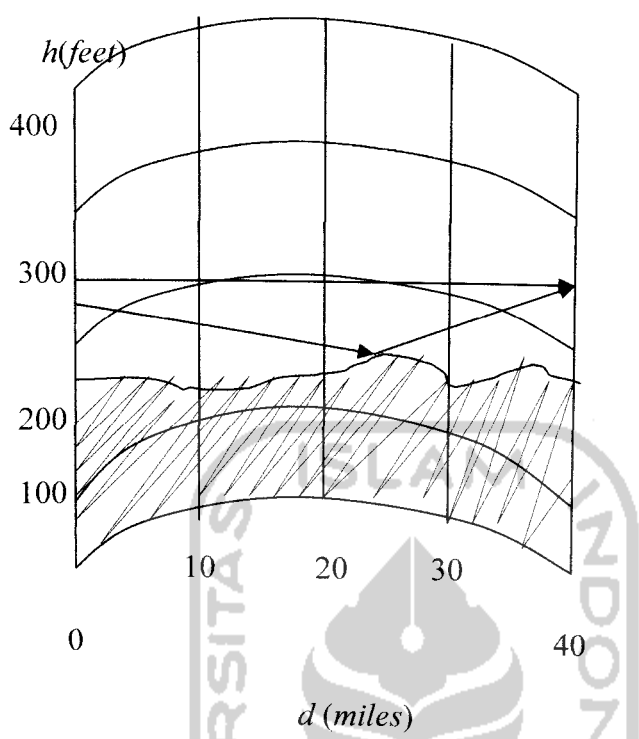
Gambar 3.12. Peta Kountur ( tinggi rendah ) untuk perencanaan jalur
