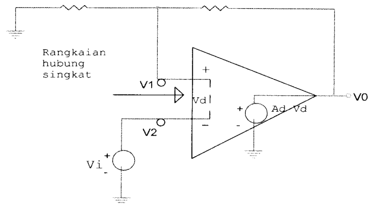
Gambar 2.10 Rangkaian ekivalen
