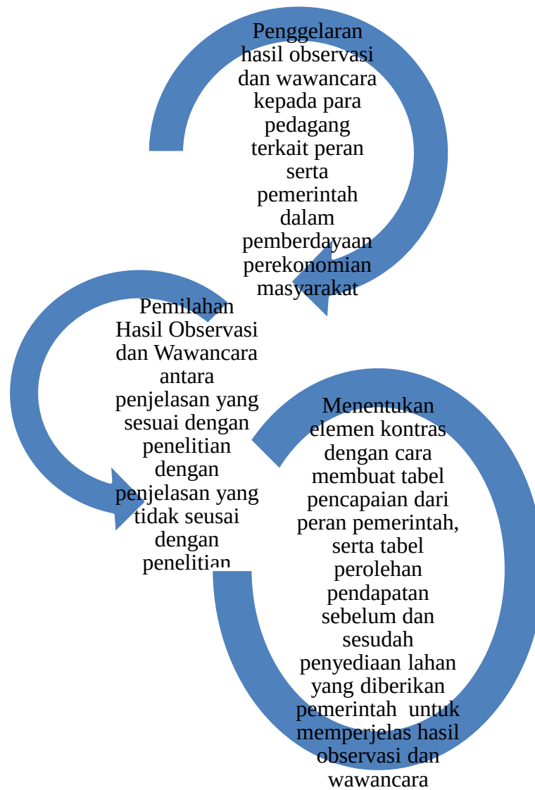
Gambar 3.1 Skema Teknik Analisis Komponensial
