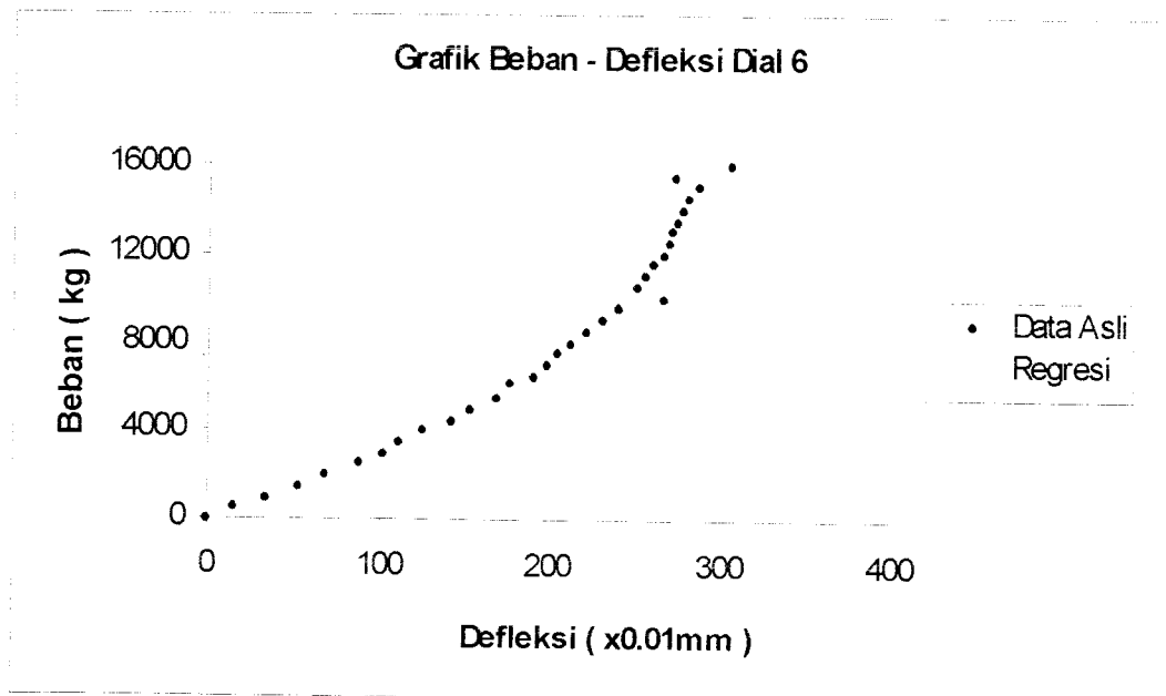
Gambar 5.17 Grafik Beban – Defleksi Dial 6 Benda Uji 1,0m / B / 1
