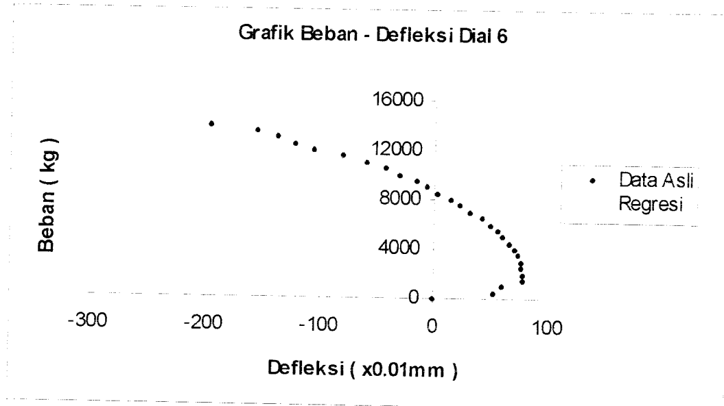
Gambar 5.11 Grafik Beban – Defleksi Dial 6 Benda Uji 1,0m / A / 1
