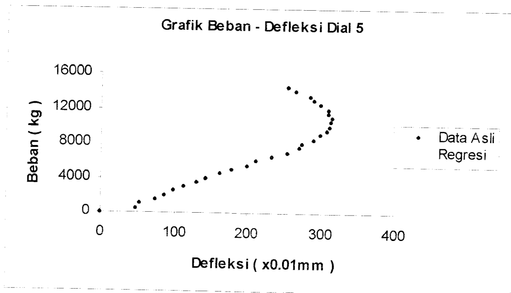
Gambar 5.10 Grafik Beban – Defleksi Dial 5 Benda Uji 1,0m / A / 1
