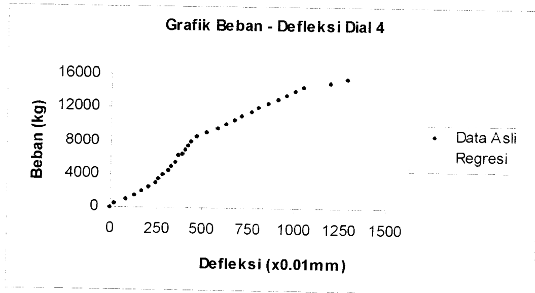
Gambar 5.15 Grafik Beban – Defleksi Dial 4 Benda Uji 1,0m / B / 1
