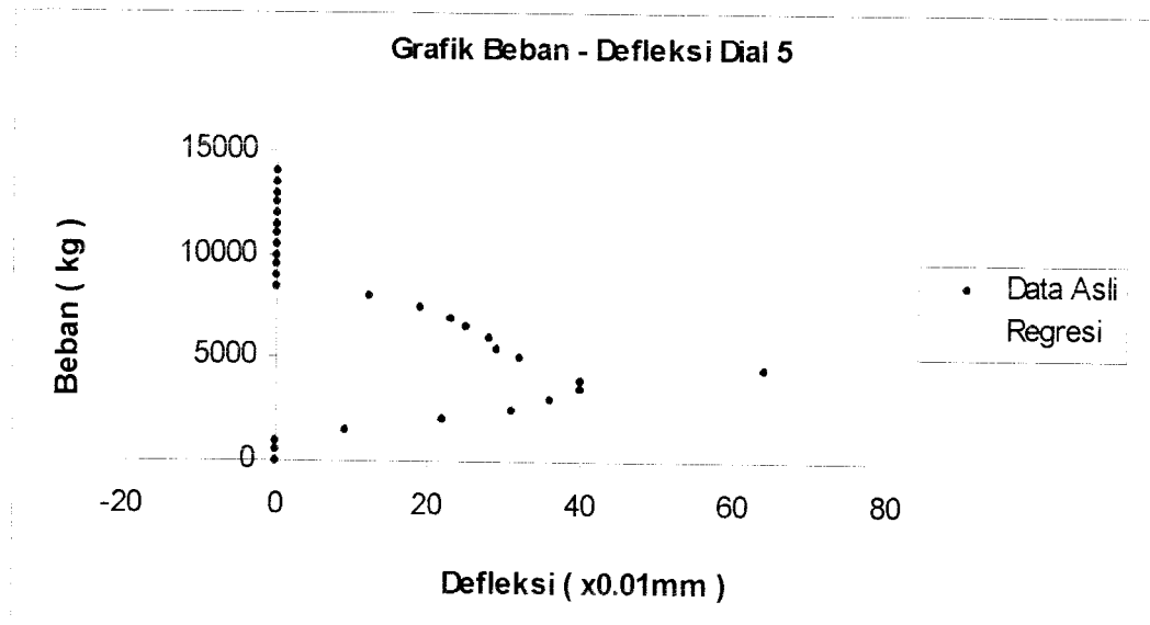
Gambar 5.28 Grafik Beban – Defleksi Dial 5 Benda Uji 1,3m / A / 2
