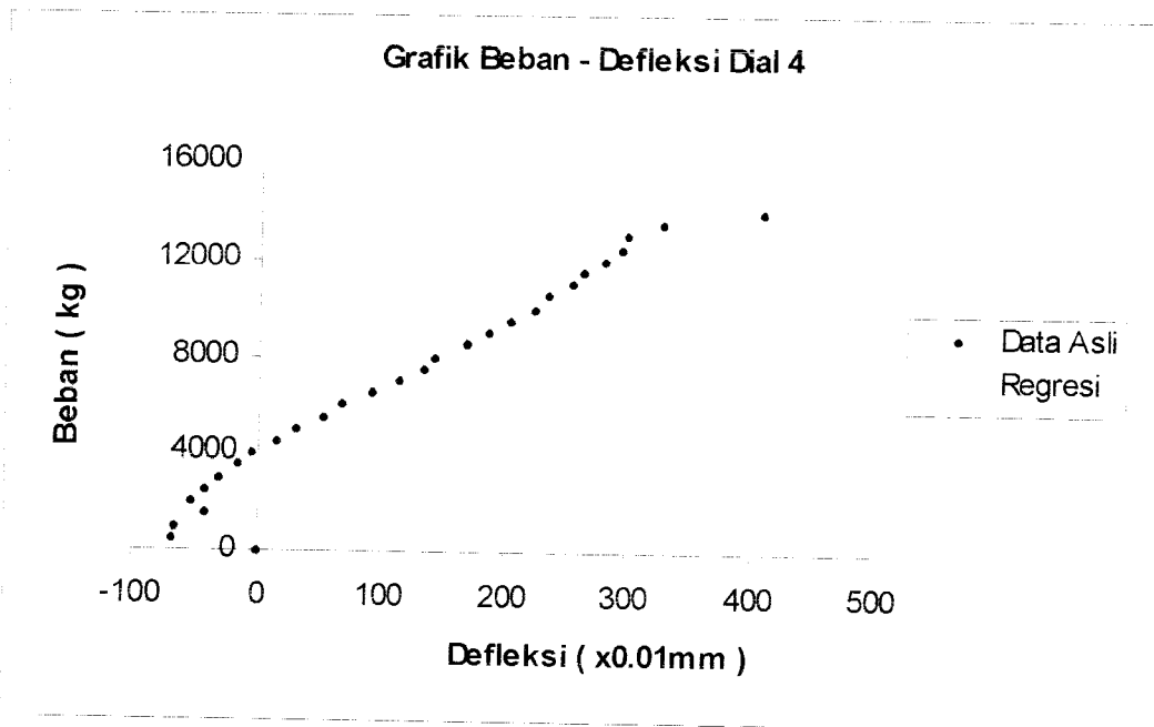
Gambar 5.9 Grafik Beban – Defleksi Dial 4 Benda Uji 1,0m / A / 1
