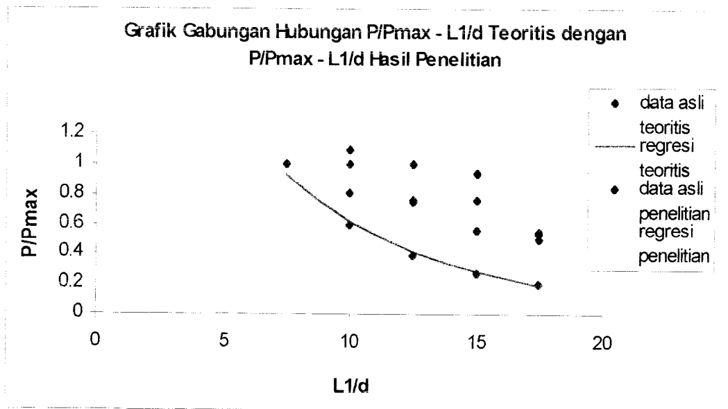
Gambar 6.20 Grafik Gabungan Hubungan P/P_{\max} - L_1/d Teoritis dengan P/P_{\max} - L_1/d Hasil Penelitian
