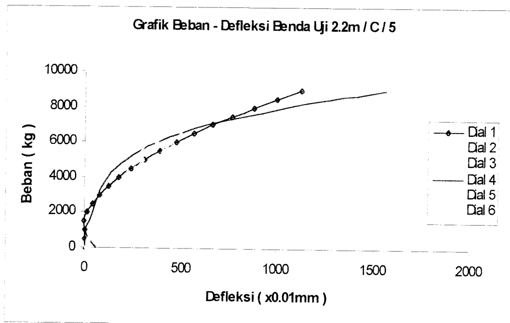
Gambar 6.15 Grafik Gabungan Beban – Defleksi Benda Uji 2,2m / C / 5
