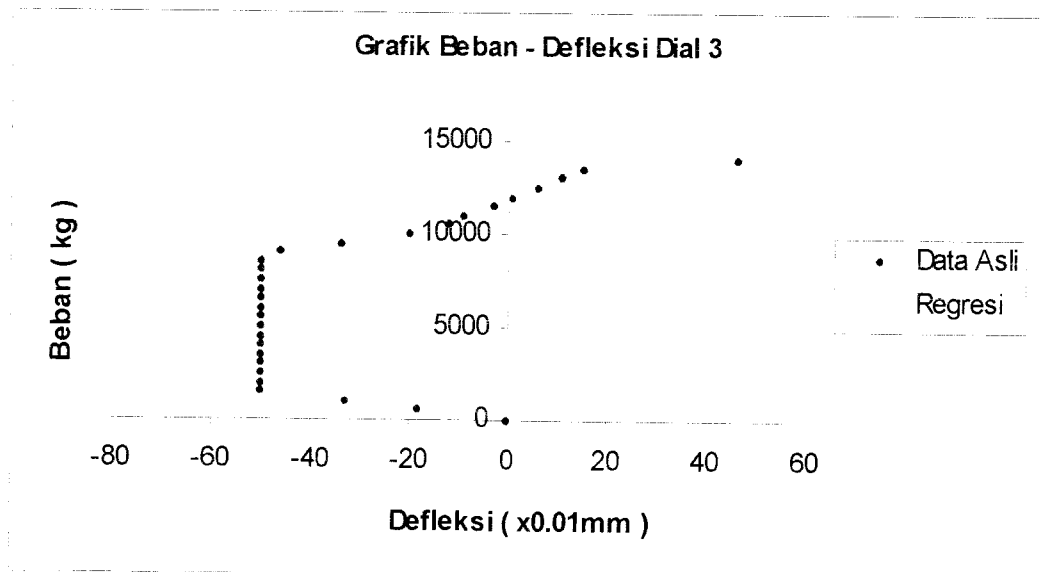
Gambar 5.26 Grafik Beban – Defleksi Dial 3 Benda Uji 1,3m / A / 2
