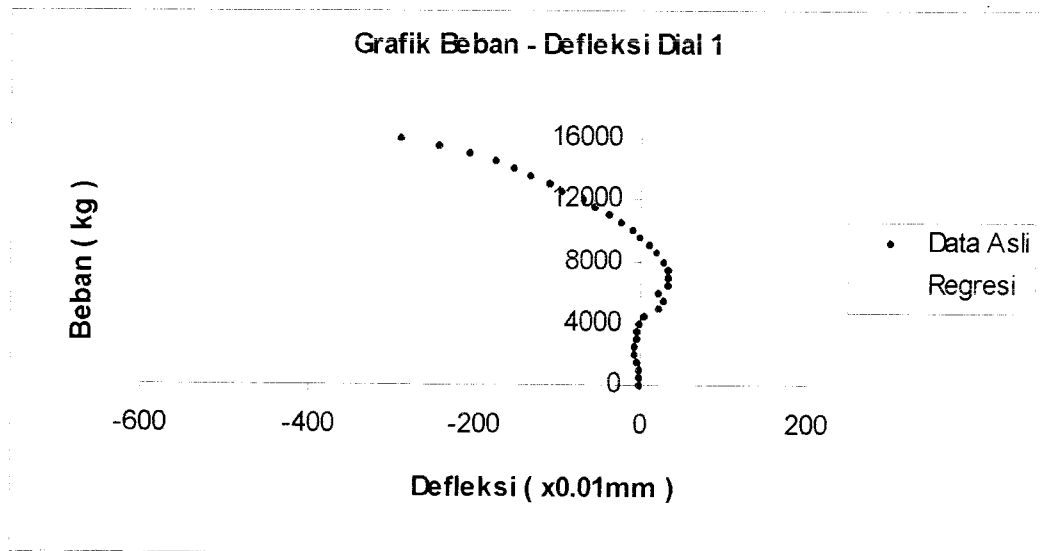
Gambar 5.35 Grafik Beban – Defleksi Dial 1 Benda Uji 1,3m / C / 2
