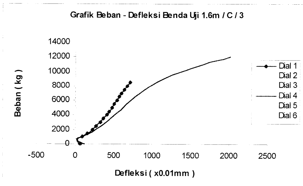
Gambar 6.9 Grafik Gabungan Beban – Defleksi Benda Uji 1,6m / C / 3
