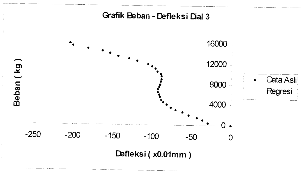
Gambar 5.20 Grafik Beban – Defleksi Dial 3 Benda Uji 1,0m / C / 1
