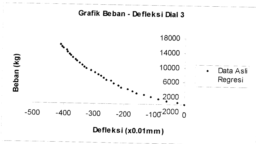
Gambar 5.14 Grafik Beban – Defleksi Dial 3 Benda Uji 1,0m / B / 1
