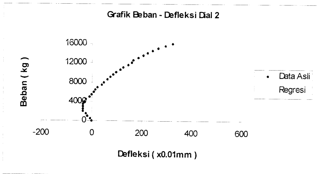
Gambar 5.36 Grafik Beban – Defleksi Dial 2 Benda Uji 1,3m / C / 2
