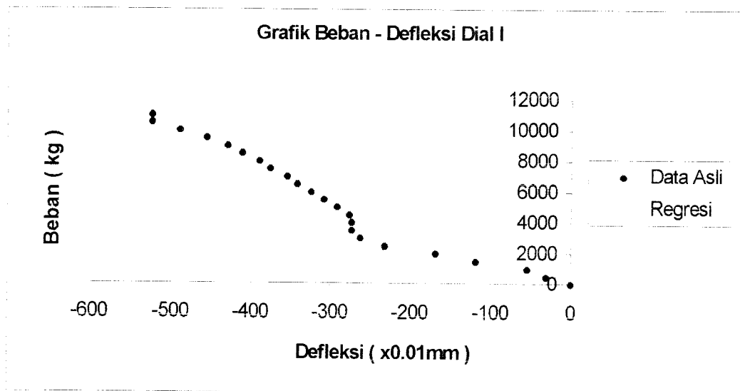
Gambar 5.30 Grafik Beban – Defleksi Dial I Benda Uji 1,3m / B / 2
