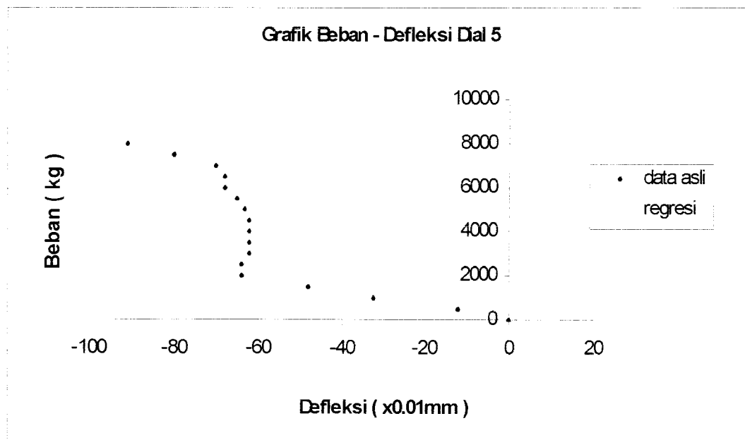
Gambar 5.75 Grafik Beban – Defleksi Dial 5 Benda Uji 1,9m / C / 4
