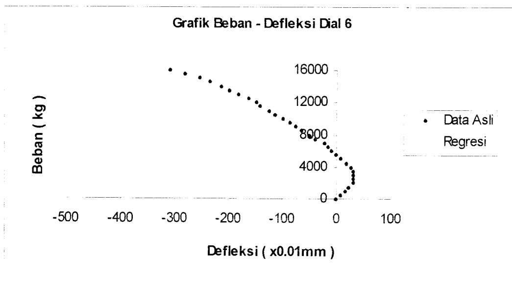
Gambar 5.40 Grafik Beban – Defleksi Dial 6 Benda Uji 1,3m / C / 2
