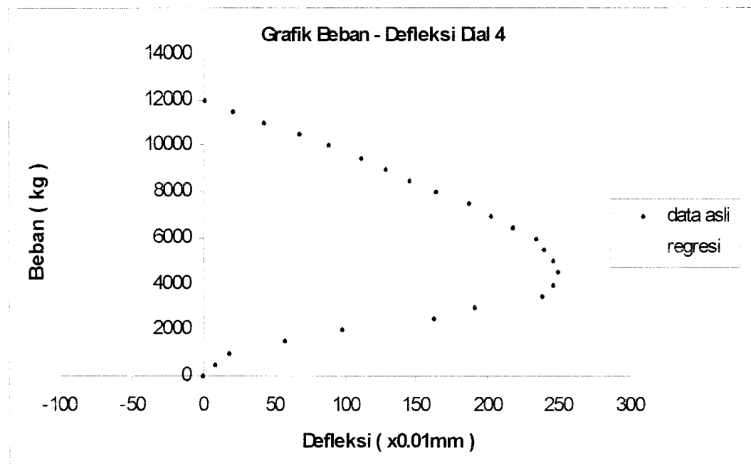
Gambar 5.50 Grafik Beban – Defleksi Dial 4 Benda Uji 1,6m / B / 3
