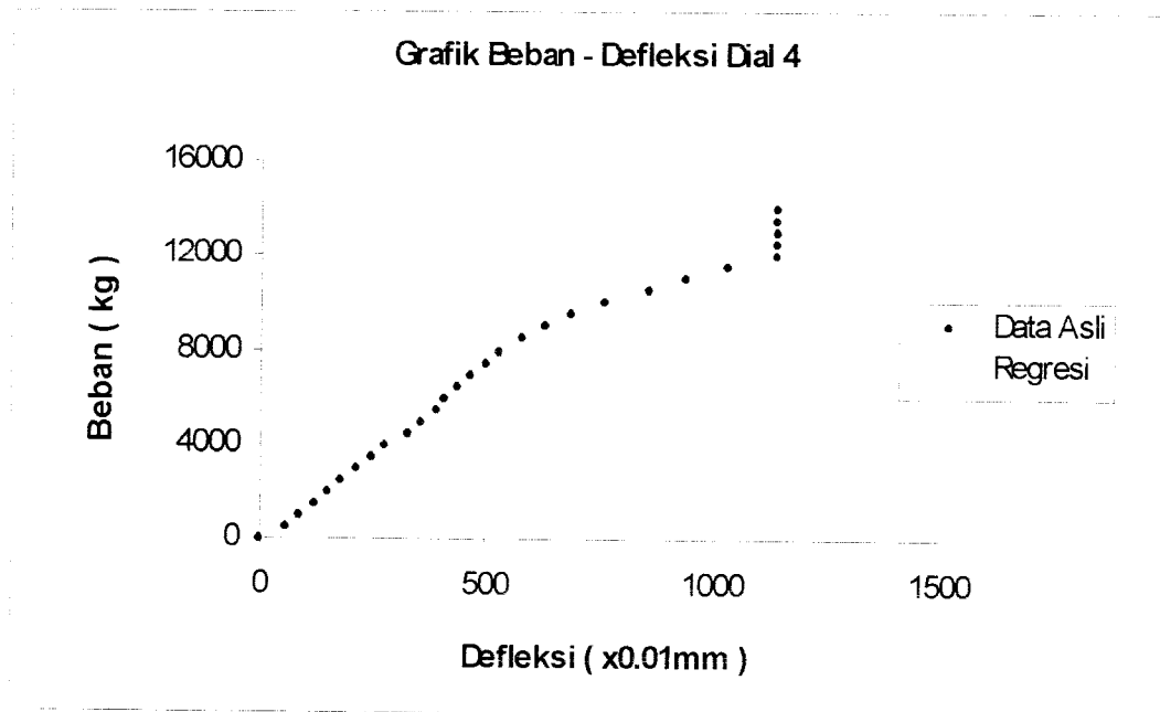
Gambar 5.27 Grafik Beban – Defleksi Dial 4 Benda Uji 1,3m / A / 2
