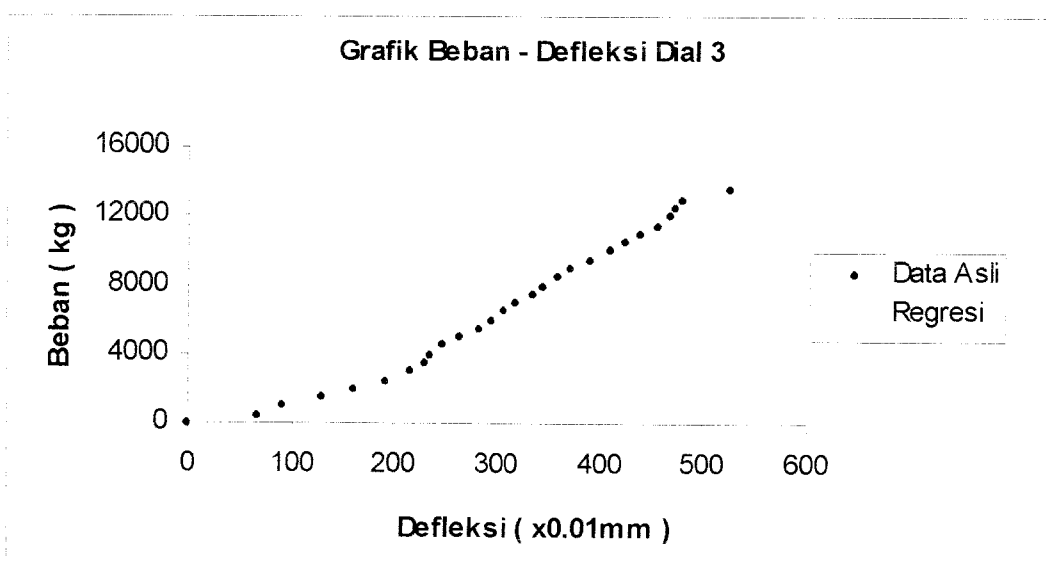
Gambar 5.32 Grafik Beban – Defleksi Dial 3 Benda Uji 1,3m / B / 2
