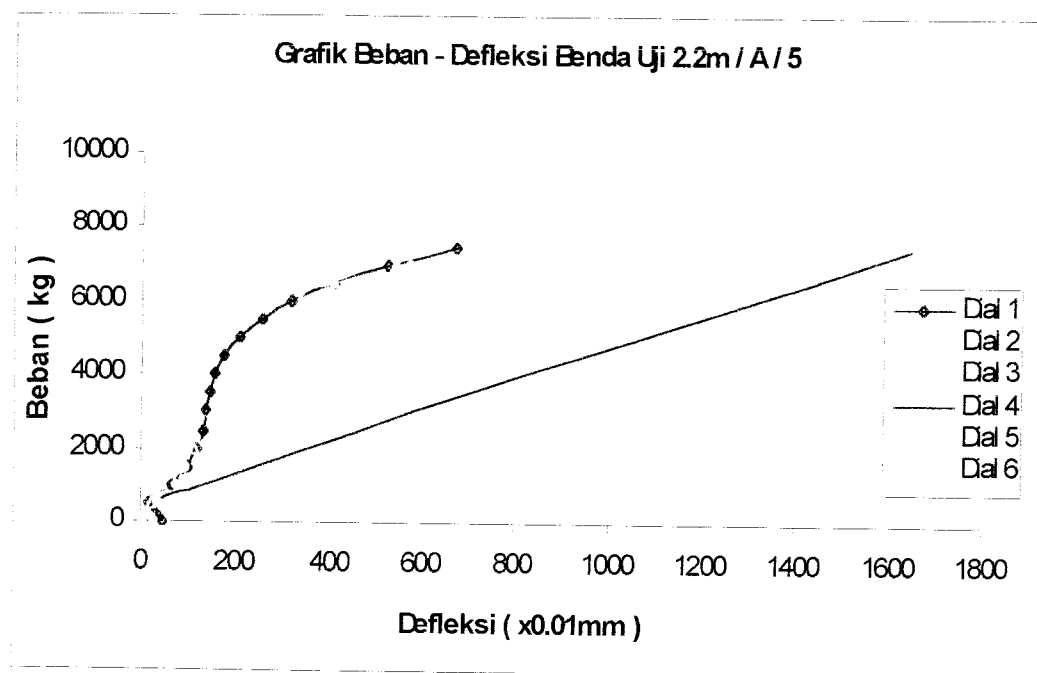
Gambar 6.13 Grafik Gabungan Beban – Defleksi Benda Uji 2,2m / A / 5
