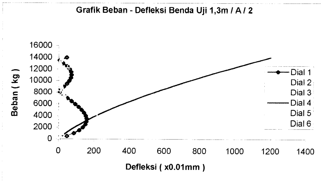
Gambar 6.4 Grafik Gabungan Beban – Defleksi Benda Uji 1,3m / A / 2
