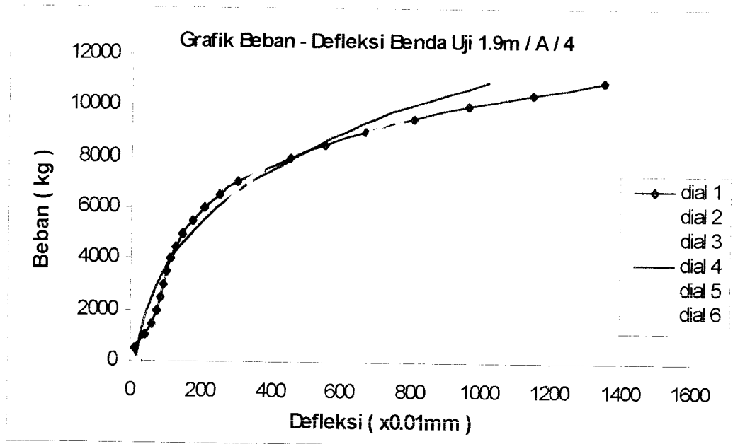
Gambar 6.10 Grafik Gabungan Beban – Defleksi Benda Uji 1,9m / A / 4
