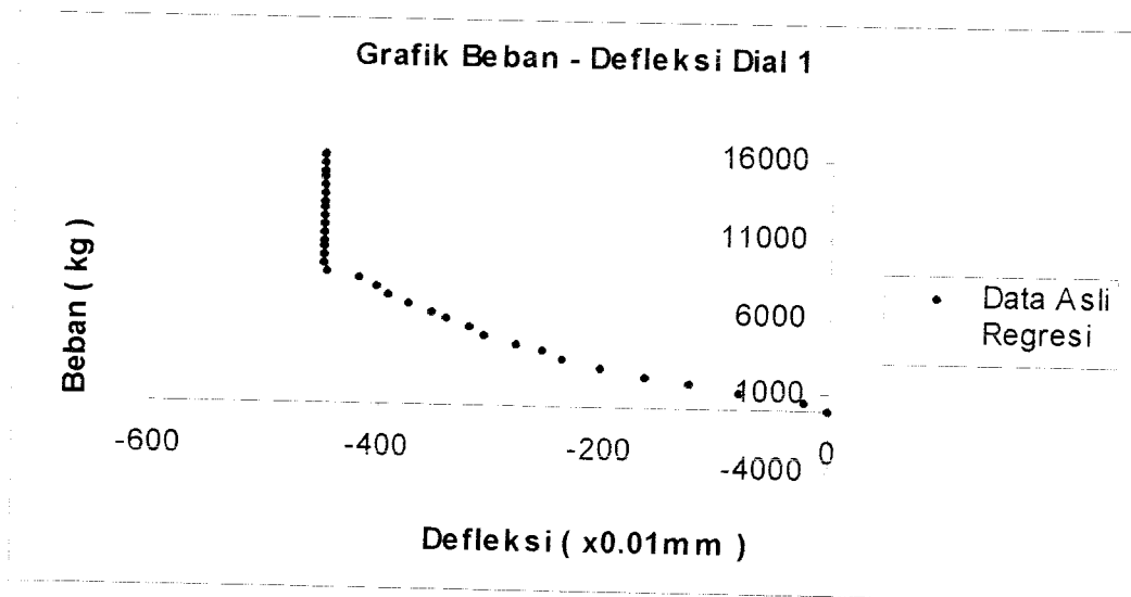
Gambar 5.12 Grafik Beban – Defleksi Dial 1 Benda Uji 1,0m / B / 1
