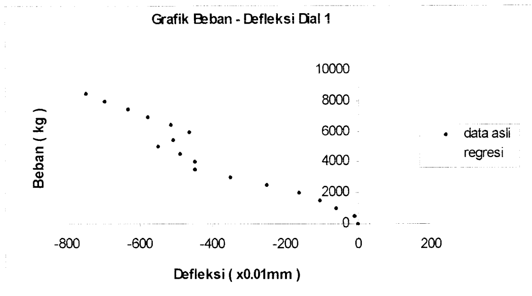
Gambar 5.53 Grafik Beban – Defleksi Dial 1 Benda Uji 1,6m / C / 3
