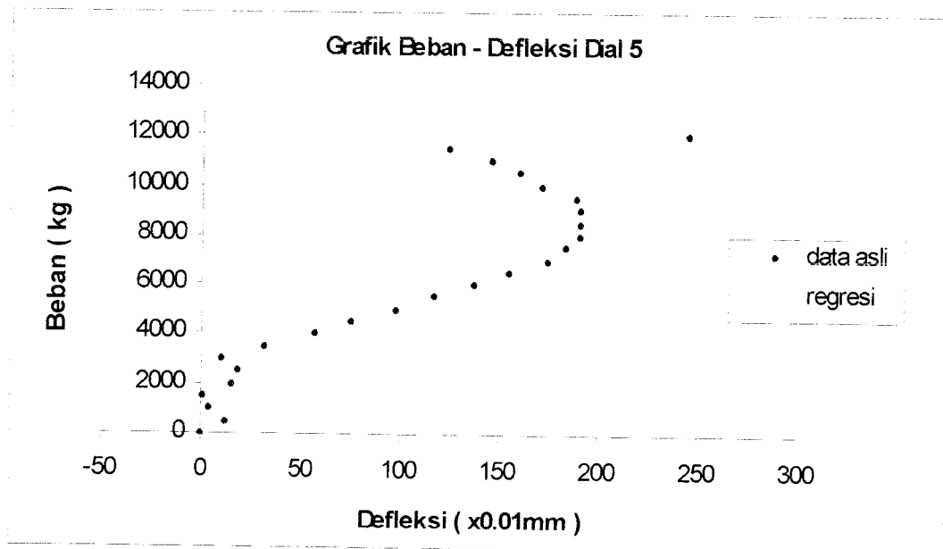
Gambar 5.57 Grafik Beban – Defleksi Dial 5 Benda Uji 1,6m / C / 3
