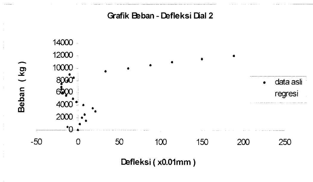
Gambar 5.54 Grafik Beban – Defleksi Dial 2 Benda Uji 1,6m / C / 3
