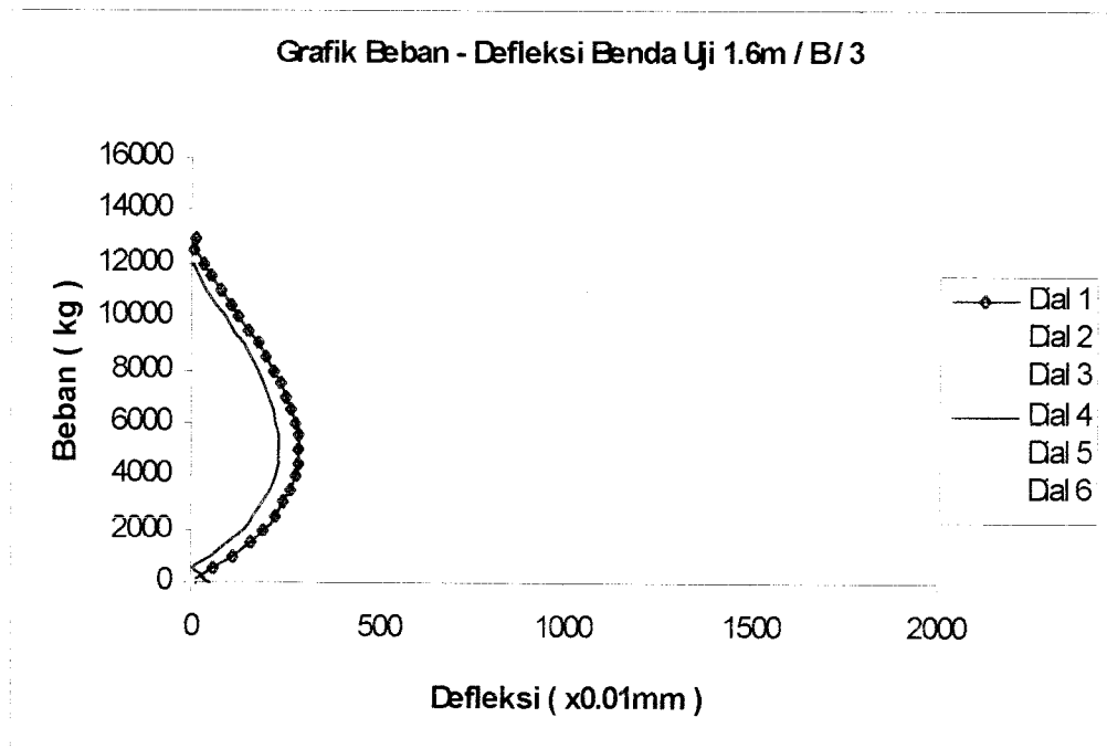
Gambar 6.8 Grafik Gabungan Beban – Defleksi Benda Uji 1,6m / B / 3
