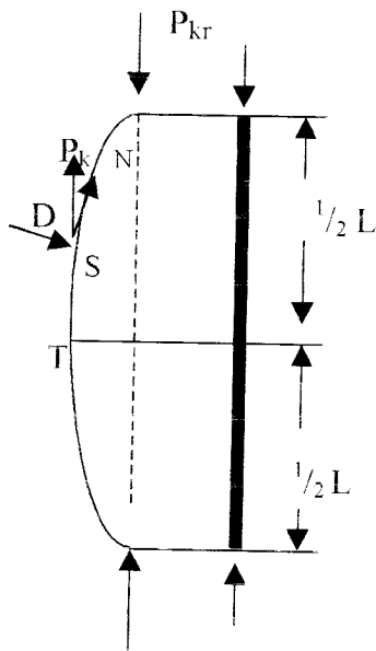
Gambar 3.3 Lentur pada Batang akibat Beban Desak
