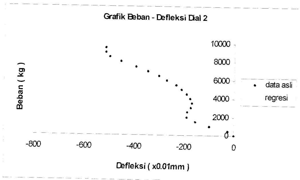
Gambar 5.60 Grafik Beban – Defleksi Dial 2 Benda Uji 1,9m / A / 4
