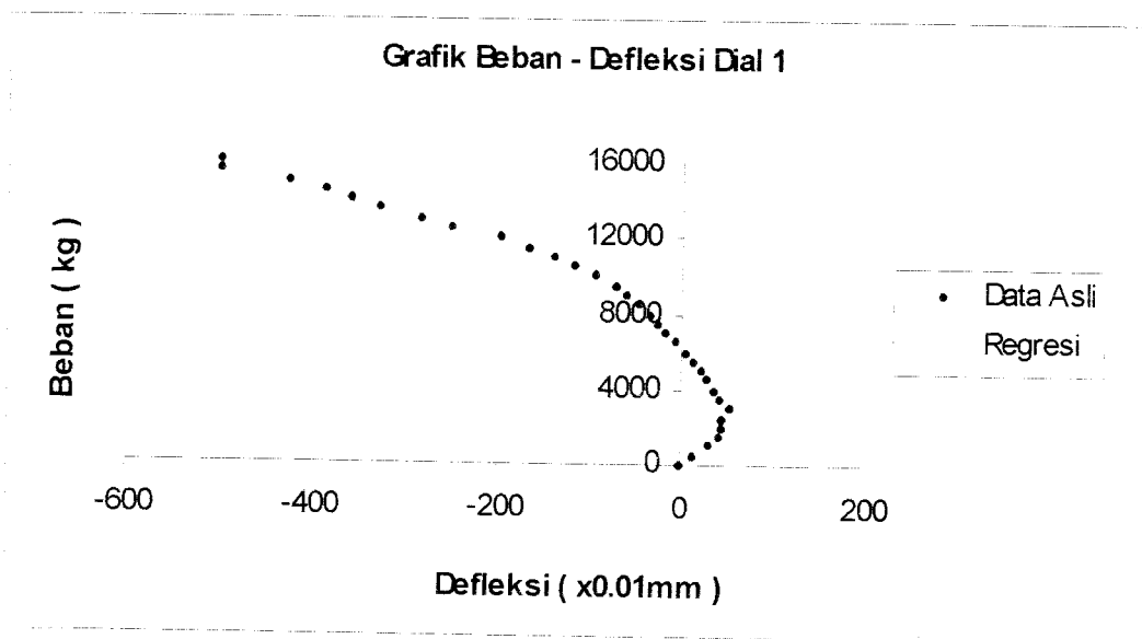
Gambar 5.18 Grafik Beban – Defleksi Dial 1 Benda Uji 1,0m / C / 1
