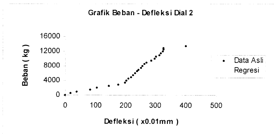
Gambar 5.31 Grafik Beban – Defleksi Dial 2 Benda Uji 1,3m / B / 2
