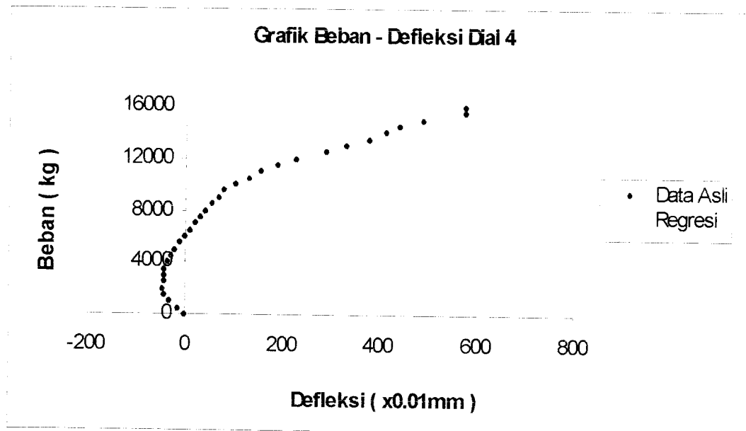
Gambar 5.21 Grafik Beban – Defleksi Dial 4 Benda Uji 1,0m / C / 1
