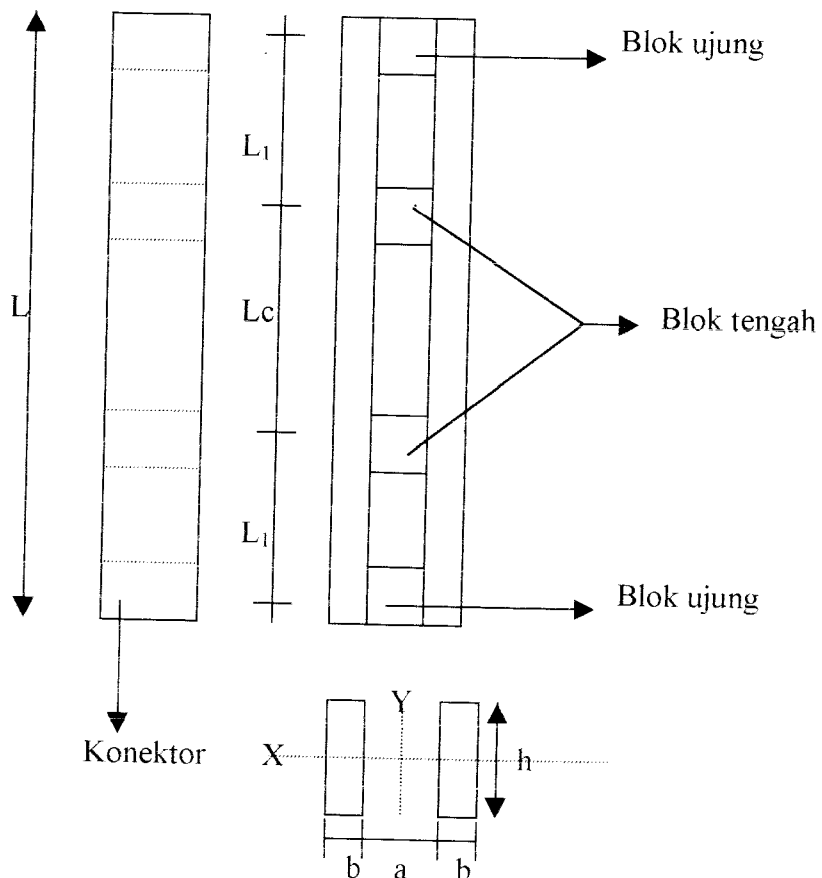
Gambar 2.1 Skema Batang Ganda dengan Klos
