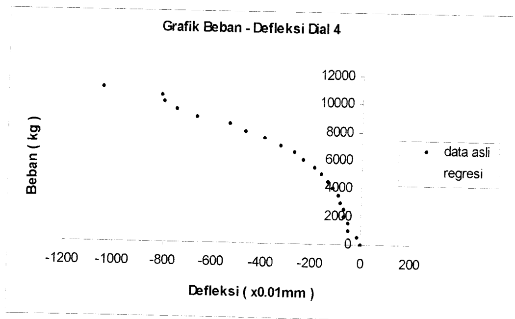
Gambar 5.62 Grafik Beban – Defleksi Dial 4 Benda Uji 1,9m / A / 4
