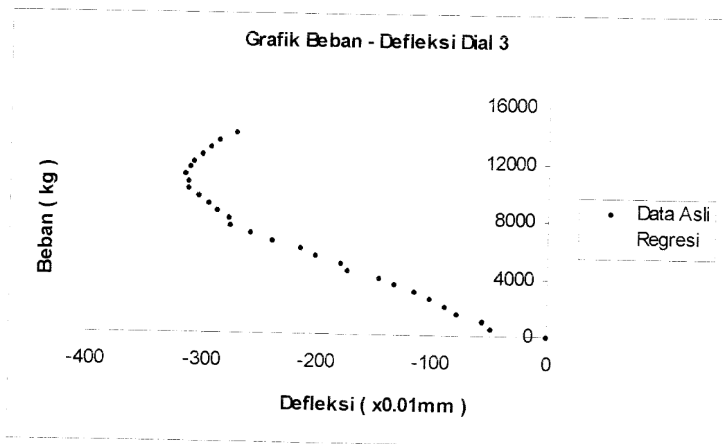
Gambar 5.8 Grafik Beban – Defleksi Dial 3 Benda Uji 1,0m / A / 1
