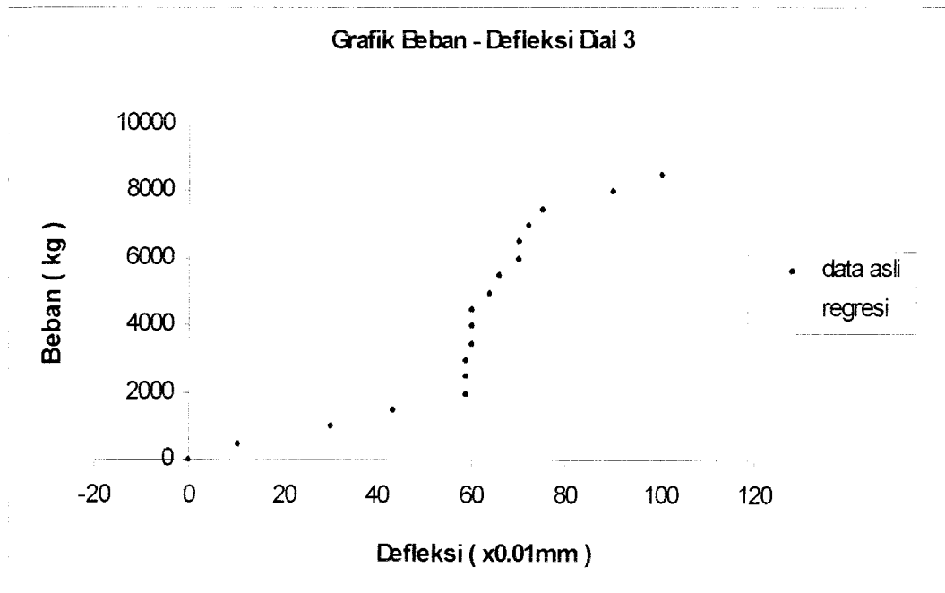
Gambar 5.73 Grafik Beban – Defleksi Dial 3 Benda Uji 1,9m / C / 4
