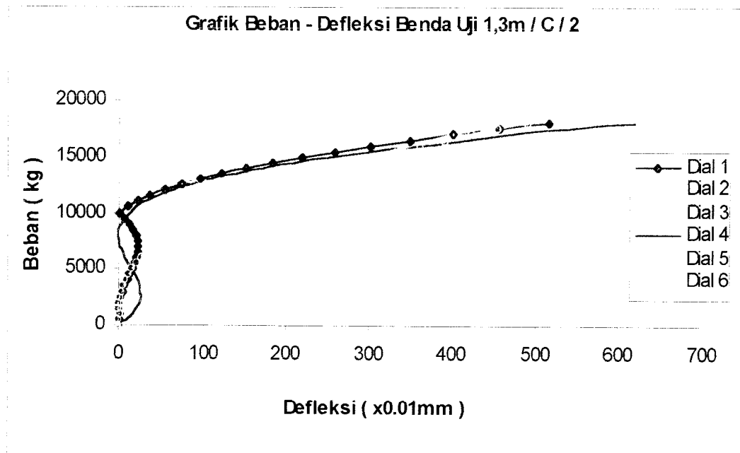
Gambar 6.6 Grafik Gabungan Beban – Defleksi Benda Uji 1,3m / C / 2
