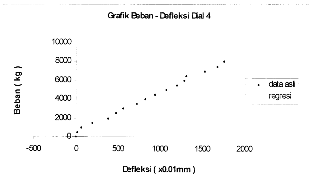
Gambar 5.80 Grafik Beban – Defleksi Dial 4 Benda Uji 2,2m / A / 5
