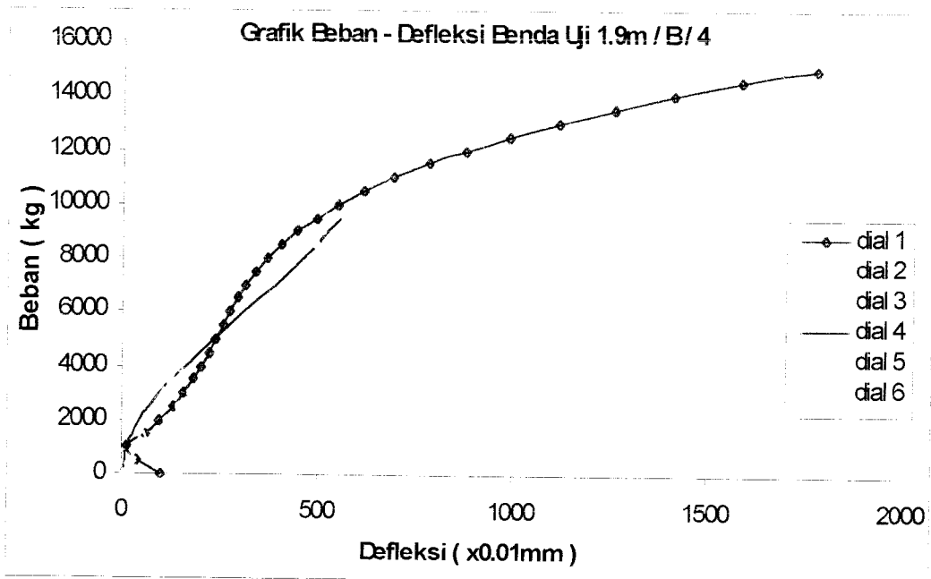
Gambar 6.11 Grafik Gabungan Beban – Defleksi Benda Uji 1,9m / B / 4
