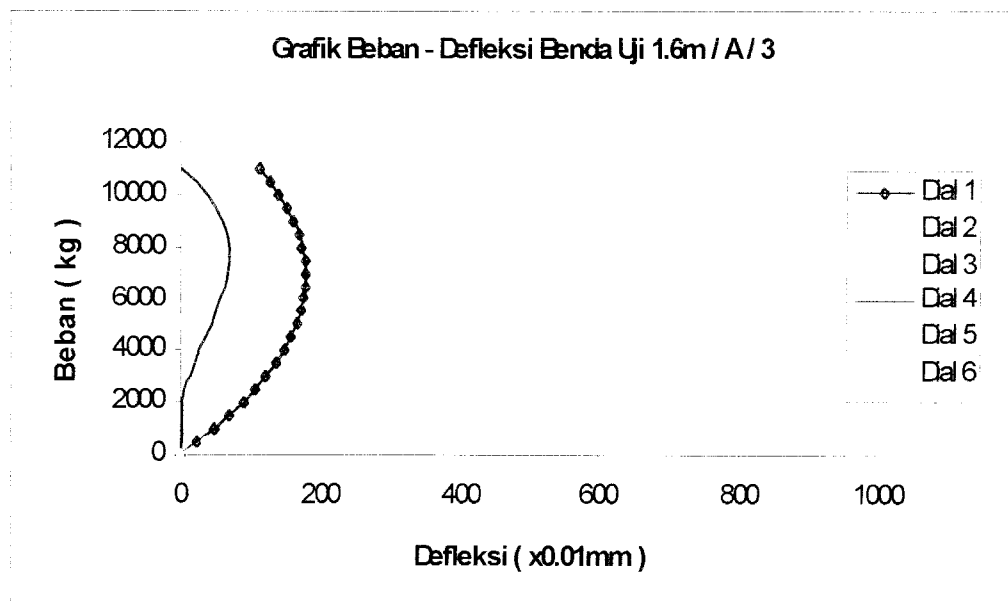
Gambar 6.7 Grafik Gabungan Beban – Defleksi Benda Uji 1,6m / A / 3
