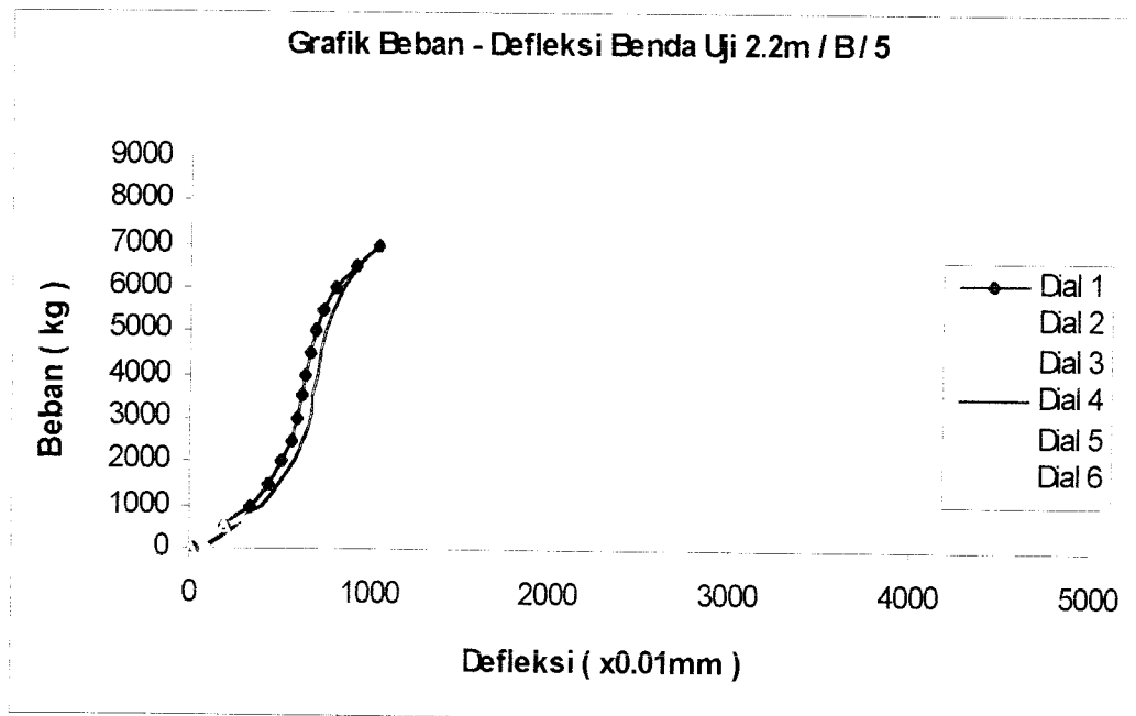
Gambar 6.14 Grafik Gabungan Beban – Defleksi Benda Uji 2,2m / B / 5
