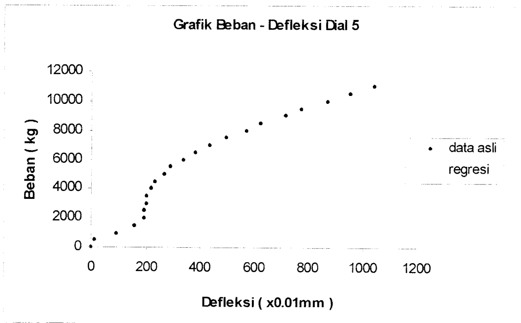
Gambar 5.63 Grafik Beban – Defleksi Dial 5 Benda Uji 1,9m / A / 4
