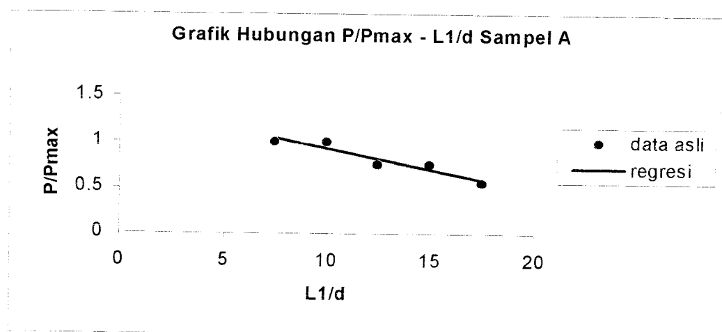
Gambar 6.16 Grafik Hubungan P/P_{max} - L_1/d Sampel A
