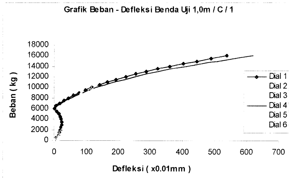
Gambar 6.3 Grafik Gabungan Beban – Defleksi Benda Uji 1,0m / C / 1
