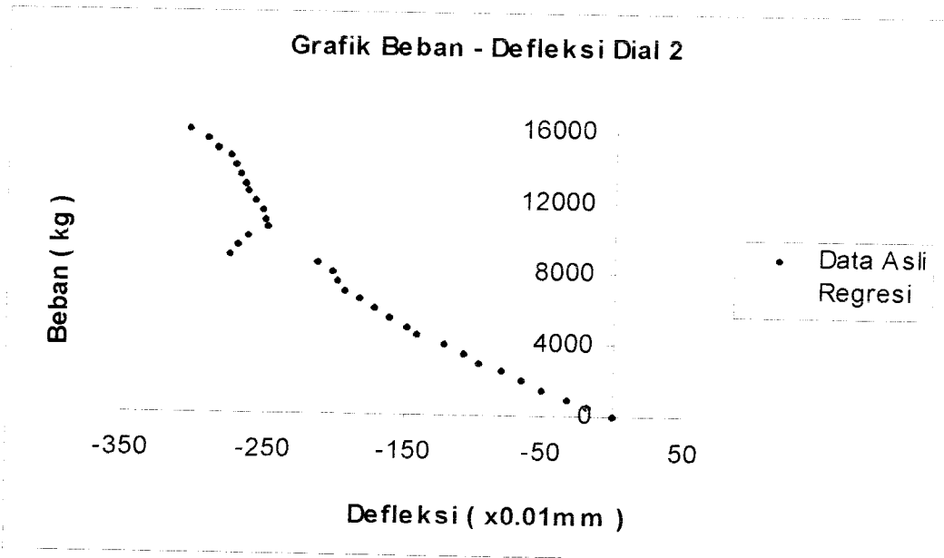
Gambar 5.13 Grafik Beban – Defleksi Dial 2 Benda Uji 1,0m / B / 1
