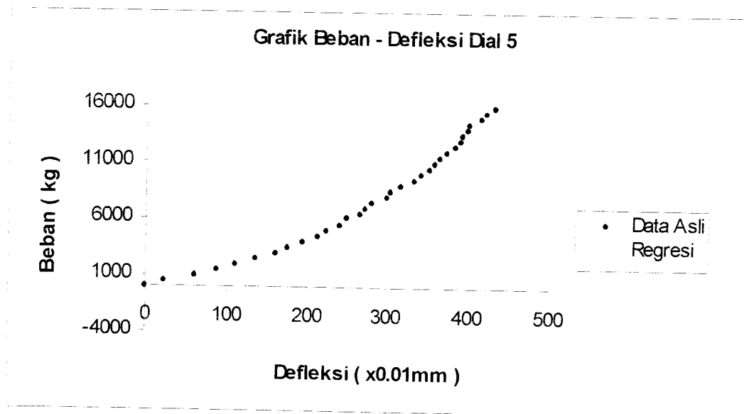
Gambar 5.16 Grafik Beban – Defleksi Dial 5 Benda Uji 1,0m / B / 1
