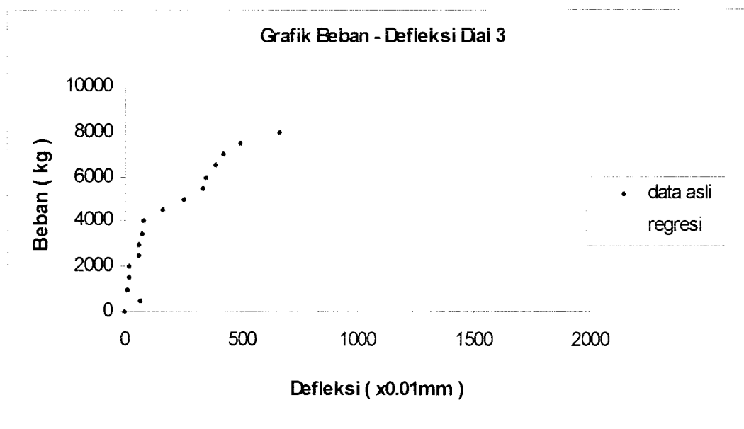
Gambar 5.79 Grafik Beban – Defleksi Dial 3 Benda Uji 2,2m / A / 5
