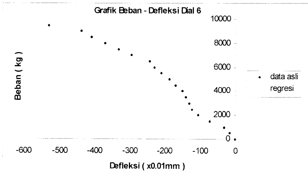
Gambar 5.46 Grafik Beban – Defleksi Dial 6 Benda Uji 1,6m / A / 3
