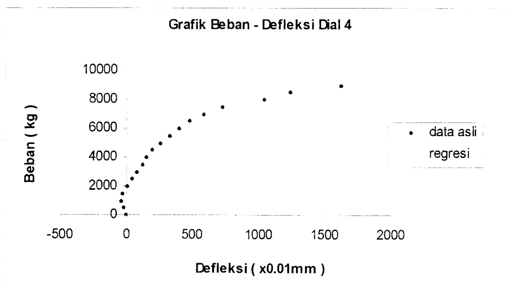
Gambar 5.92 Grafik Beban – Defleksi Dial 4 Benda Uji 2,2m / C / 5
