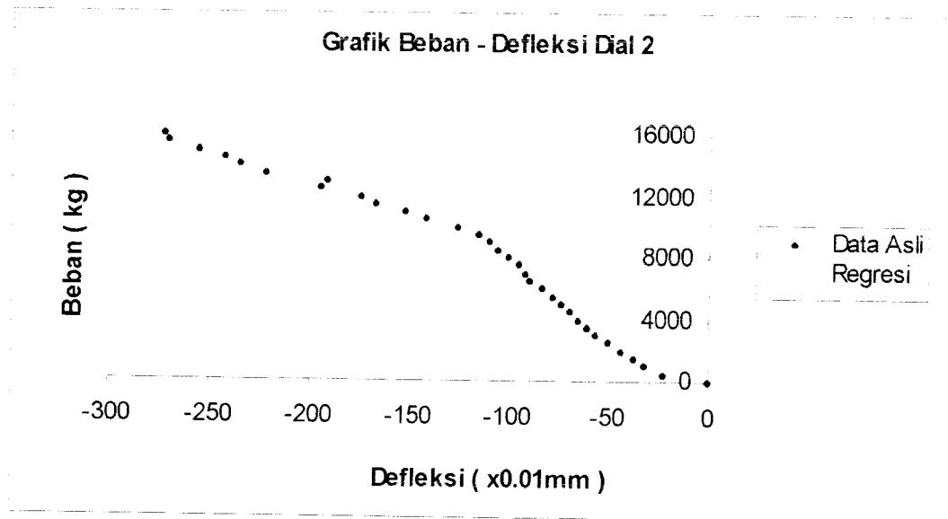
Gambar 5.19 Grafik Beban – Defleksi Dial 2 Benda Uji 1,0m / C / 1
