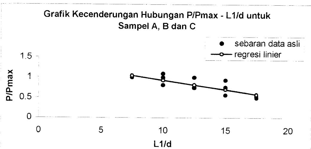
Gambar 6.19 Grafik Kecenderungan P/P_{\max} - L_1/d untuk Tiga Sampel Penelitian
