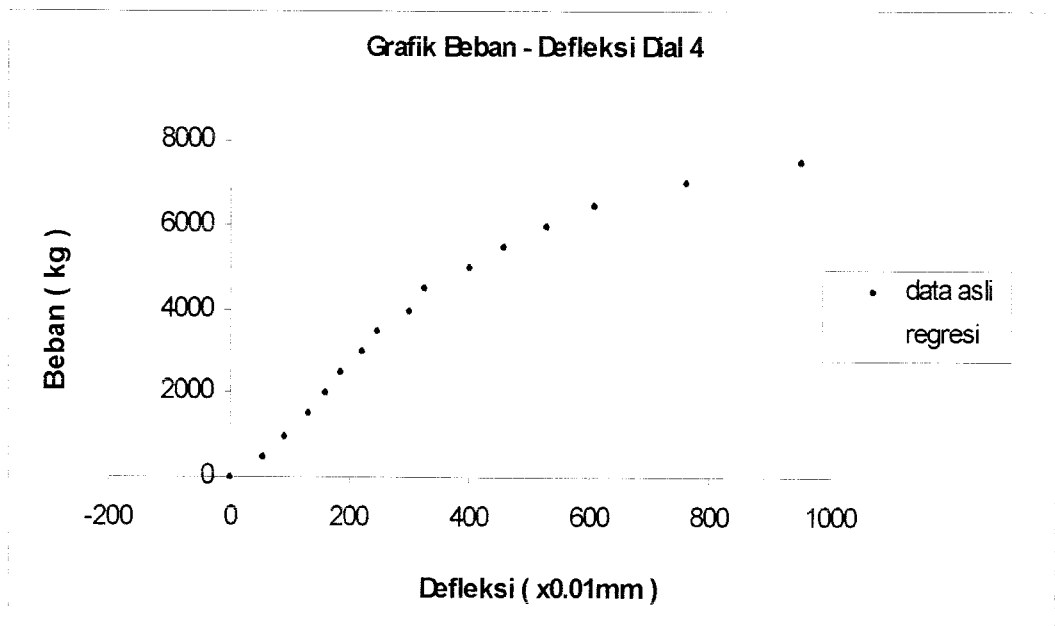
Gambar 5.74 Grafik Beban – Defleksi Dial 4 Benda Uji 1,9m / C / 4
