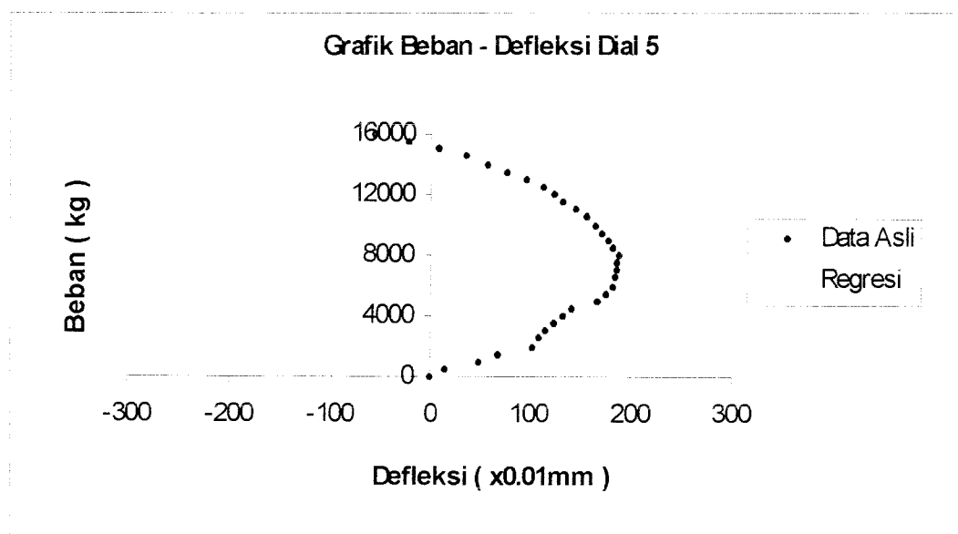
Gambar 5.39 Grafik Beban – Defleksi Dial 5 Benda Uji 1,3m / C / 2
