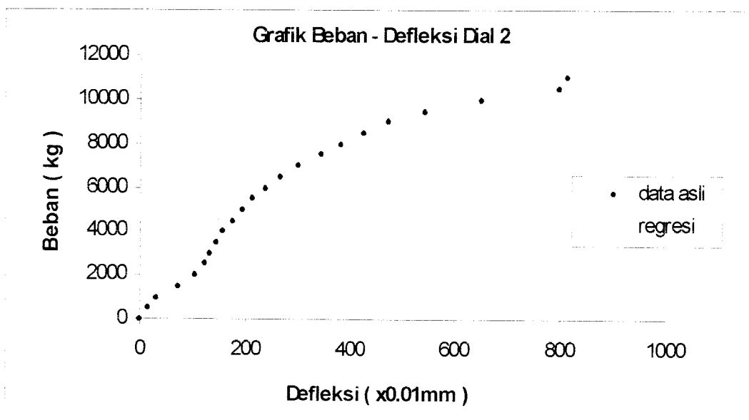
Gambar 5.42 Grafik Beban – Defleksi Dial 2 Benda Uji 1,6m / A / 3
