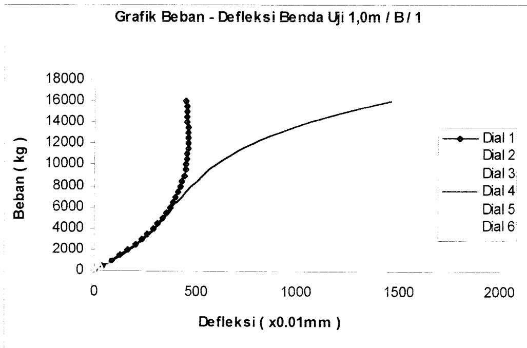
Gambar 6.2 Grafik Gabungan Beban – Defleksi Benda Uji 1,0m / B / 1
