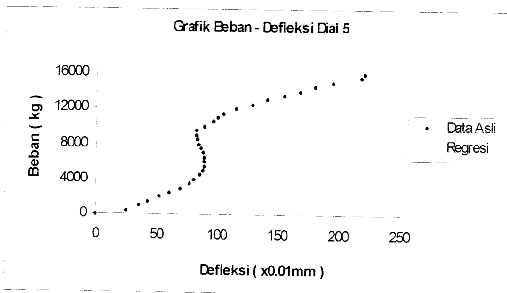
Gambar 5.22 Grafik Beban – Defleksi Dial 5 Benda Uji 1,0m / C / 1
