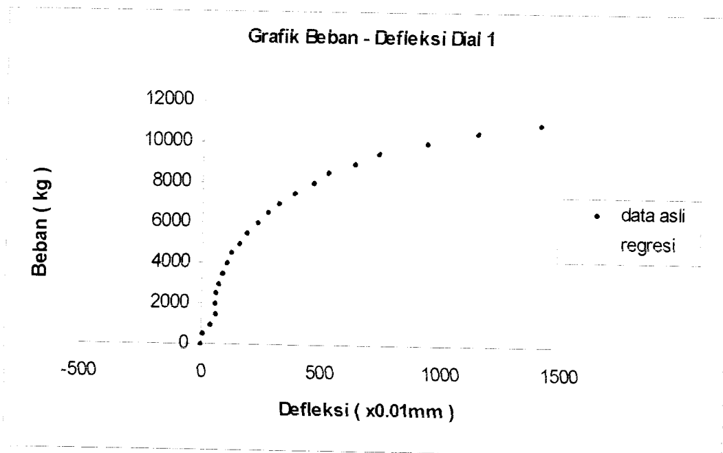
Gambar 5.59 Grafik Beban – Defleksi Dial 1 Benda Uji 1,9m / A / 4
