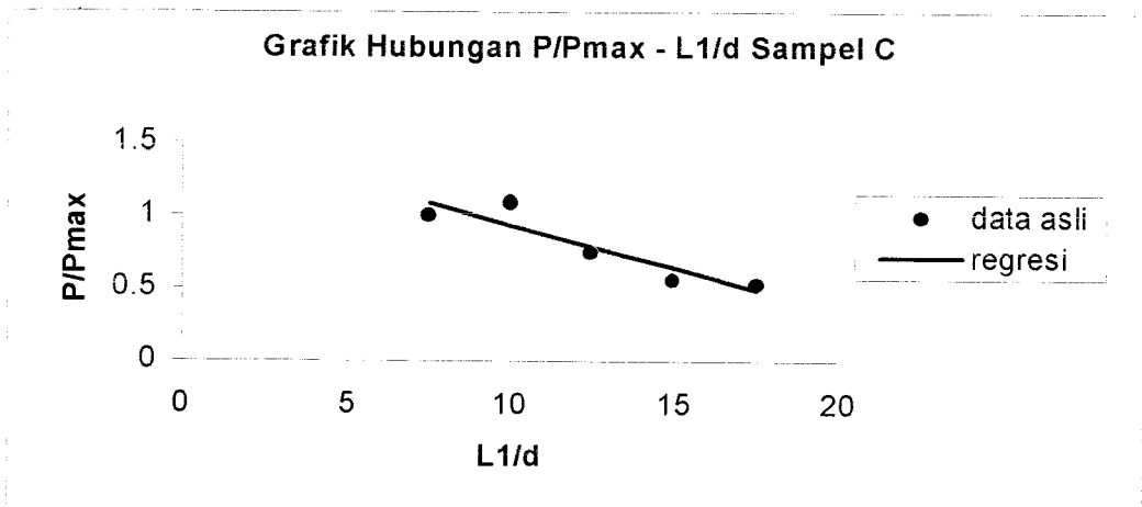
Gambar 6.18 Grafik Hubungan P/P_{\max} - ( L_1/d ) Sampel C
