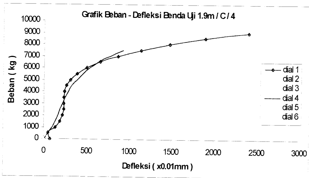
Gambar 6.12 Grafik Gabungan Beban – Defleksi Benda Uji 1,9m / C / 4
