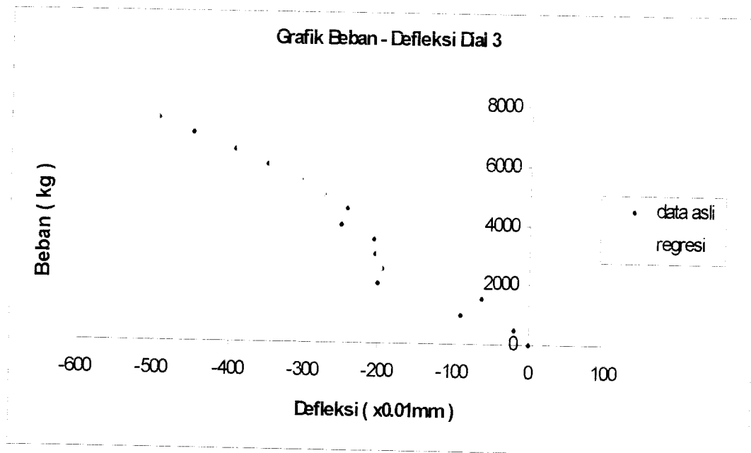
Gambar 5.61 Grafik Beban – Defleksi Dial 3 Benda Uji 1,9m / A / 4
