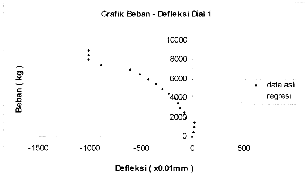
Gambar 5.89 Grafik Beban – Defleksi Dial 1 Benda Uji 2,2m / C / 5
