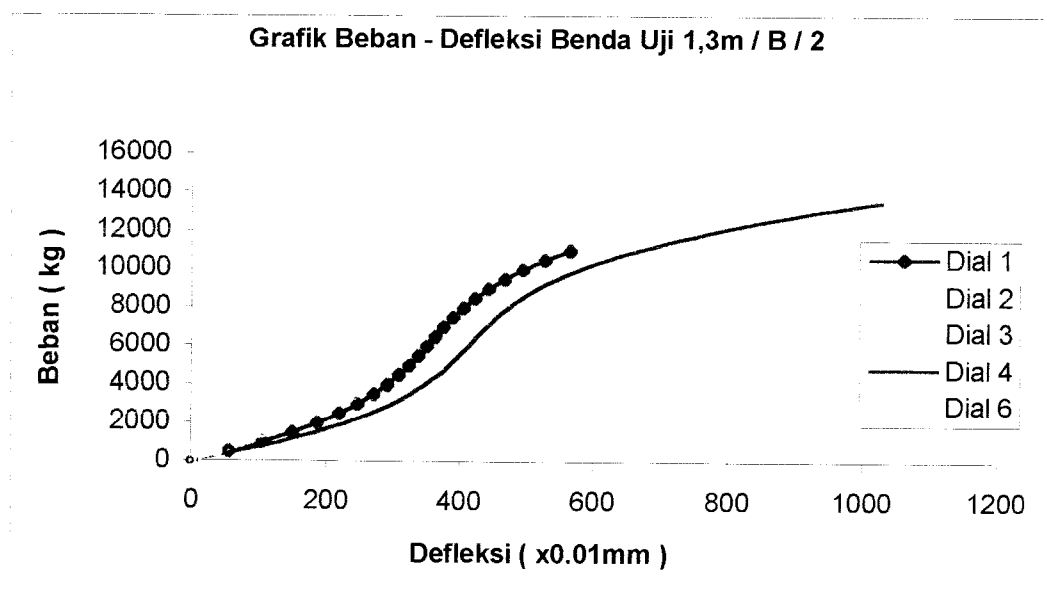
Gambar 6.5 Grafik Gabungan Beban – Defleksi Benda Uji 1,3m / B / 2
