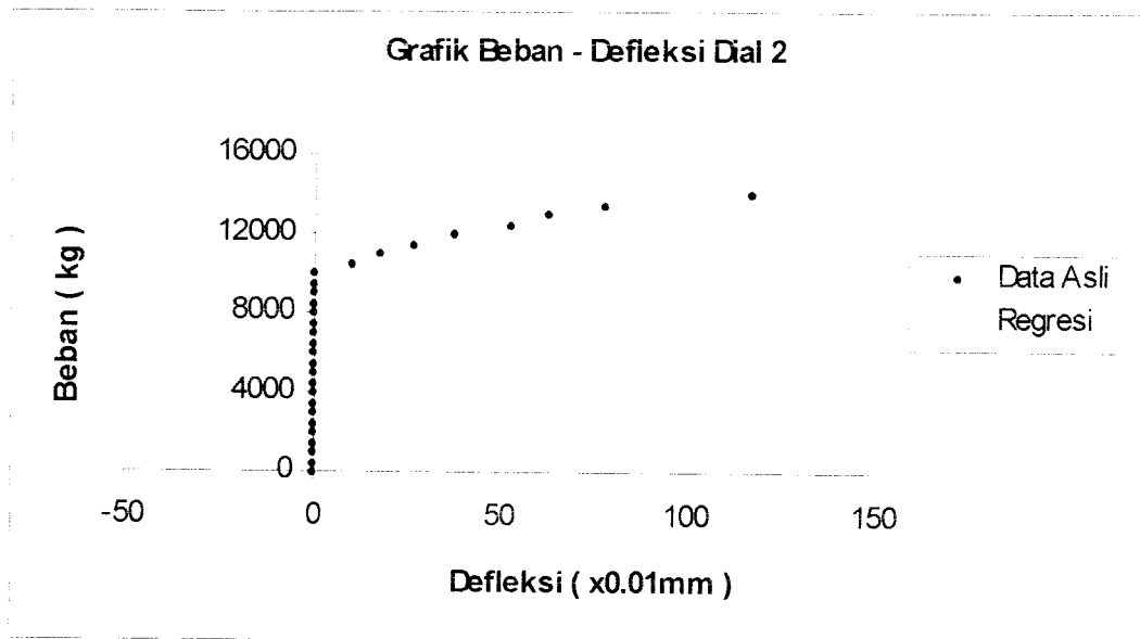
Gambar 5.25 Grafik Beban – Defleksi Dial 2 Benda Uji 1,3m / A / 2
