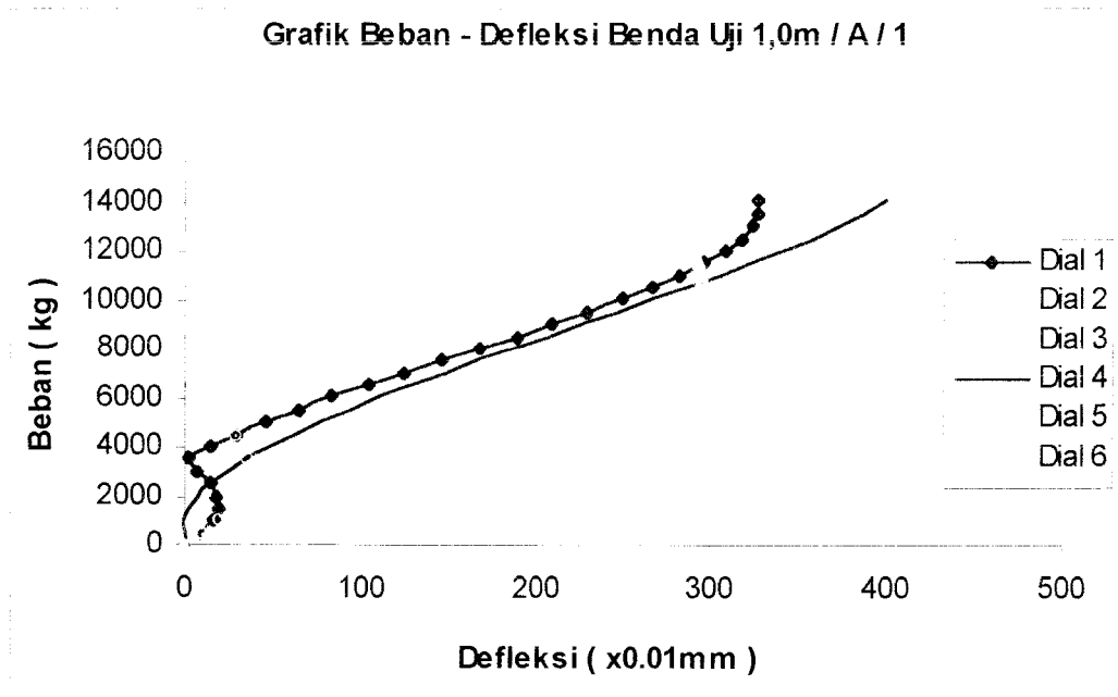
Gambar 6.1 Grafik Gabungan Beban – Defleksi Benda Uji 1,0m / A / 1
