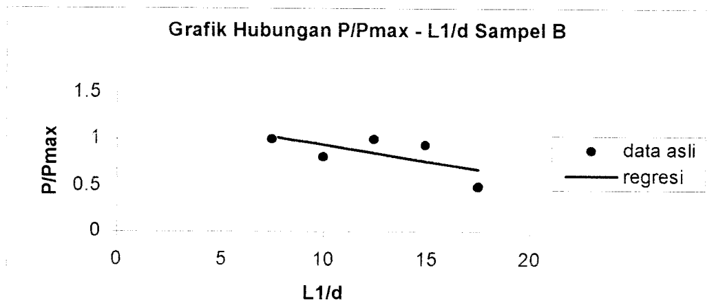
Gambar 6.17 Grafik Hubungan P/P_{\max} - ( L_1/d ) Sampel B
