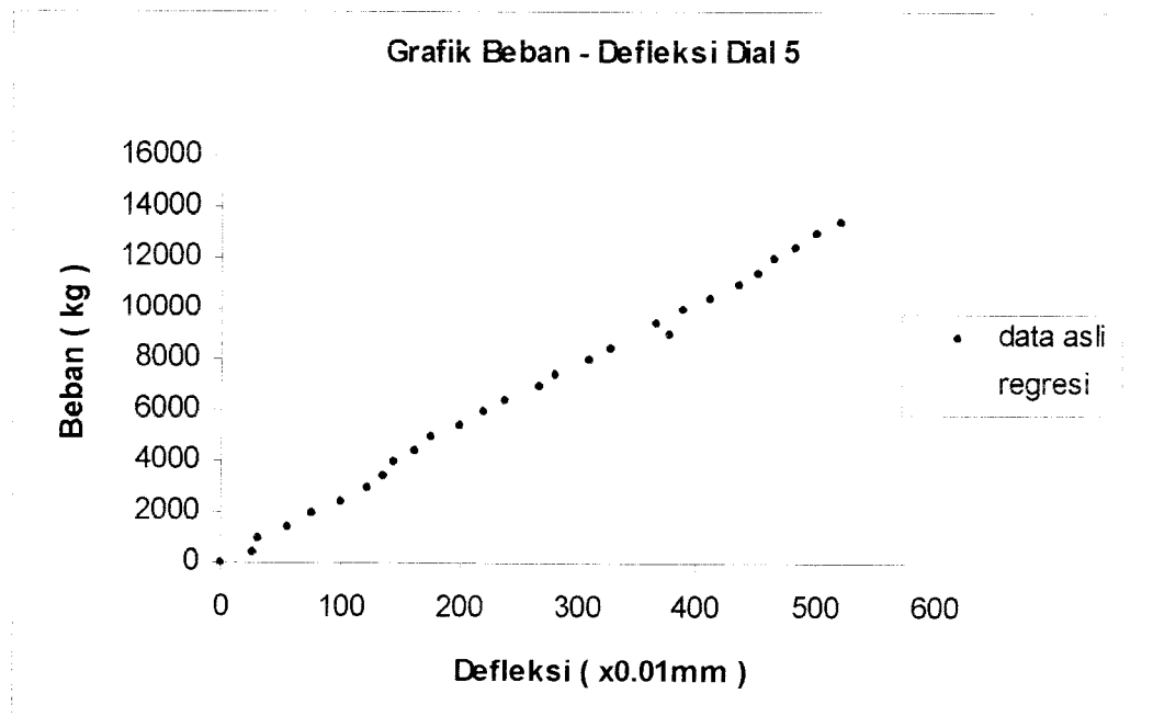
Gambar 5.69 Grafik Beban – Defleksi Dial 5 Benda Uji 1,9m / B / 4
