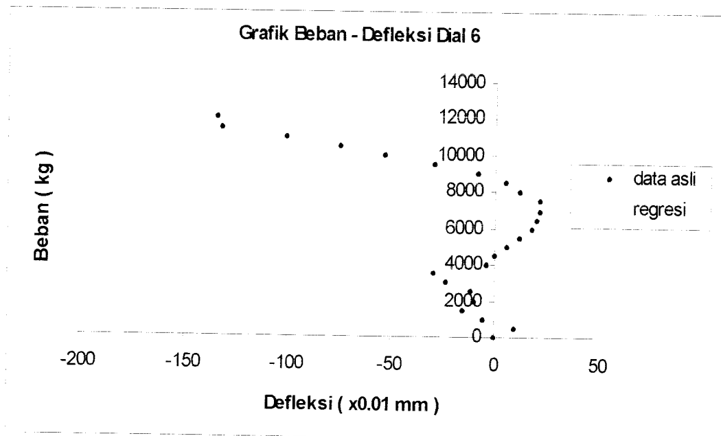
Gambar 5.58 Grafik Beban – Defleksi Dial 6 Benda Uji 1,6m / C / 3
