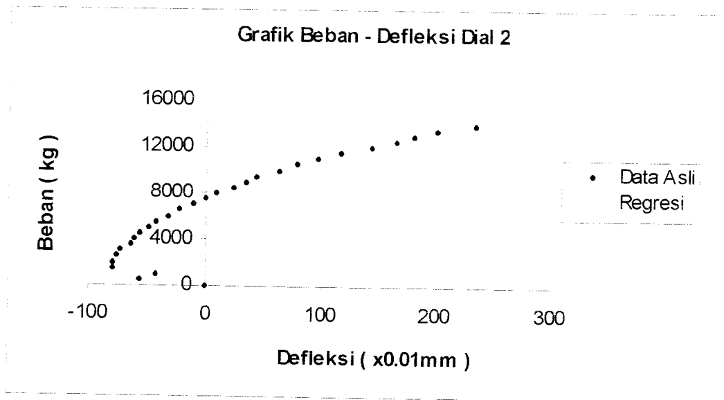
Gambar 5.7 Grafik Beban – Defleksi Dial 2 Benda Uji 1,0m / A / 1
