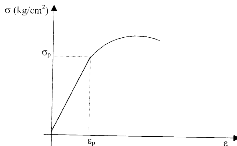
Gambar 3.2 Grafik Tegangan-Regangan
