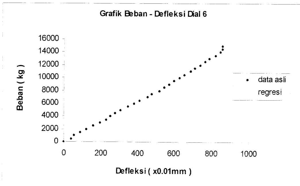
Gambar 5.70 Grafik Beban – Defleksi Dial 6 Benda Uji 1,9m / B / 4
