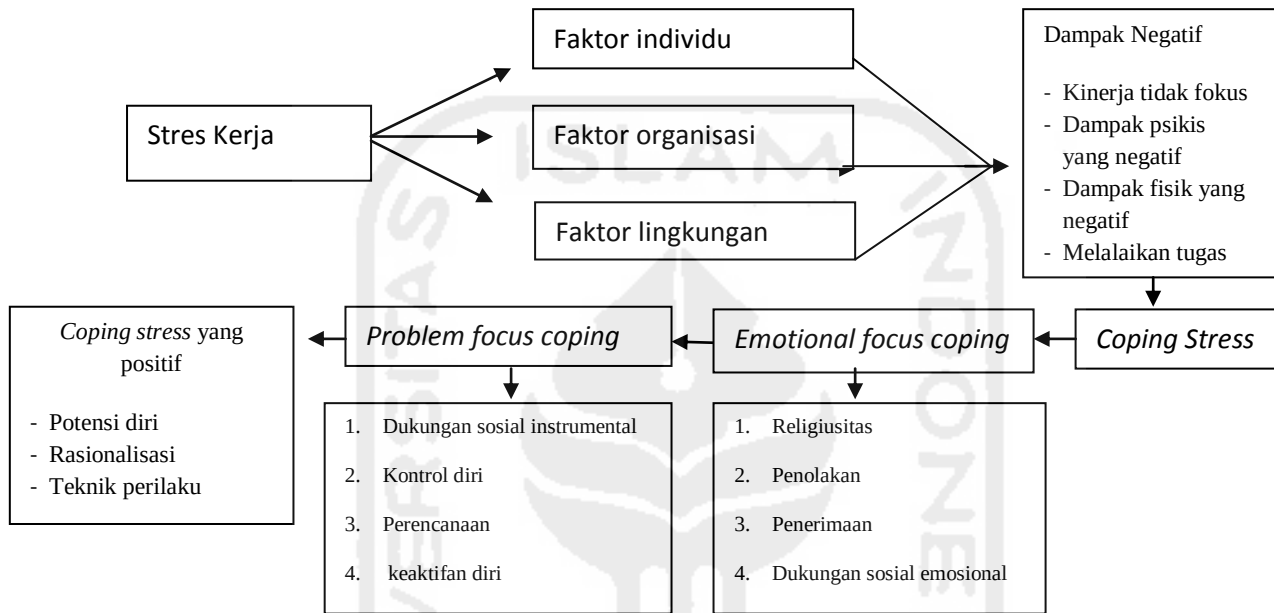
Gambar 1. Kerangka Berfikir
