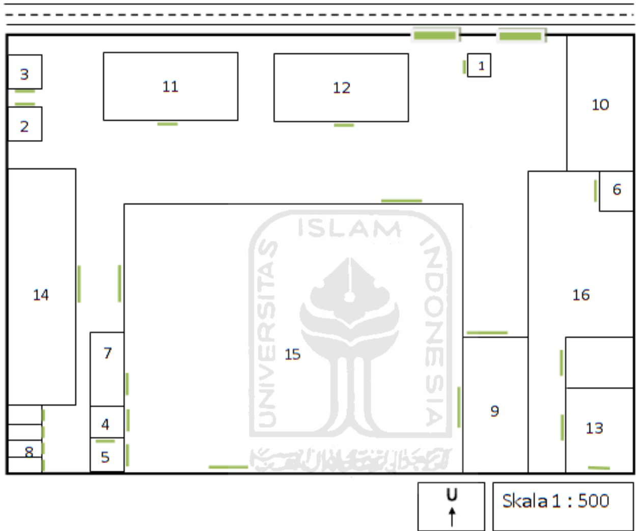
Gambar 4.1 Rencana layout pabrik
