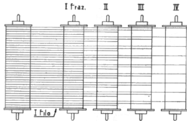
Gambar 3.2 Proses Penggulungan Pada Beam Tenun ( Beaming )
