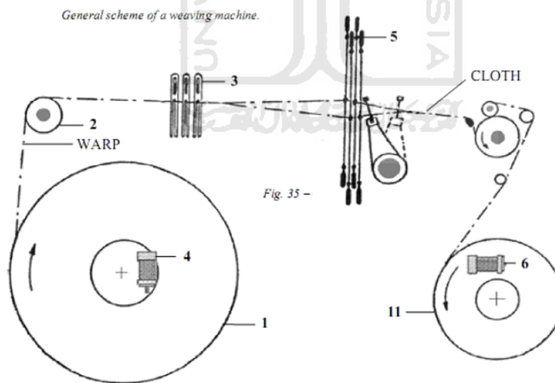
Gambar 3.5 Skema Mesin Tenun
