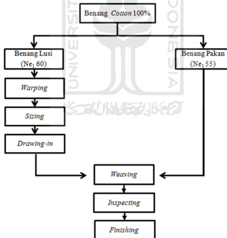
Gambar 3.1 Alur proses pembuatan kain tenun
