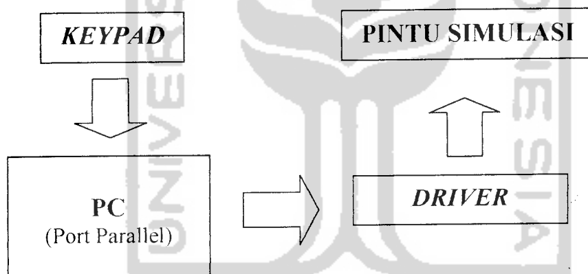
Gambar 3.1 Blok Diagram Sistem Presensi dan Pengaman Pintu
