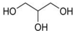
Gambar 2. Struktur Gliserin (13)
