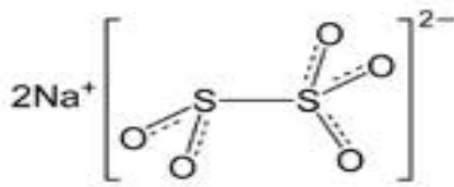
Gambar 5. Struktur natrium metabisulfit (13)
