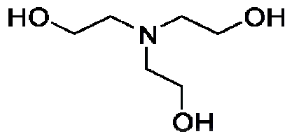
Gambar 3. Struktur Trietanolamine (13)
