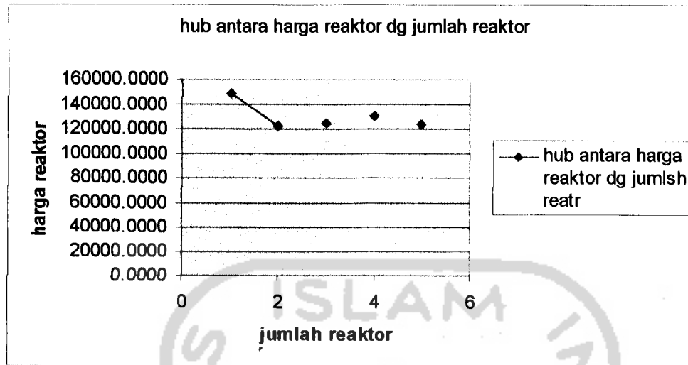
Gambar 1.1. Optimasi jumlah reaktor
