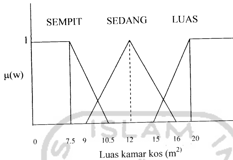
Gambar 3.20 variabel luas kamar
