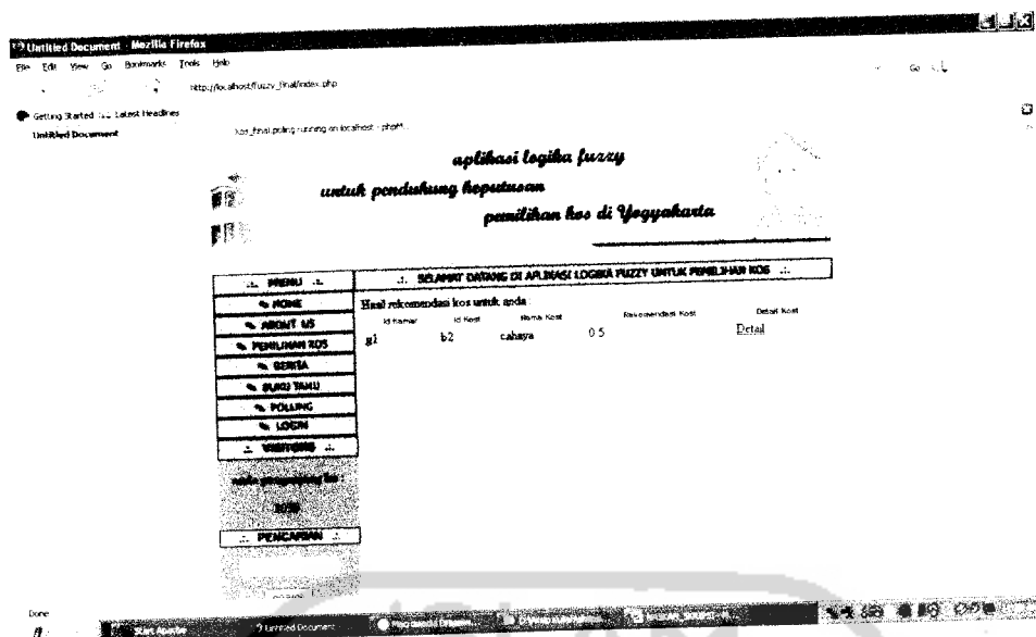
Gambar 4.13 Hasil rekomendasi
