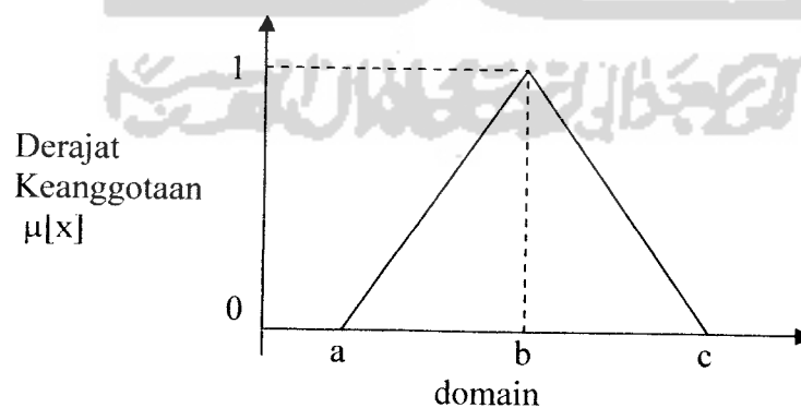
Gambar 2.3 gambar segitiga naik
