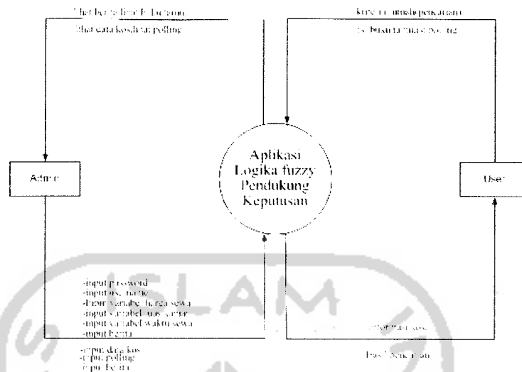
Gambar 3.1 Diagram konteks
