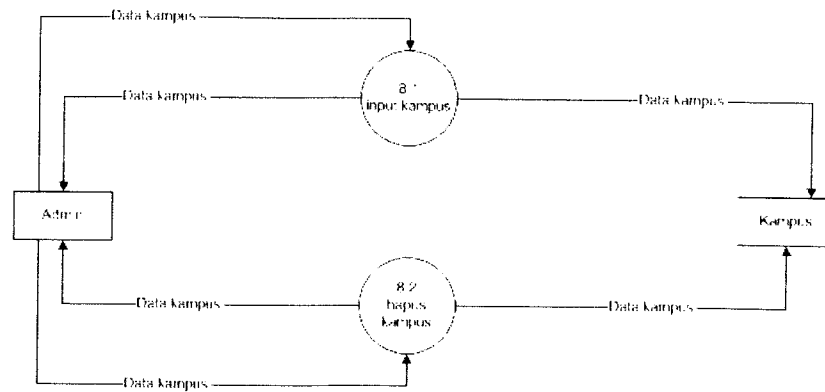
Gambar 3.10 DFD level 2 pengolahan kampus
