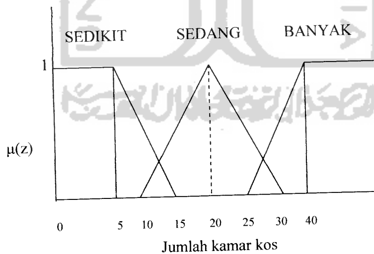
Gambar 3.19 variabel jumlah kamar
