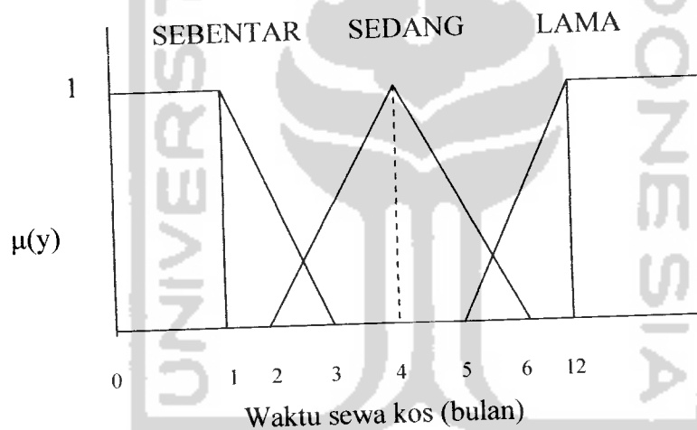
Gambar 3.18 variabel waktu sewa
