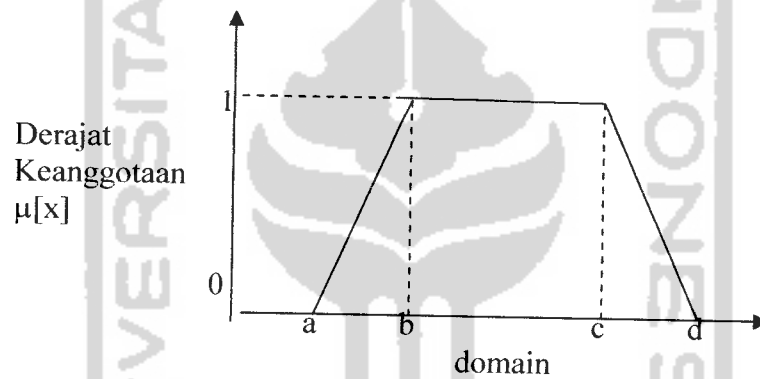
Gambar 2.4 kurva trapesium naik
