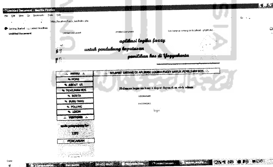
Gambar 3.42 Halaman Login
