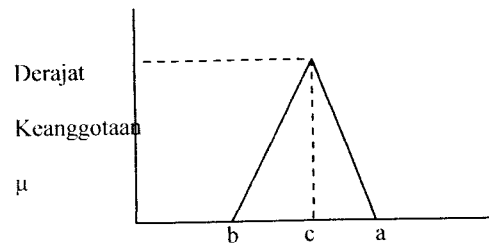
Gambar 3.15 Kurva segitiga
