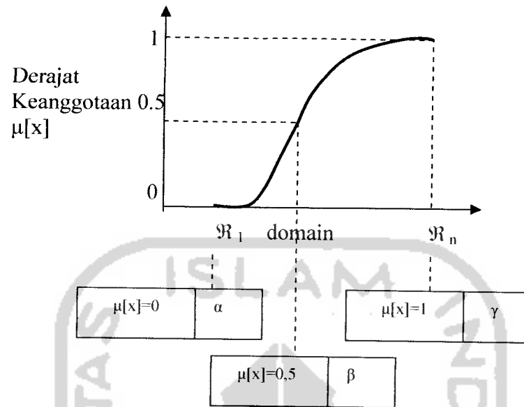
Gambar 2.7 kurva -S PERTUMBUHAN
