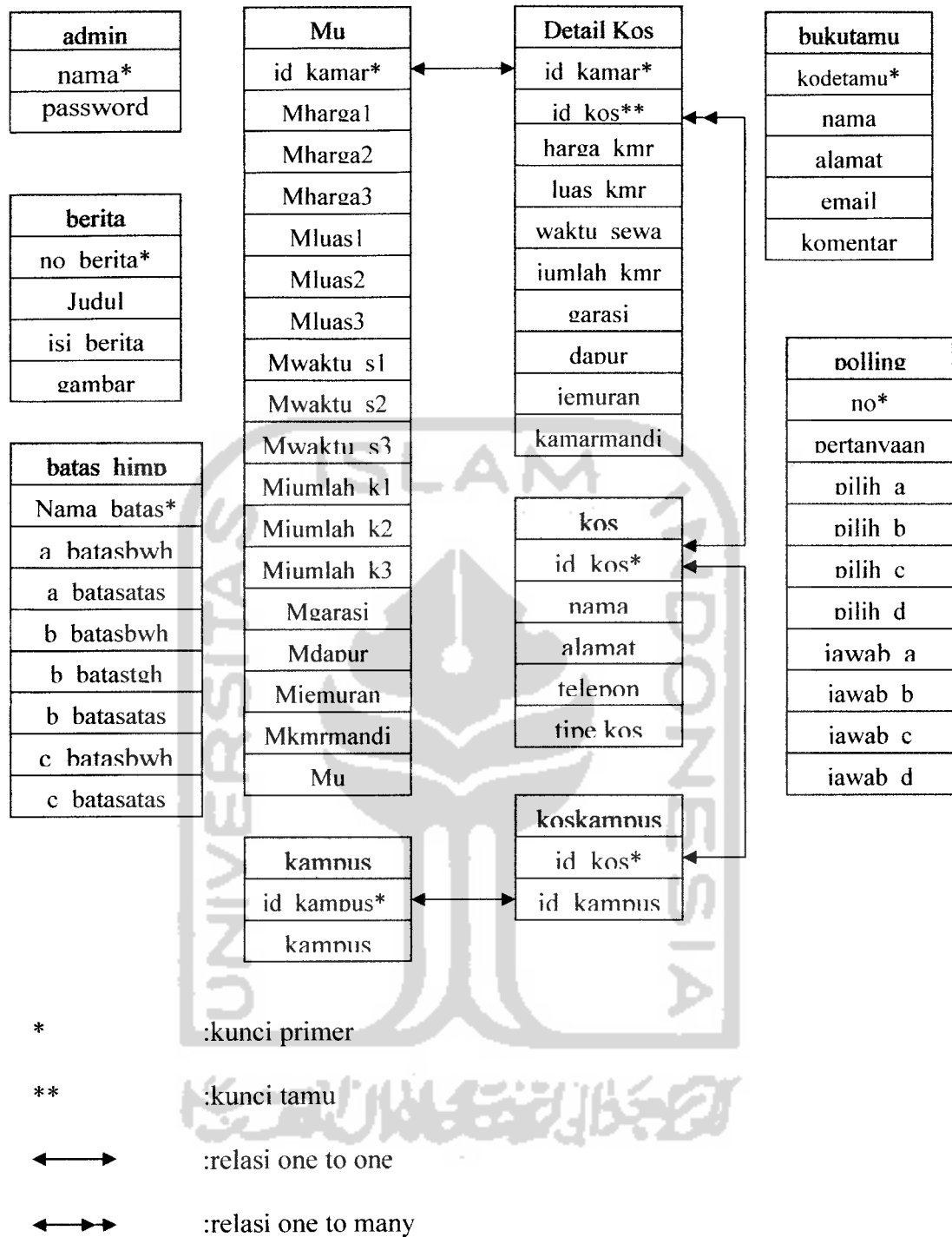
Gambar 3.21 Relasi Tabel
