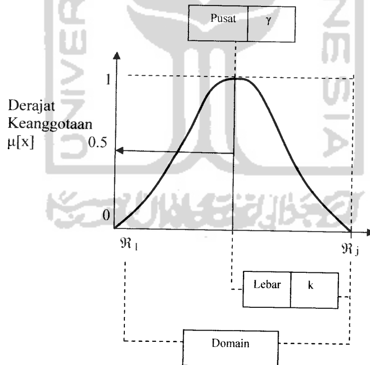
Gambar 2.10 Karakteristik fungsional kurva GAUSS
