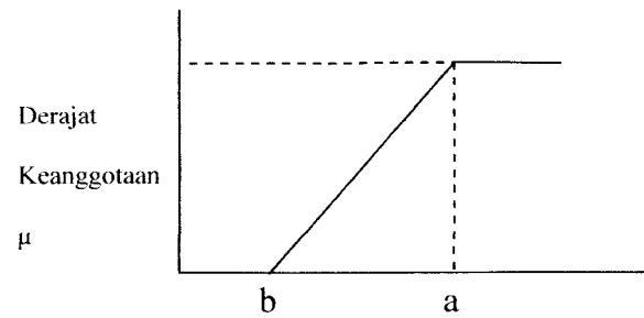
Gambar 3.13 Kurva bahu kanan
