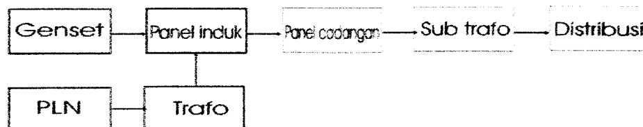
Gambar 4.14 Sistem jaringan
