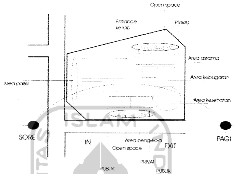
Gambar 4.6 Tanggapan site
