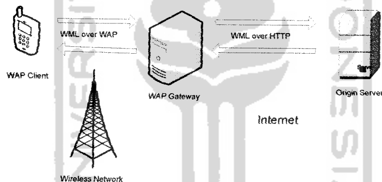
Gambar 2.2 Arsitektur WAP
