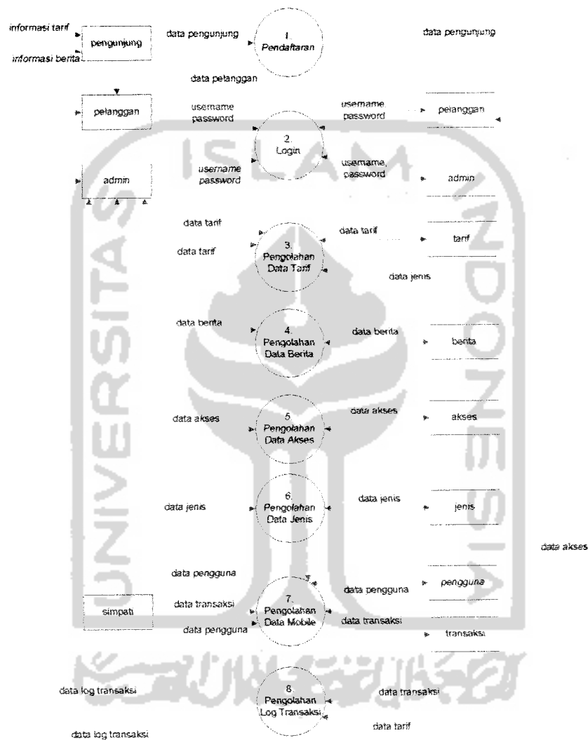
Gambar 3.2 DFD Level 1
