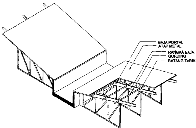
POTONGAN STRUKTUR
