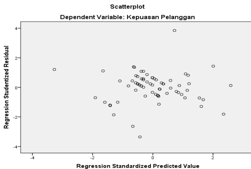
Gambar 4.1 Scatter Plot Uji Heteroskerdastisitas
