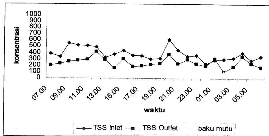
Gambar 5.19 Grafik perbandingan konsentrasi TSS dengan standart
