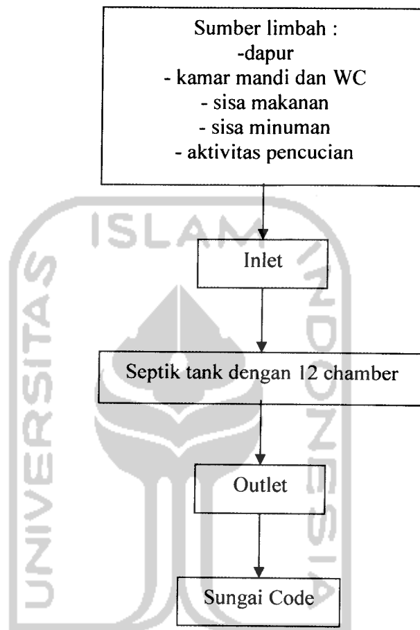
Gambar 2.4 Diagram Alir IPAL Komunal Jetis Harjo Jogjakarta (Sumber : Hasil Penelitian, 2007)
