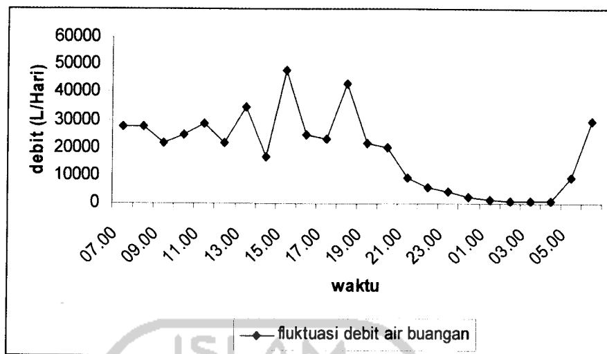
Gambar 5.17 Gambar Fluktuasi Debit Air Buangan Domestik
