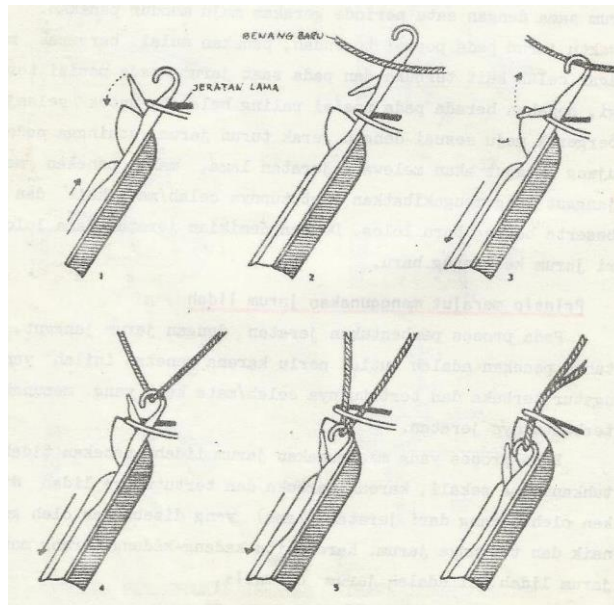
Gambar 1. 7 Prinsip Kerja Jarum Lidah
