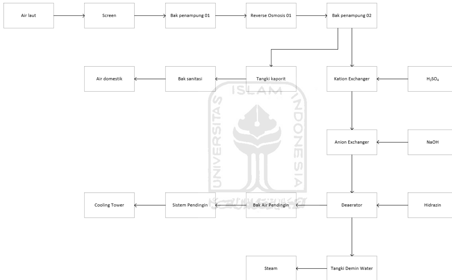
Gambar 4. 6 Diagram alir proses pengolahan air laut
