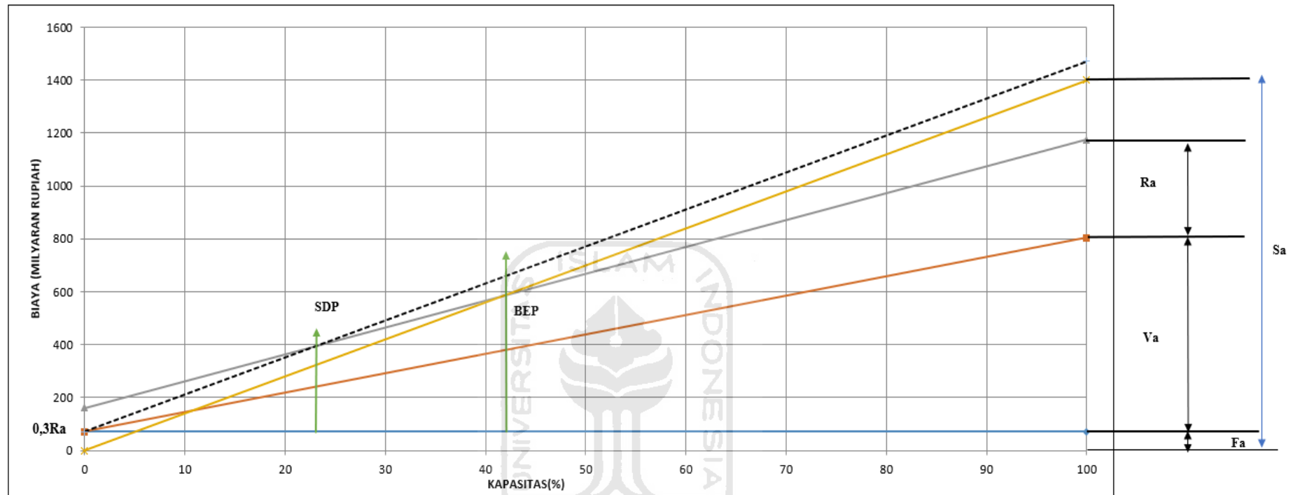
Gambar 4. 8 Grafik Hubungan Kapasitas dengan Biaya
