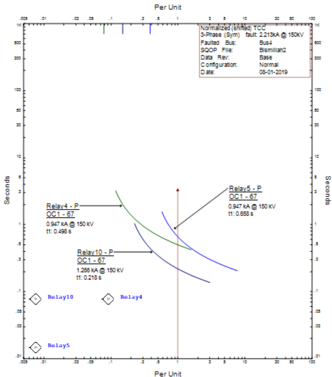
Gambar 4.6 Grafik koordinasi saat posisi gangguan di Bus 4
