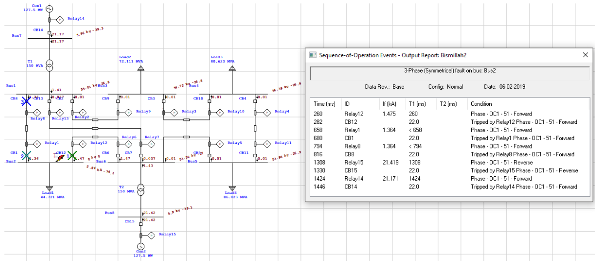
Gambar 4.1 Hasil koordinasi saat posisi gangguan di Bus 2
