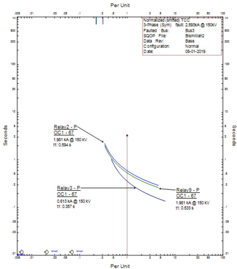
Gambar 4.4 Grafik koordinasi saat posisi gangguan di Bus 3
