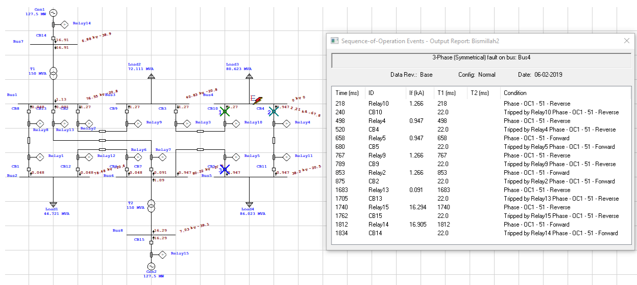
Gambar 4.5 Hasil koordinasi saat posisi gangguan di Bus 4
