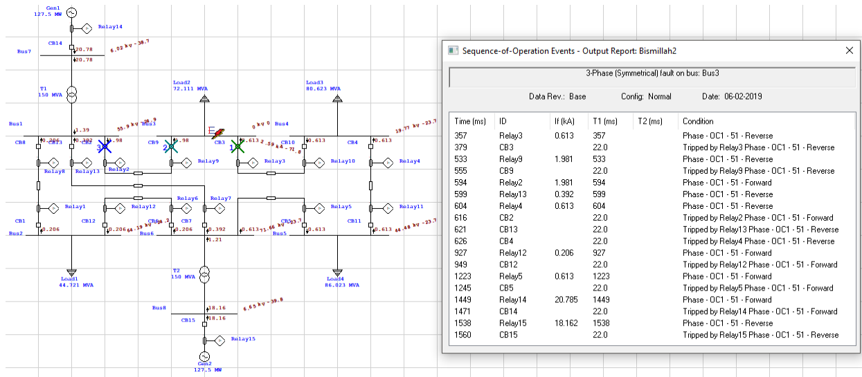
Gambar 4.3 Hasil koordinasi saat posisi gangguan di Bus 3
