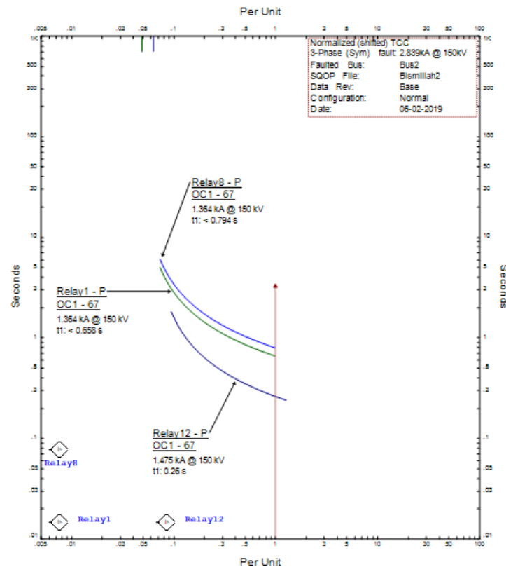
Gambar 4.2 Grafik koordinasi saat posisi gangguan di Bus 2
