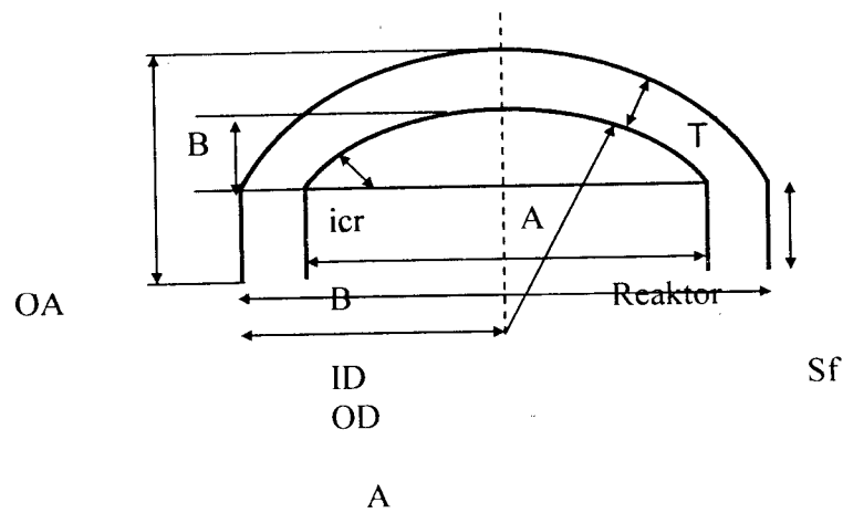
Gambar. Dimensi tutup reaktor
