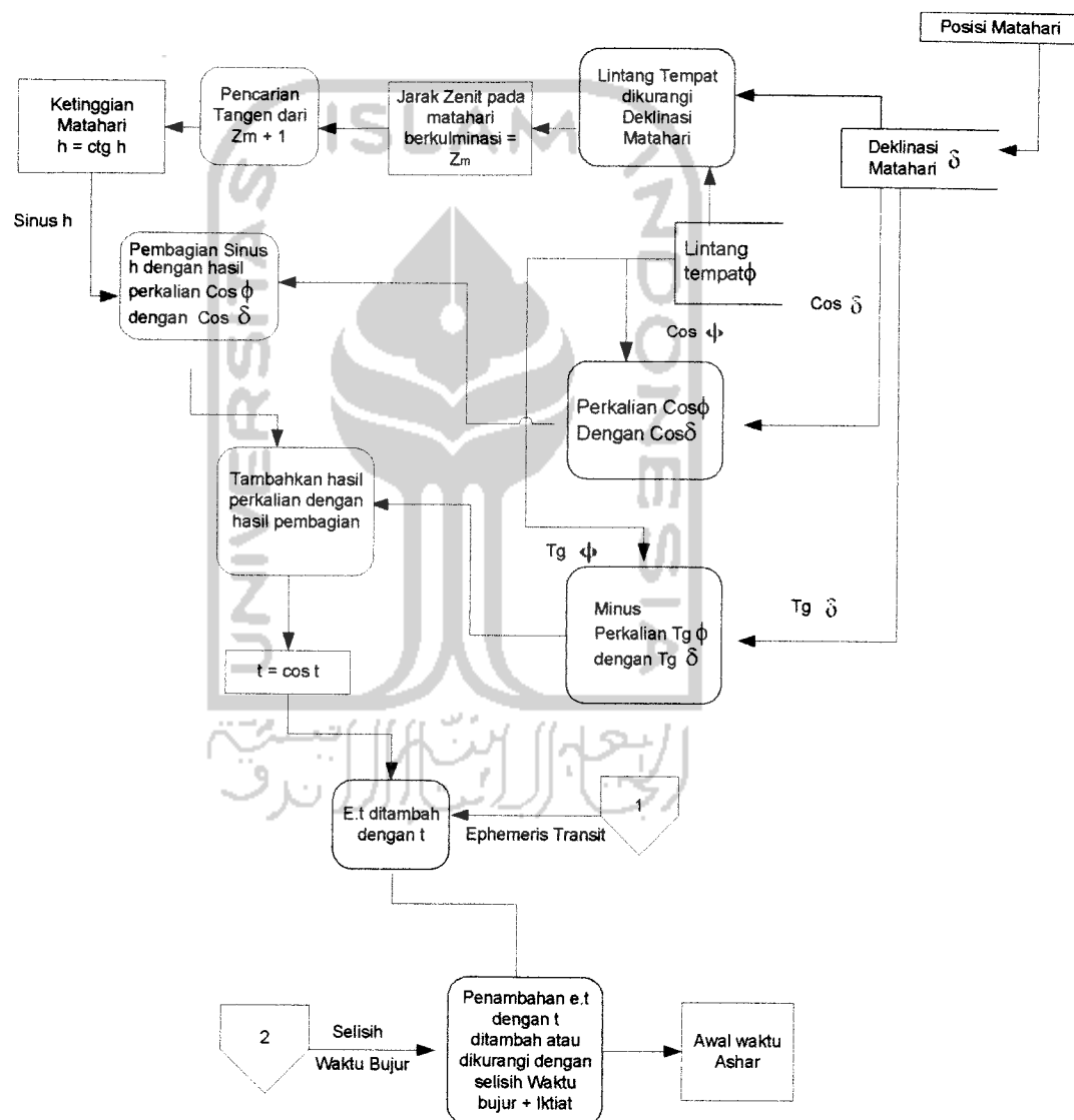
Gambar 4.5. Pencarian jadwal waktu sholat ashar
