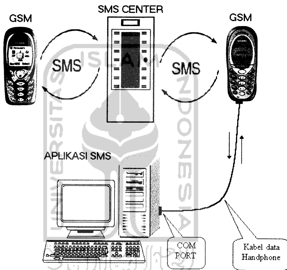
Gambar 2.3. Mekanisme sistem aplikasi komputasi jadwal awal sholat berbasis SMS dengan ilmu falak
