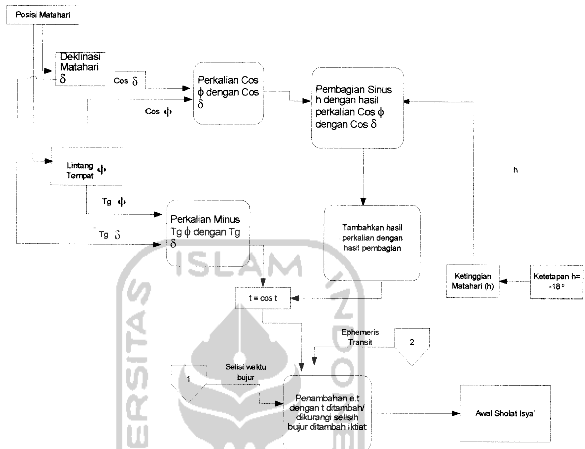
Gambar 4.8. Pencarian awal waktu sholat isya'
