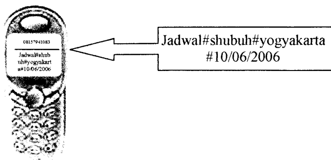
Gambar 6.4. Kaidah format request sms sebagai input dari handphone
