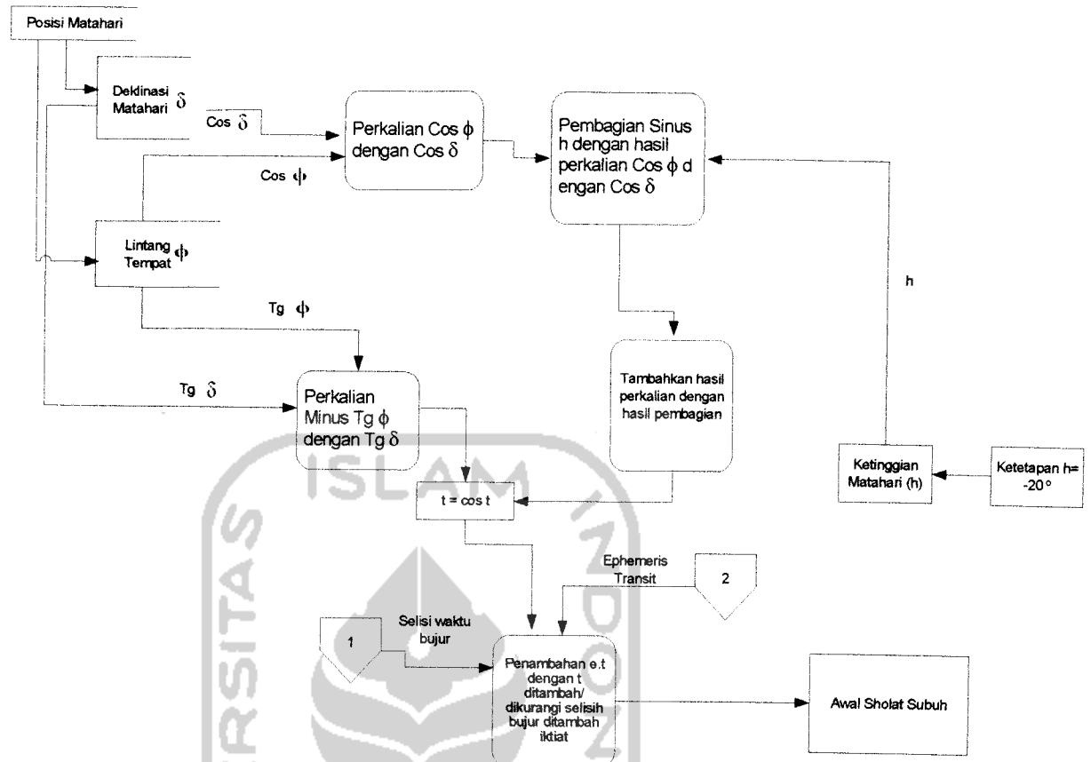
Gambar 4.9. Pencarian awal waktu sholat shubuh.
