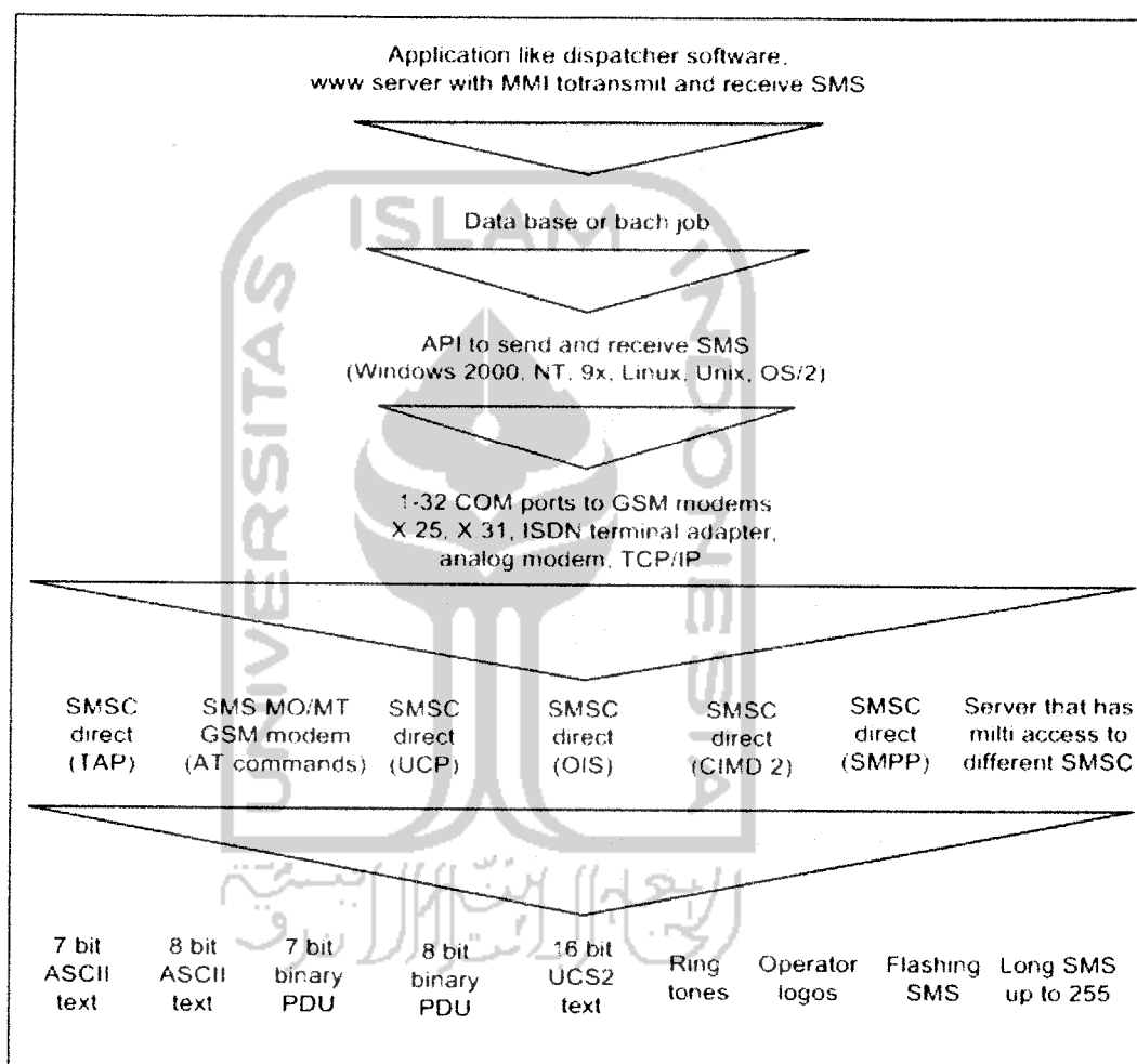
Gambar 2.2. Tipe koneksi SMS center
