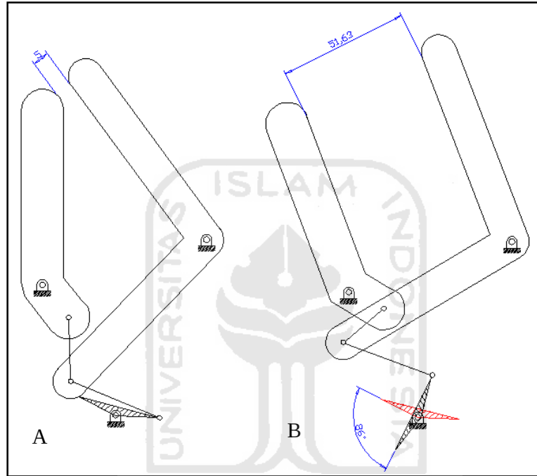
Gambar 5-4 mekanik denga AutoCAD
