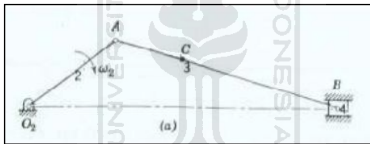
Gambar 2-7 Mekanisme engkol peluncur (Holowenko, 1985)
