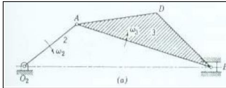
Gambar 2-8 Mekanisme empat penghubung (Holowenko, 1985)
