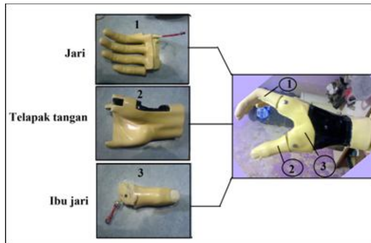
Gambar 4-15 Pemisahan bagian mekanik.
