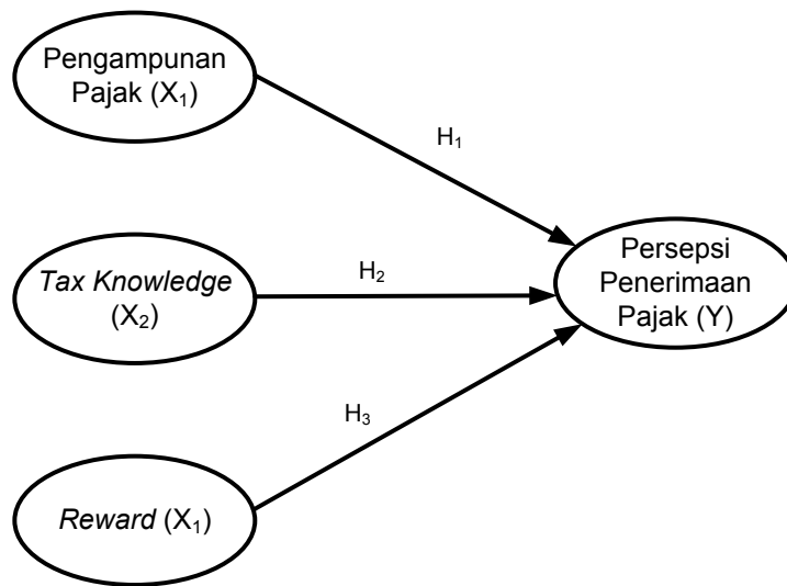
Gambar 2.2 Kerangka Pemikiran
