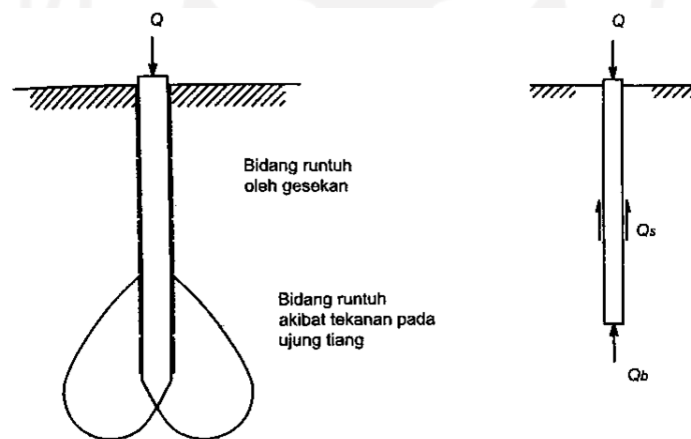
(a) Bidang runtuh pada tiang tekan (b) Tahanan ujung dan tahanan gesek
