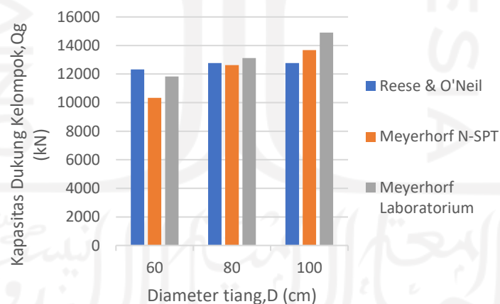
Gambar 5.17 Perbandingan Kapasitas Dukung Tiang Kelompok
