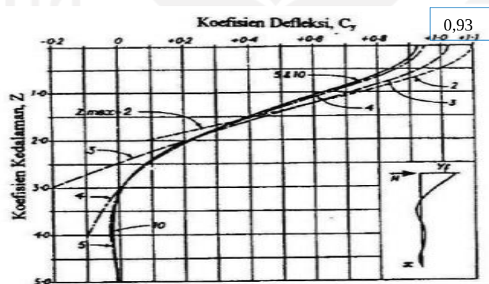
Gambar 5.15 Koefisien C_y Pondasi Tiang pada Tanah Granuler
