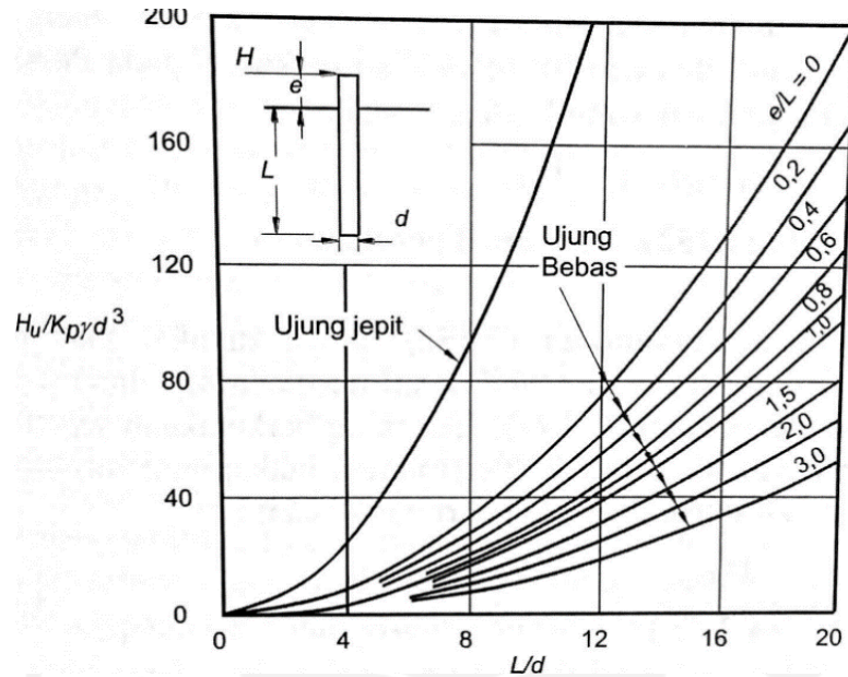
(a) Tiang ujung pendek
