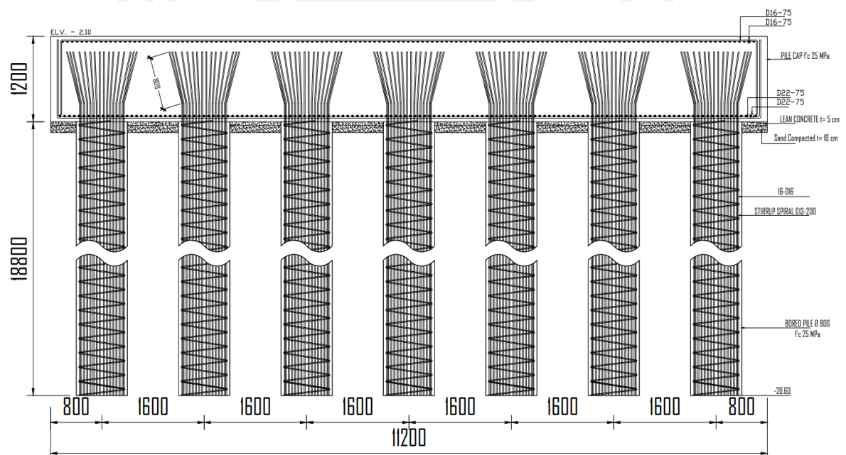
Gambar 5.10 Potongan Melintang Pondasi Tipe F-B
