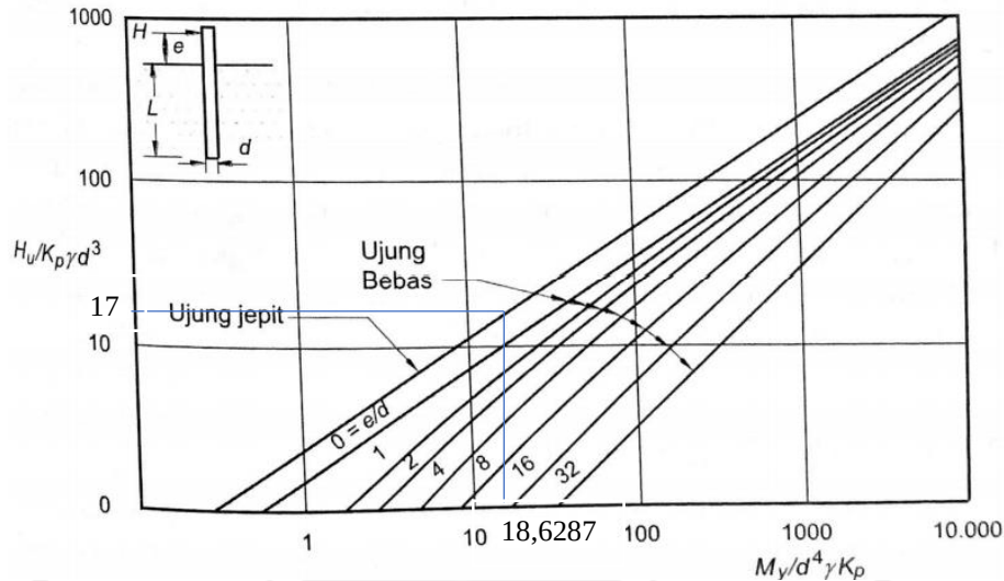
Gambar 5.14 Daya Dukung Ujung Batas Tiang Bor pada Tanah Granuler
