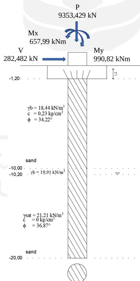
Gambar 5.12 Pemodelan Struktur Beban pada Pondasi Bored Pile
