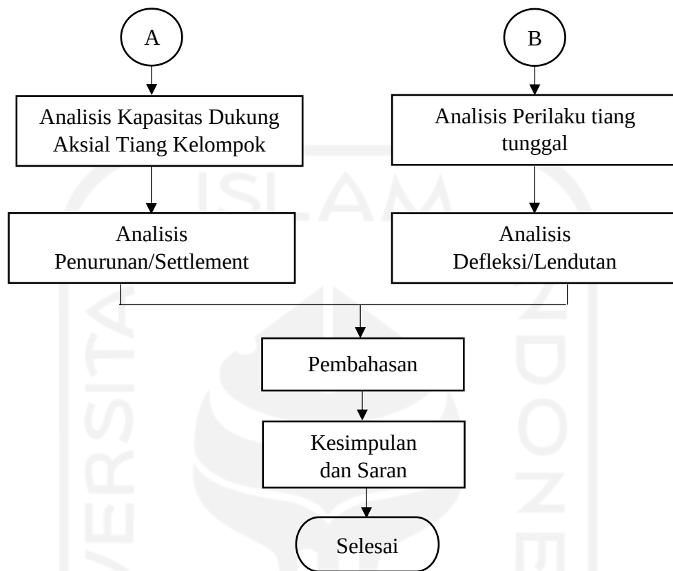
Gambar 4.2 Bagan Alir Penelitian
