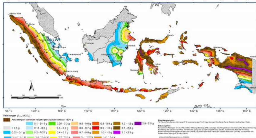
Gambar 3. 9 Peta Wilayan Percepatan Batuan Dasar Pada Perioda 1 detik ( S_1 )
