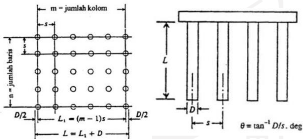
Gambar 3.7 Efisiensi Kelompok Tiang
