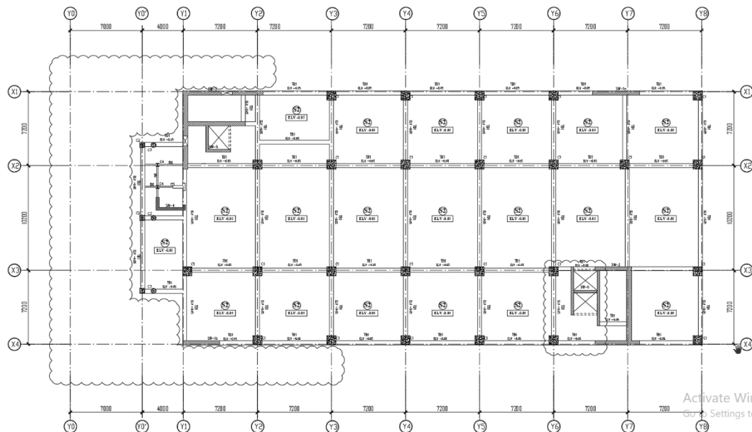
Gambar 5.1 Denah Konstruksi Gedung APSLC UGM (Sumber : PT. Pembangunan Perumahan (Persero) Tbk)
