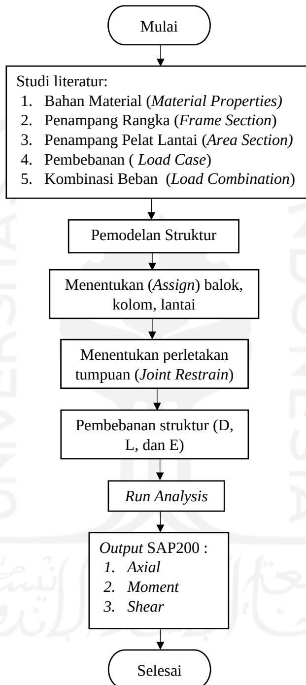
Gambar 4.3 Bagan Alir SAP2000
