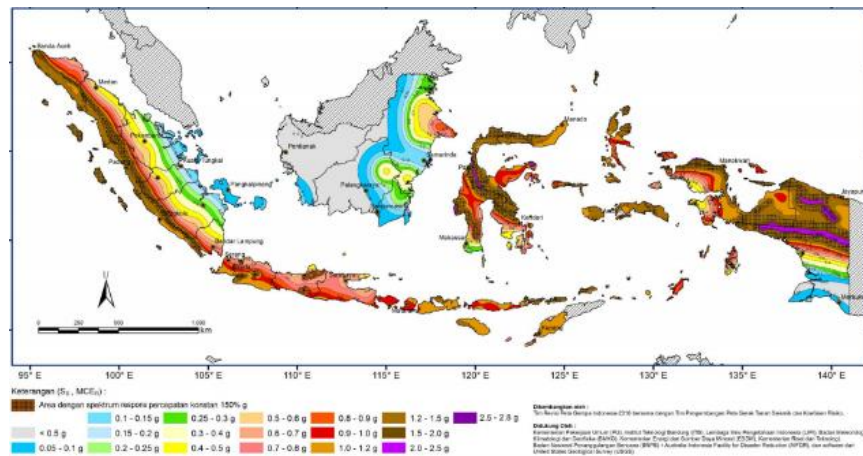
Gambar 3. 8 Peta Wilayan Percepatan Batuan Dasar Pada Perioda Pendek ( S_s )
