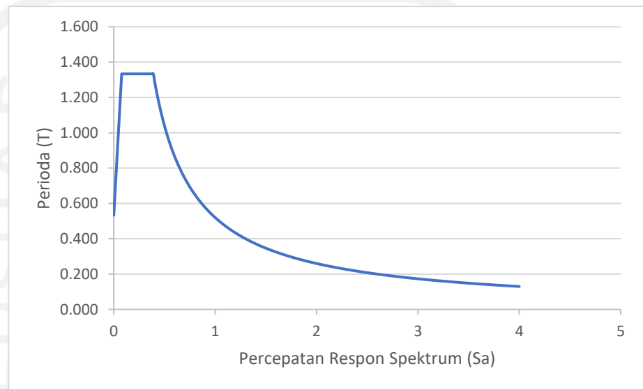
Gambar 5.5 Hasil Respon Spektrum
