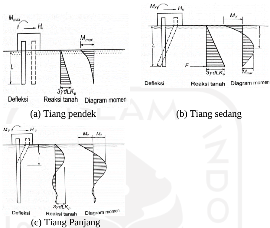
Gambar 3. 5 Tiang ujung jepit dalam tanah granuler (Broms,1964)
