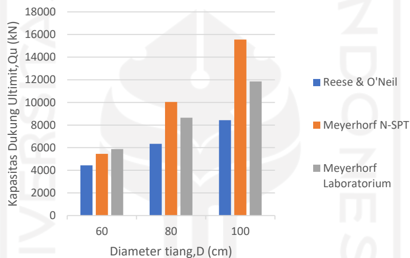
Gambar 5.16 Perbandingan Kapasitas Dukung Pondasi Tiang Tunggal
