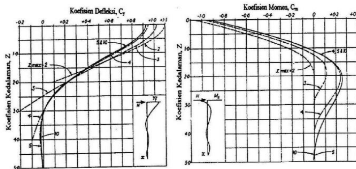
Gambar 3. 6 Grafik Koefisien Cy dan Cm Pondasi Tiang
