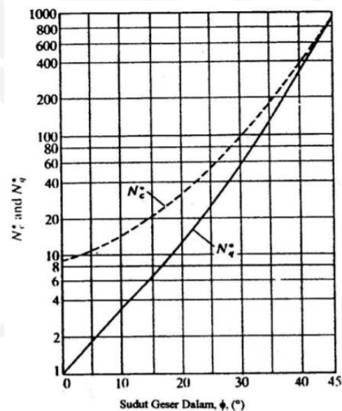
Gambar 3.2 Faktor Daya Dukung Ujung N_c^* dan N_q^*
