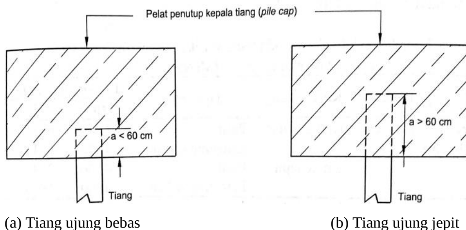
Gambar 3.3 Definisi tiang ujung jepit dan ujung bebas (McNulty, 1956)
