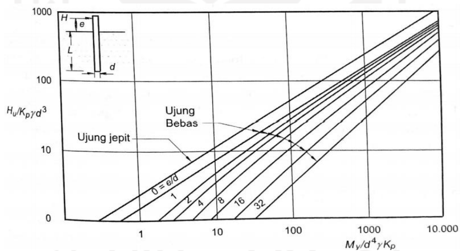
(b) Tiang ujung panjang
