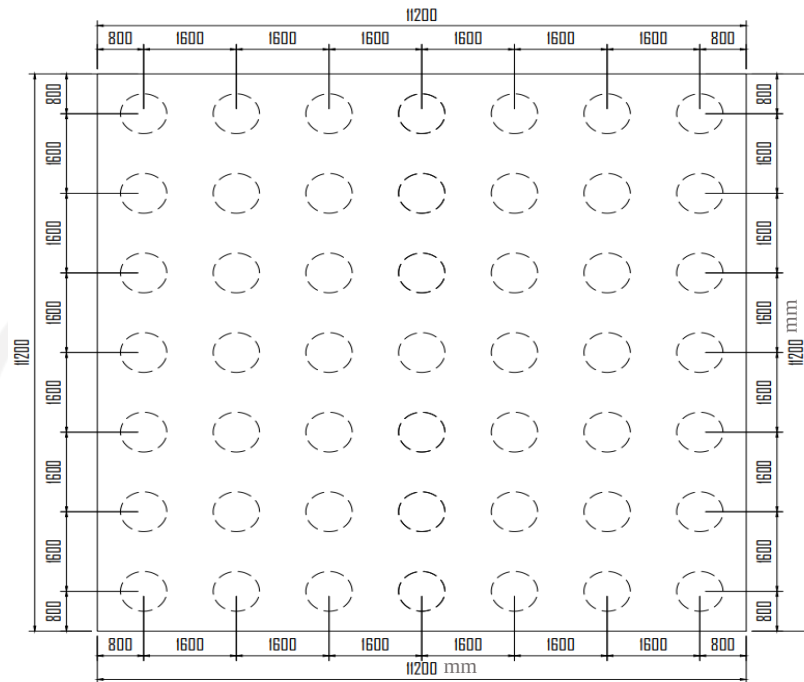
Gambar 5.9 Tampak Atas Pondasi Tipe F-B
