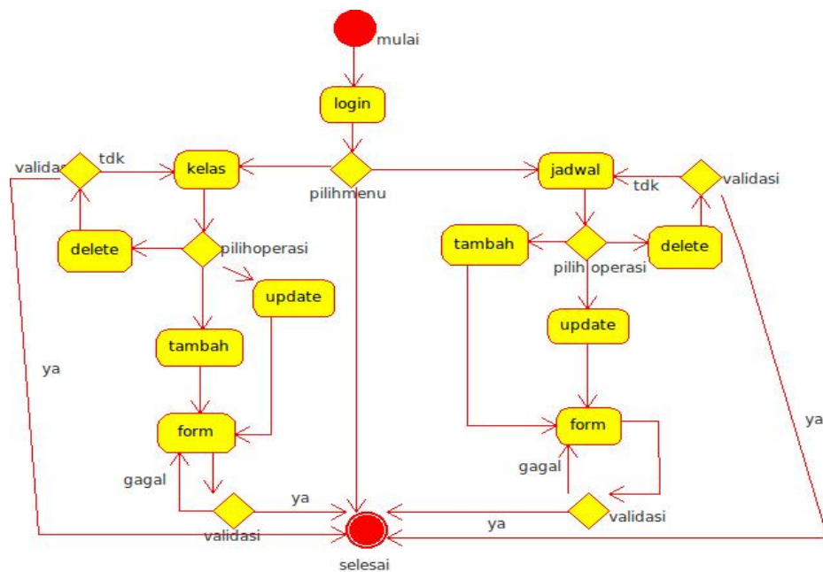
Gambar 3.5 Activity Diagram Manajemen Kelas dan Penjadwalan
