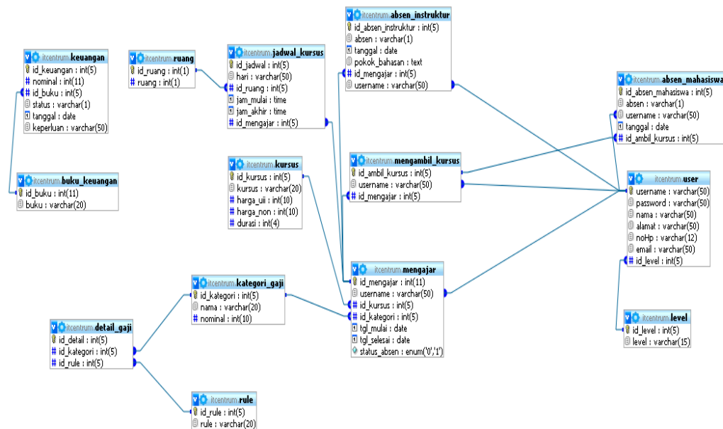
Gambar 3.10 Relasi Antar Tabel Database Sistem
