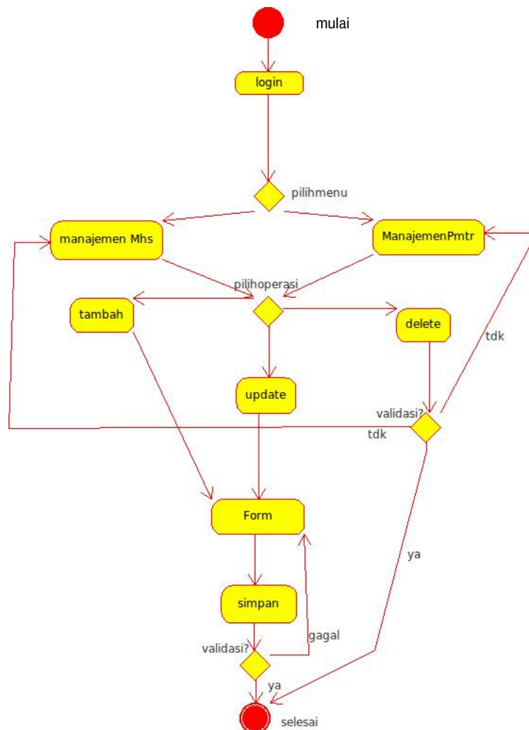
Gambar 3.4 Activity Diagram Manajemen Mahasiswa dan Instruktur
