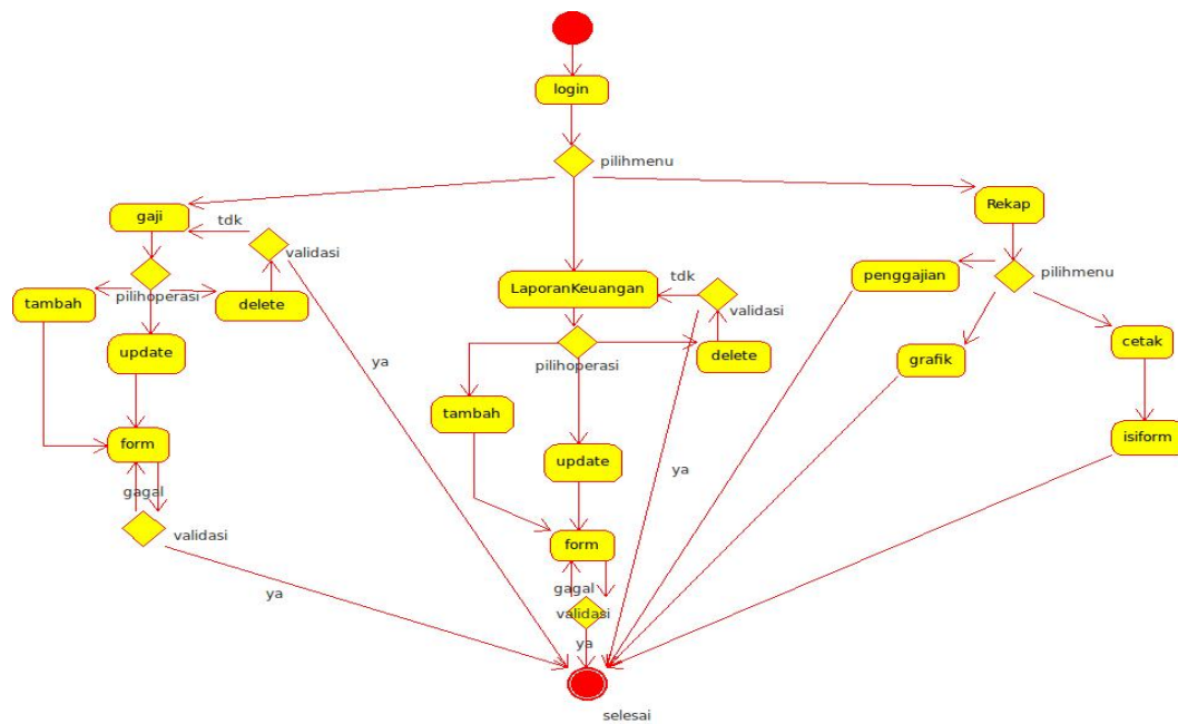
Gambar 3.6 Activity Diagram Manajemen Gaji, Laporan Keuangan dan Rekap
