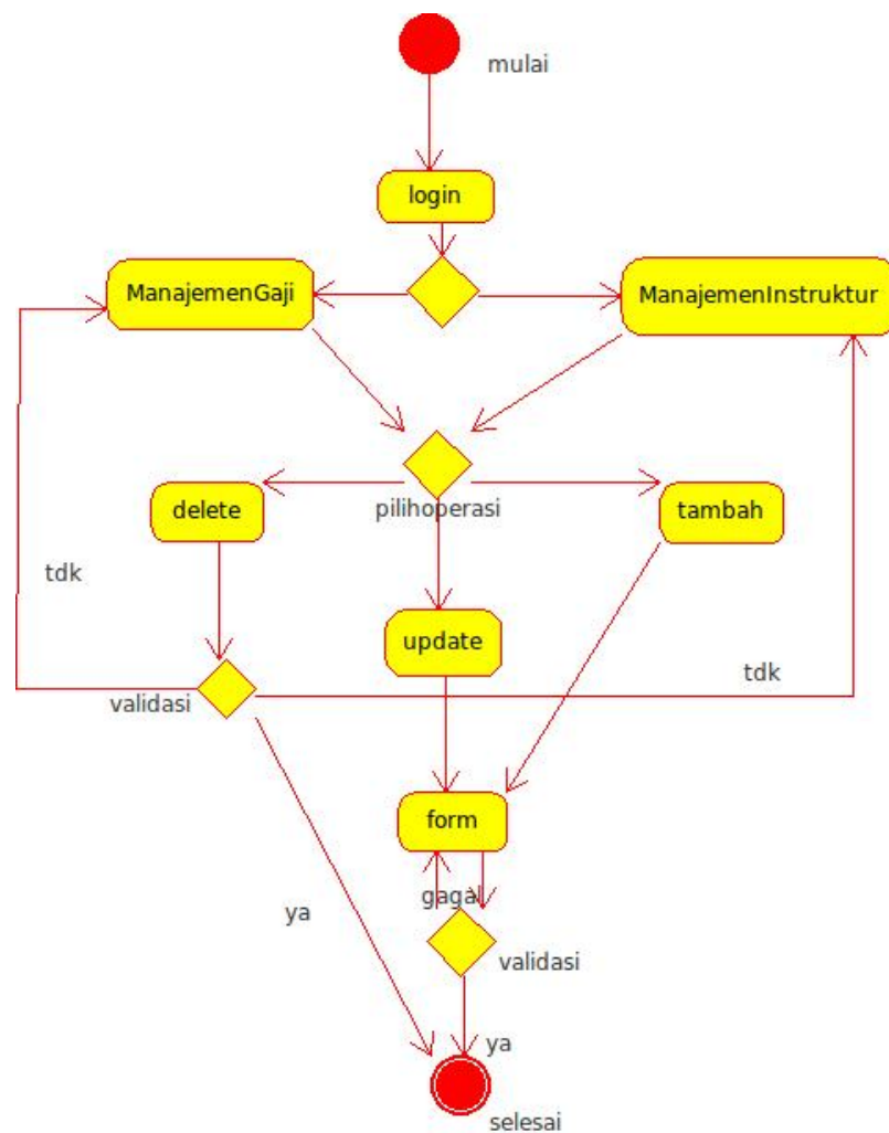
Gambar 3.9 Activity Diagram Direktur
