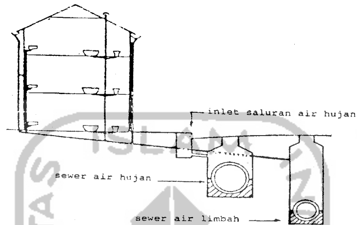
Gambar 3.11 Sistem Terpisah Sebagian (Parsial)
