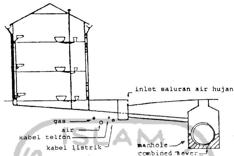
Gambar 3.10 Sistem Tercampur
