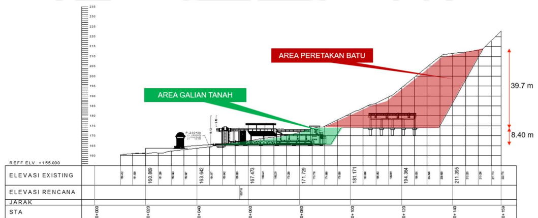
Gambar 4. 3 Gambar Potongan Melintang Area Galian dan Peretakan
