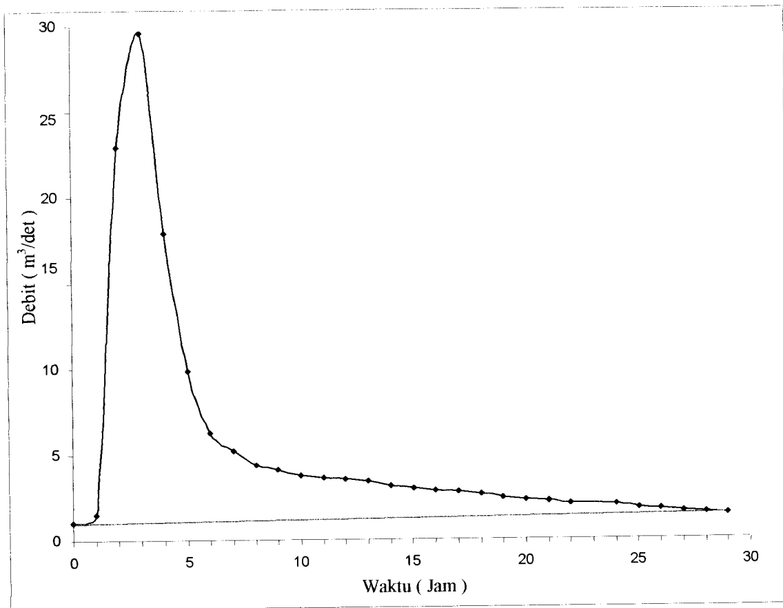
Gambar 5 Pemisahan Aliran Tahun 2000
