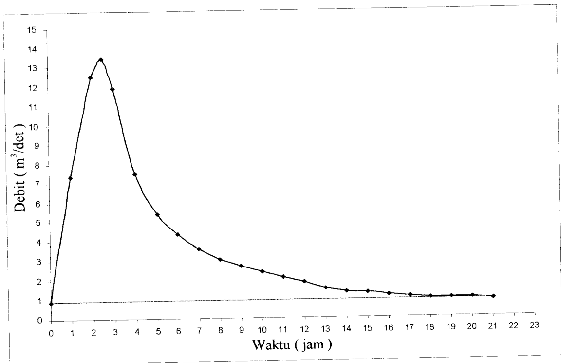
Gambar 1 Pemisahan Aliran Tahun 1994
