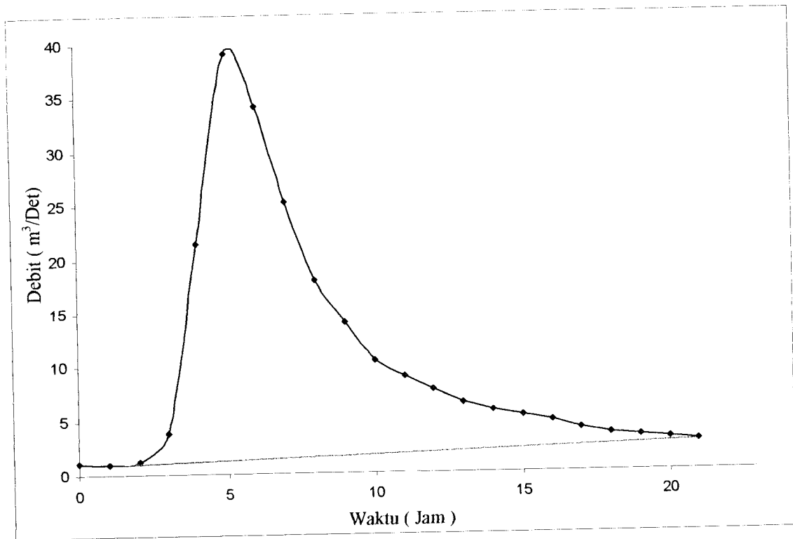
Gambar 3 Pemisahan Aliran Tahun 1996
