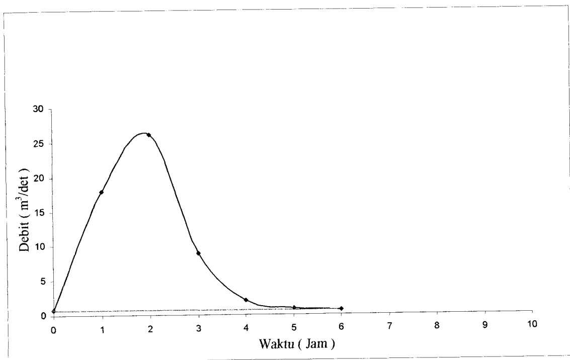
Gambar 6 Pemisahan Aliran Tahun 2001
