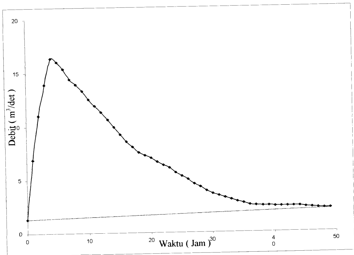
Gambar 2 Pemisahan Aliran Tahun 1995
