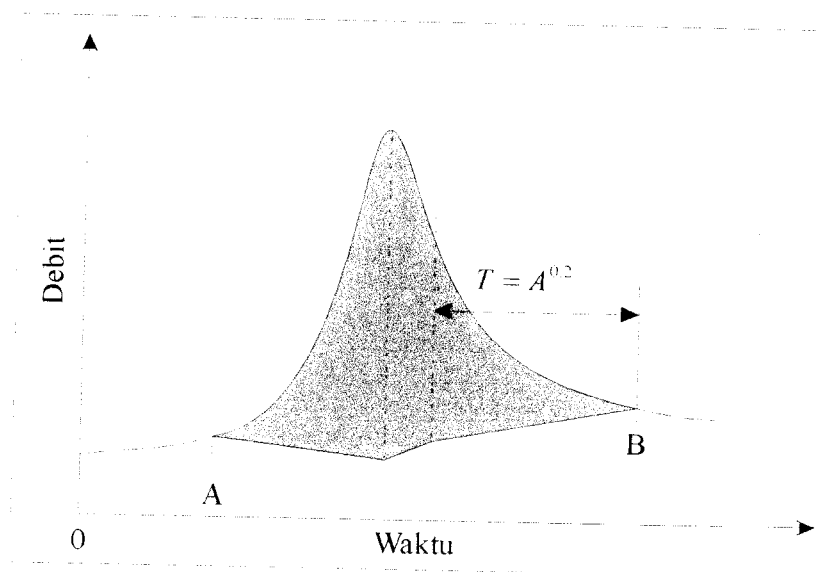
Gambar 3.4 Pemisahan aliran dasar dengan Variable Slope Method
