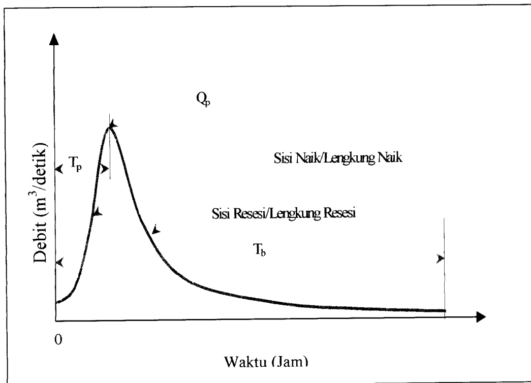
Gambar 3.1 Bagian-bagian hidrograf
