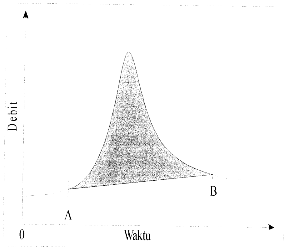
Gambar 3.2 Pemisahan aliran dasar dengan Metode Garis Lurus
