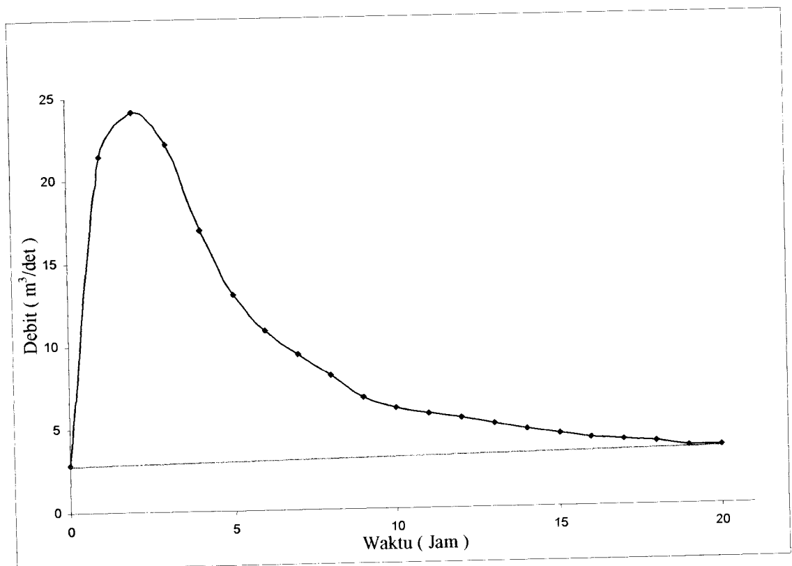
Gambar 4 Pemisahan Aliran Tahun 1999
