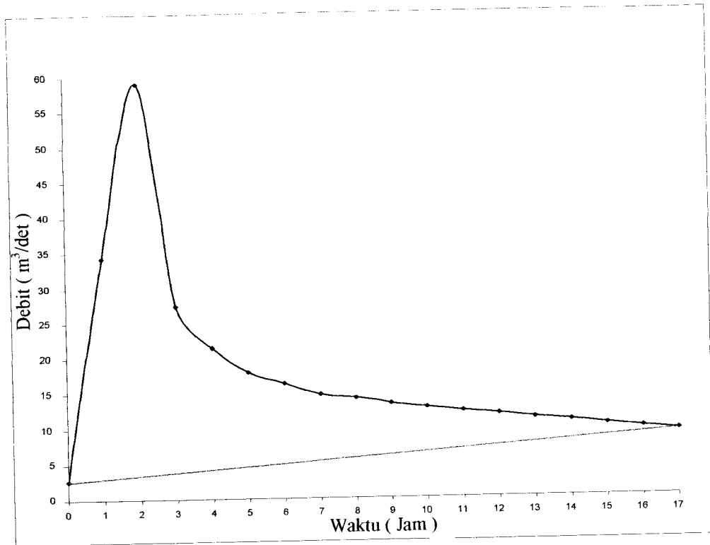
Gambar 7 Pemisahan Aliran Tahun 2002
