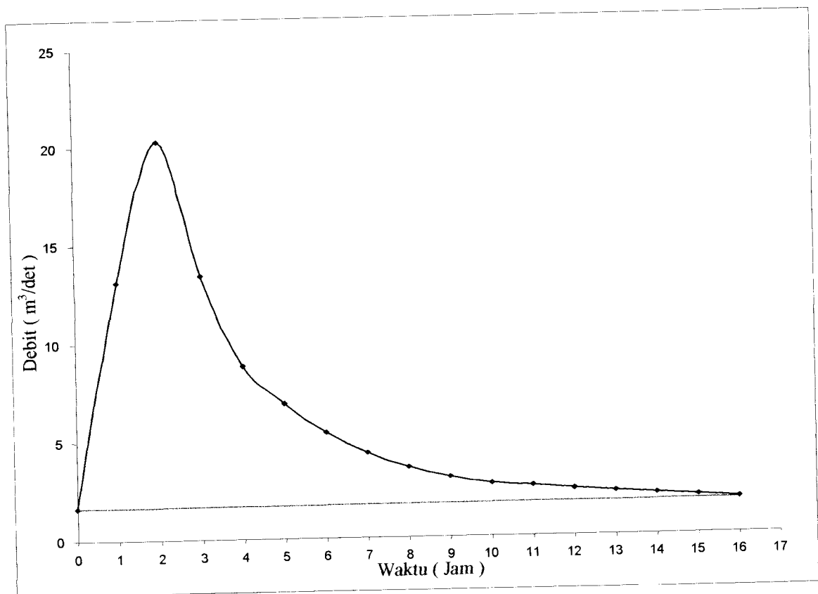
Gambar 8 Pemisahan Aliran Tahun 2003
