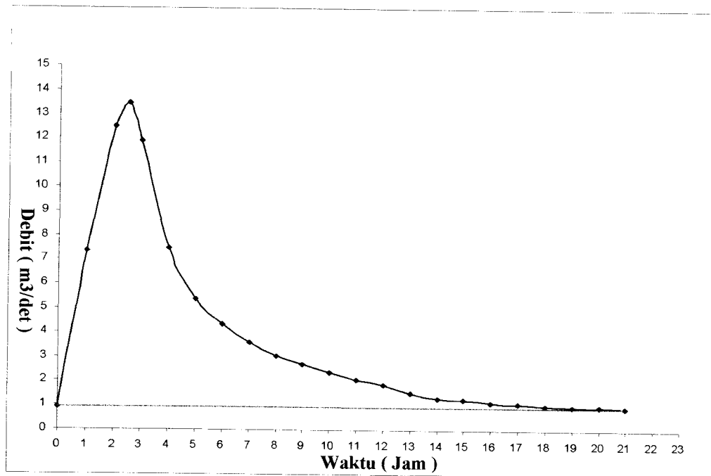
Gambar 5.3 Hidrograf tahun 1994
