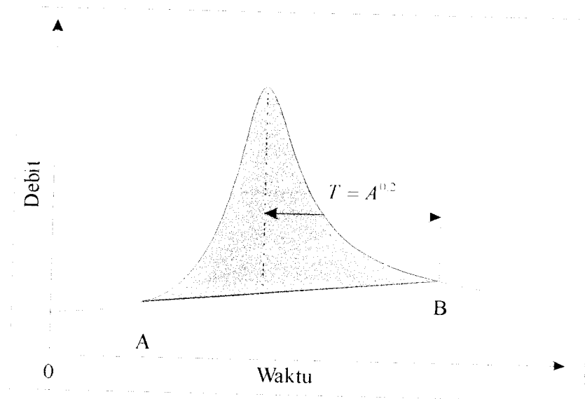
Gambar 3.3 Pemisahan aliran dasar dengan Fixed Base Length
