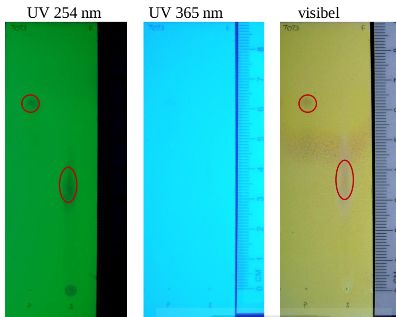
Gambar 11. Hasil Uji Kualitatif Tablet effervescent Buah Naga Dengan Kromatografi Lapis Tipis (KLT)
