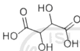
Gambar 3. Struktur molekul asam tartat
