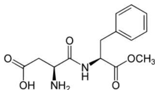
Gambar 5. Struktur molekul aspartam
