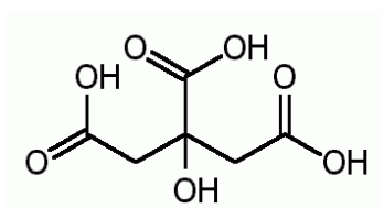
Gambar 2. Struktur molekul asam sitrat
