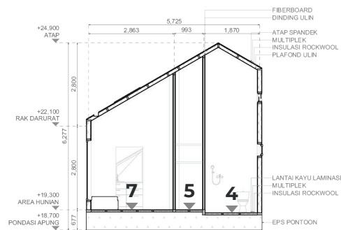
Potongan B
