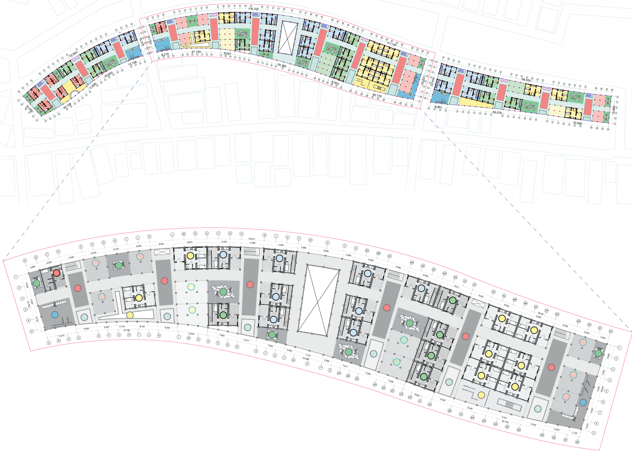
Gambar 69. Lantai 2 - Area Hunian Sumber: Penulis, 2024
