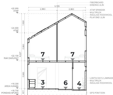
Potongan B
