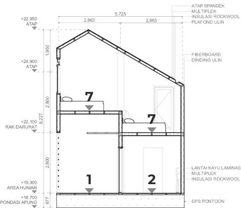
Potongan B
