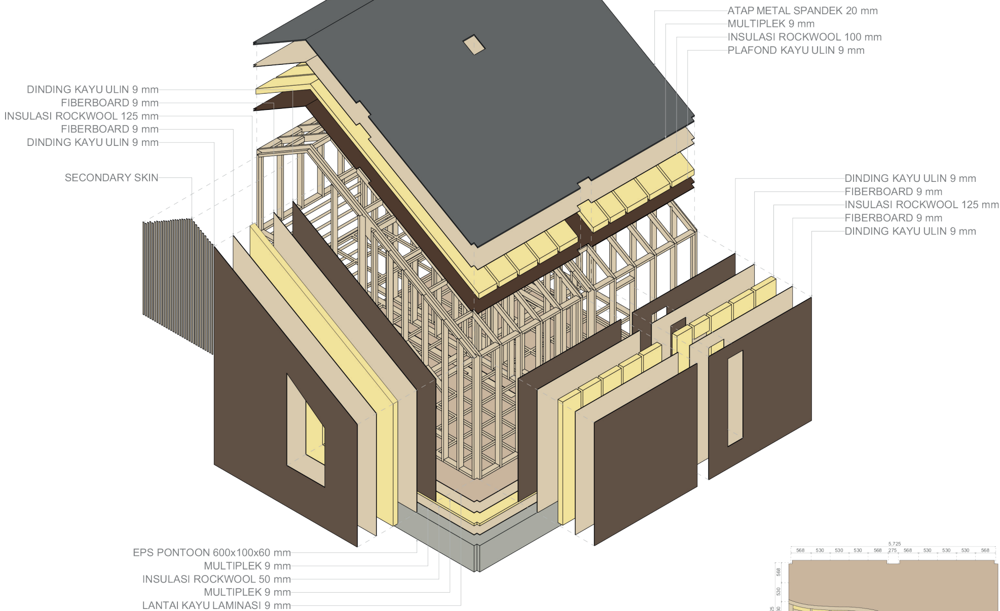
Gambar 75. Detail Selubung Modul Hunian Sumber: Penulis, 2024
