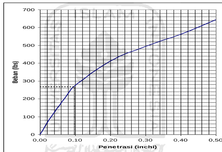
Gambar 6.9 Grafik hubungan beban dan penetrasi uji CBR sampel I
