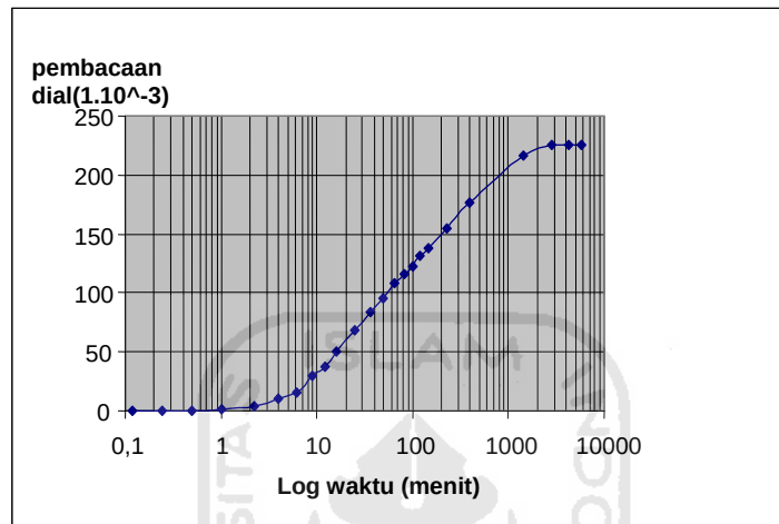
Gambar 5.14 Grafik log waktu vs Swelling
