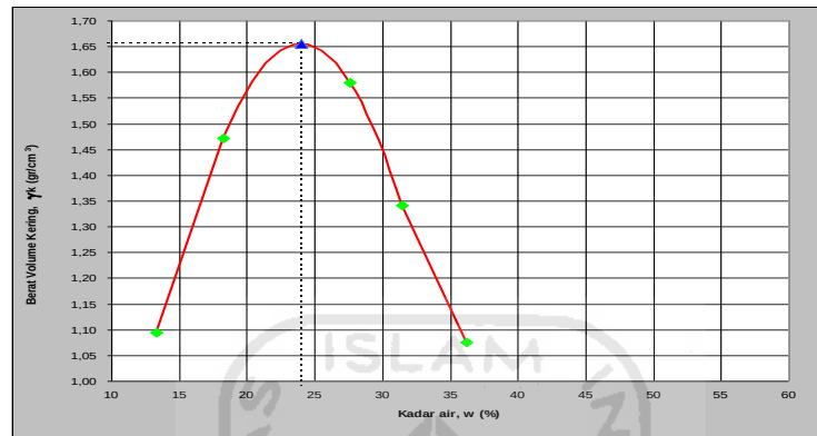
Gambar 5.5 Hasil Pengujian Pemadatan Tanah (Proktor Standar) Sampel I
