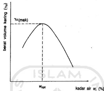
Gambar 3.10 Hubungan berat volume kering dan kadar air
