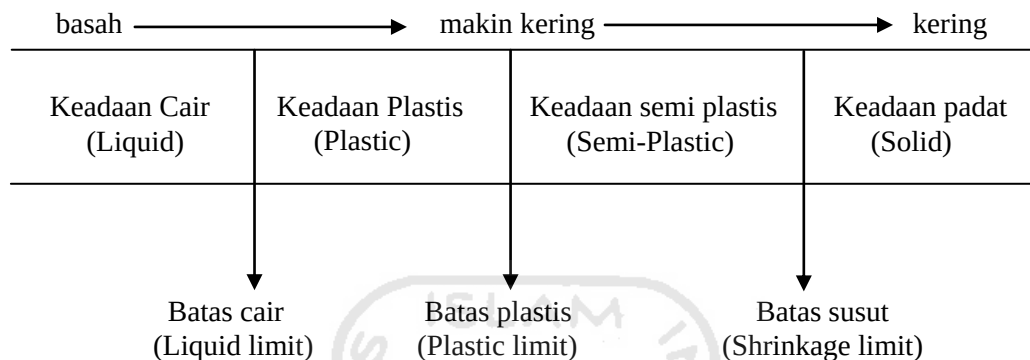
Gambar 3.7 Batas konsistensi tanah
