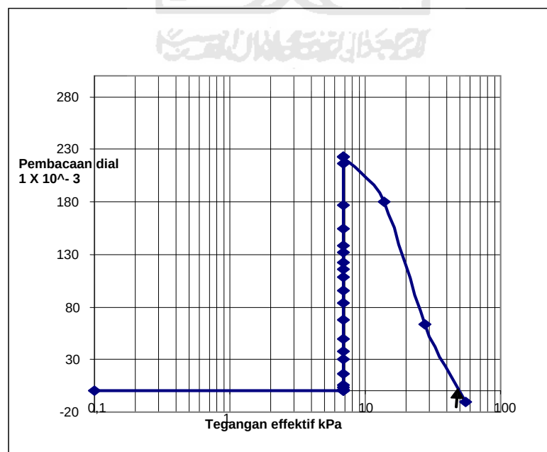
Gambar 5.13 Grafik Tegangan efektif vs Pembacaan dial
