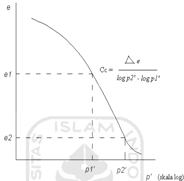
Gambar 3.14 Indeks pemampatan C_c
