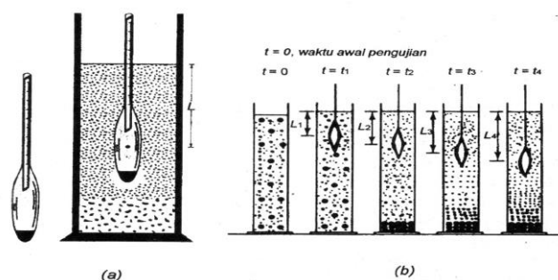
Gambar 3.5 Alat Uji Hidrometer
