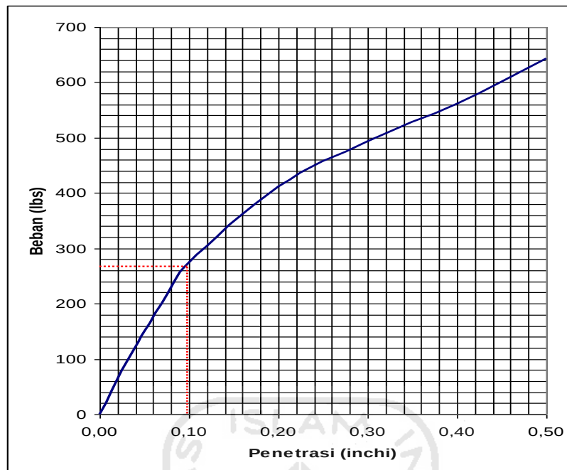
Gambar 5.16 Grafik hubungan beban dan penetrasi uji CBR sampel I
