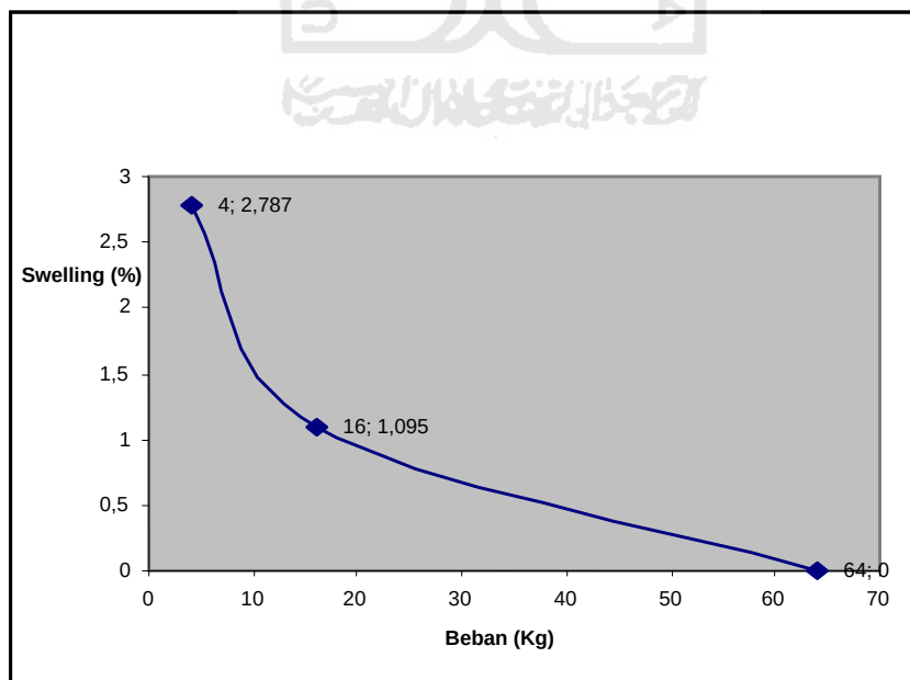
Gambar 6.5 Grafik pengaruh beban terhadap pengembangan (Swelling) sampel A1-B1 dan A2-B2 pada beban 4 kg; 16 kg; dan 64 kg
