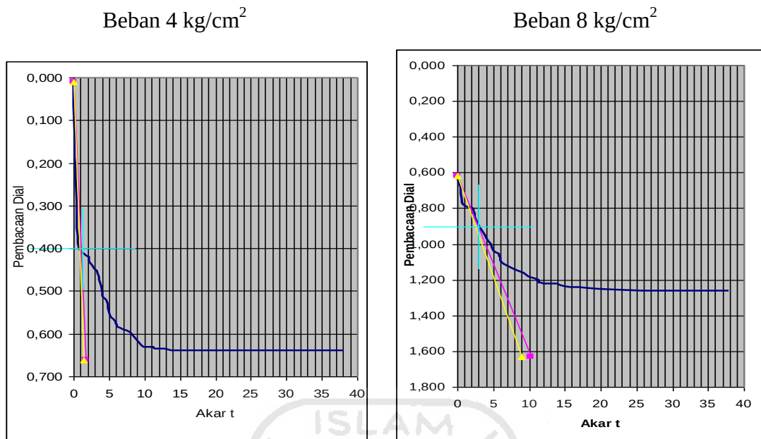
Gambar 5.10 Grafik hubungan antara penurunan & akar waktu beban 4 kg/cm 2 dan 8 kg/cm 2 untuk sampel II
