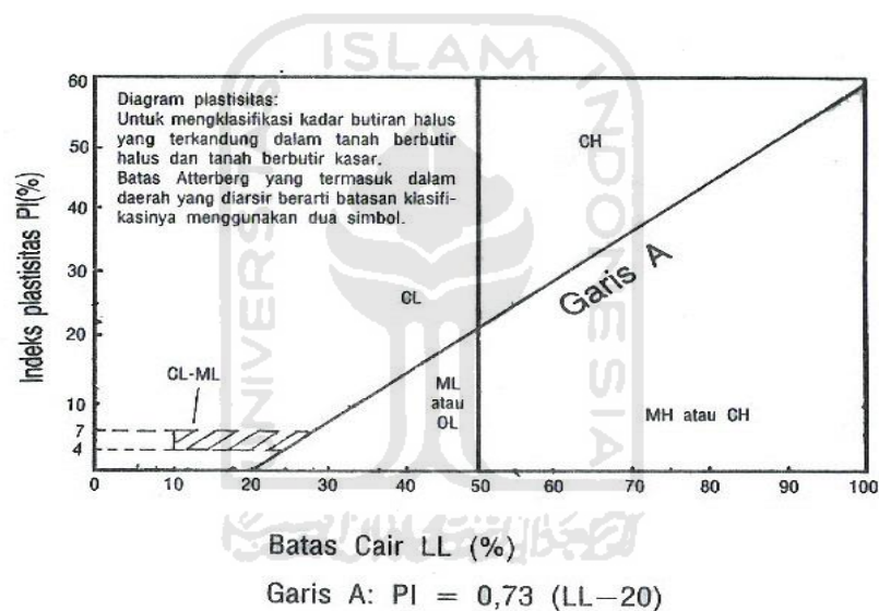
Gambar 3.2 Hubungan antara batas cair dan indeks plastis
