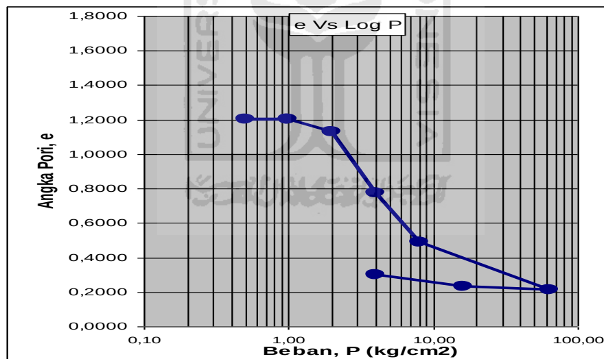
Gambar 5.9 Grafik hubungan beban dan angka pori untuk sampel II
