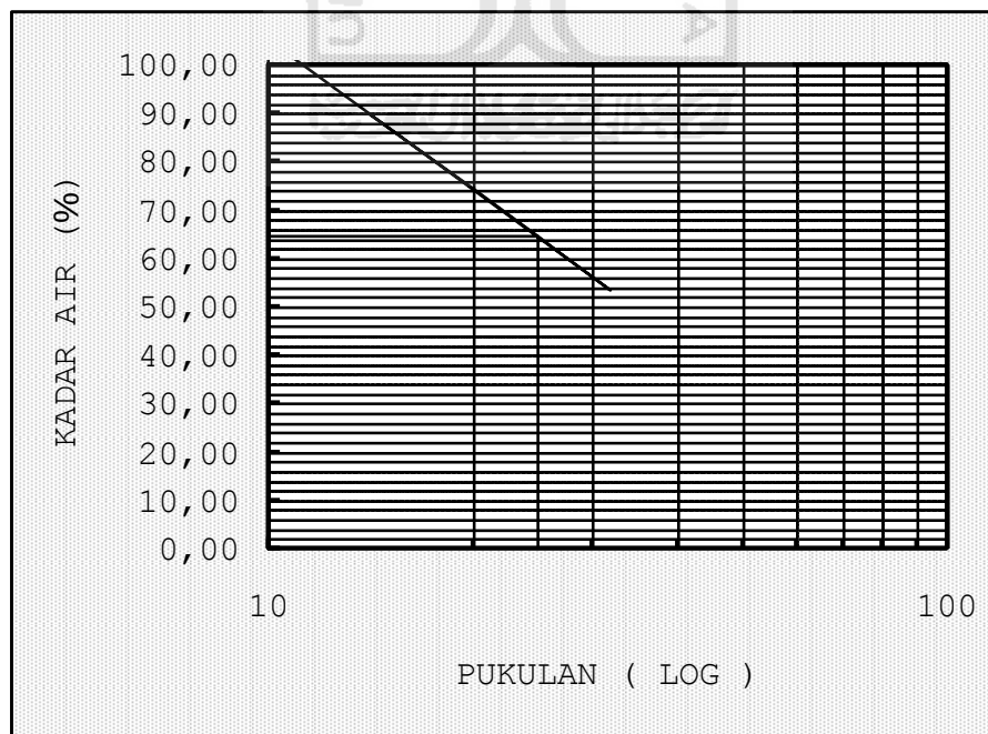
Gambar 5.3 Grafik batas cair sampel I
