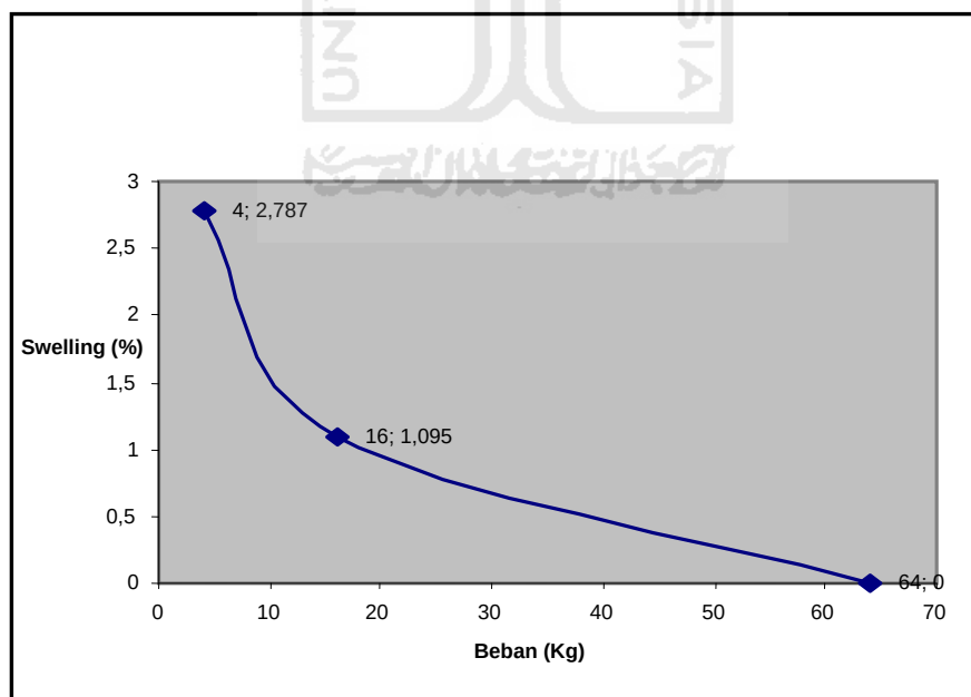
Gambar 5.11 Grafik pengaruh beban terhadap pengembangan (Swelling) sampel A1-B1 dan A2-B2 pada beban 4 kg;16 kg; dan 64 kg.
