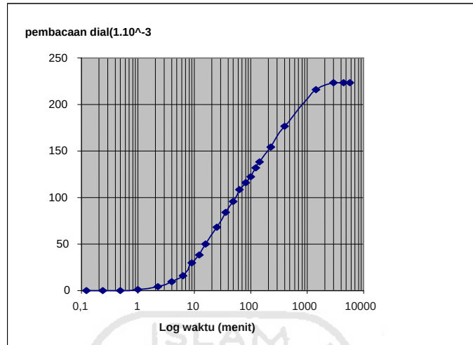
Gambar 6.7 Grafik log waktu vs Swelling
