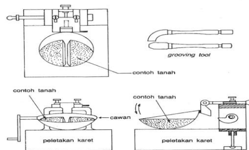
Gambar 3.8 Skema Alat Uji Batas Cair
