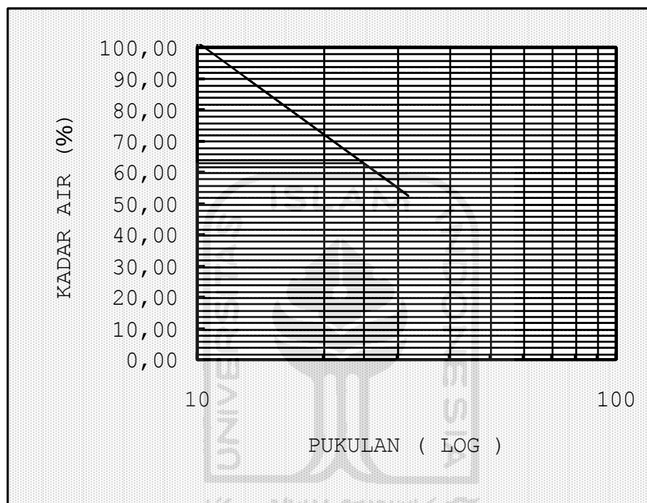
Gambar 5.4 Grafik batas cair sampel II
