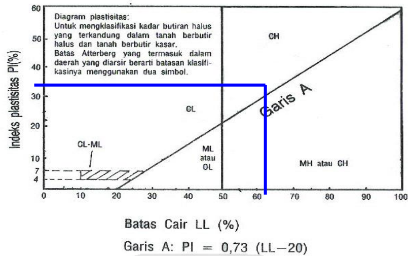
Gambar 6.2 Klasifikasi tanah berdasarkan sistem unified
