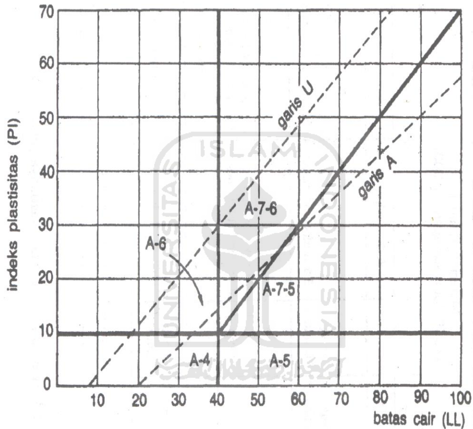
Gambar 3.3 Batas-batas Atterberg untuk subkelompok A-4, A-5, A-6 dan A-7
