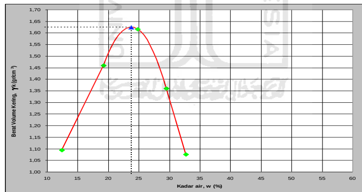
Gambar 5.6 Hasil Pengujian Pemadatan Tanah (Proktor Standar) Sampel II
