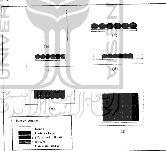
Gambar 3.4 Skema proses pembuatan produk permukaan kasar
