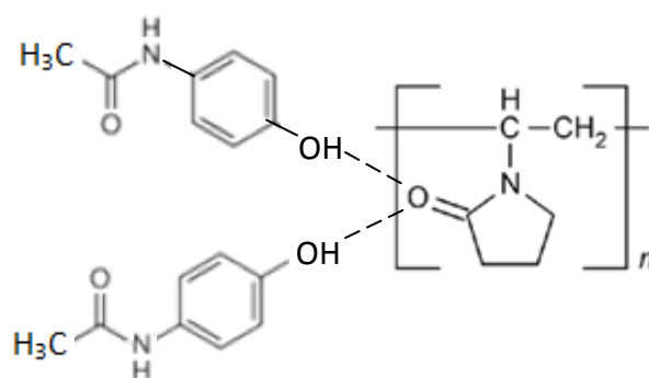
Gambar 16. Pembentukan ikatan hidrogen antara kollidon ® 25 dan parasetamol
