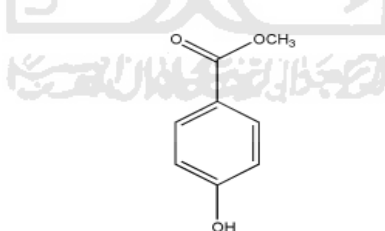
Gambar 5. Struktur kimia metil paraben (26)
