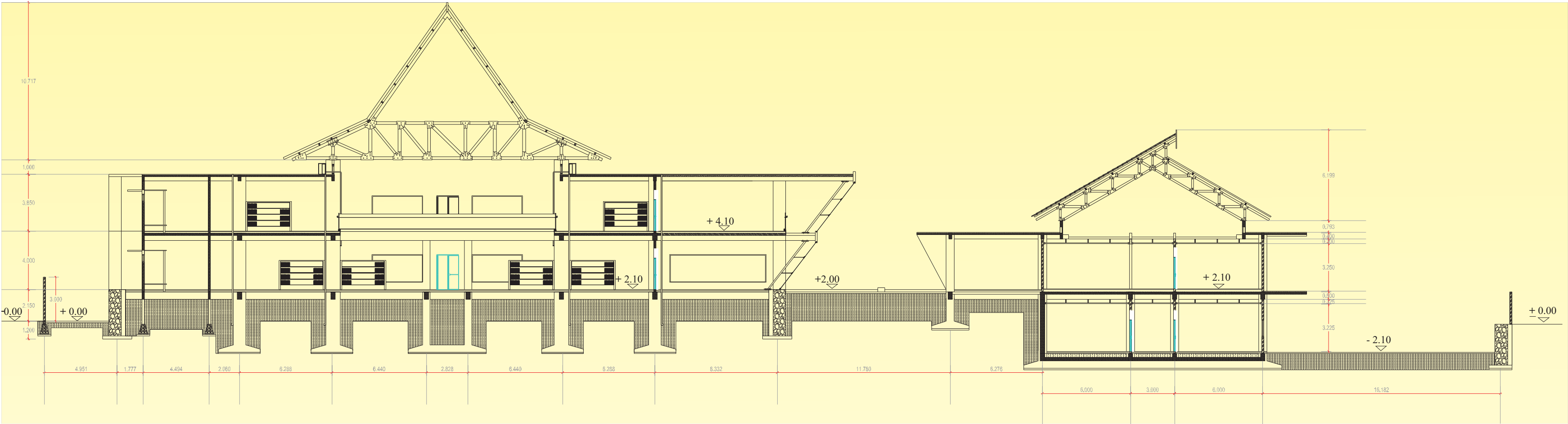
A - A
