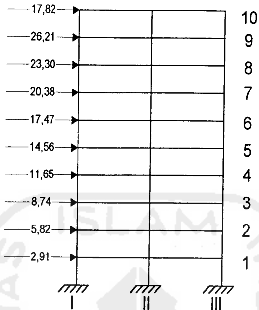
Gambar 4.8. Distribusi beban gempa untuk portal arah Y
