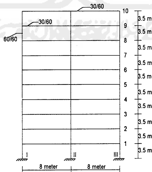
Gambar 4.2. Portal dalam arah Y
