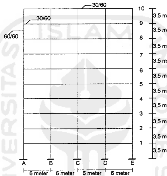
Gambar 4.1. Portal dalam arah X
