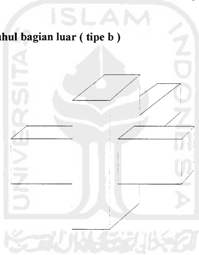
Gambar 4.38 Titik buhul balok kolom luar tipe ( b )
