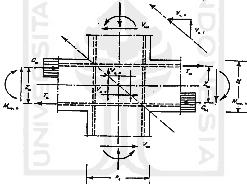
Gambar 3.4. Panel pertemuan balok dan kolom portal dalam kondisi terjadinya sendi-sendi plastis pada kedua ujung balok
