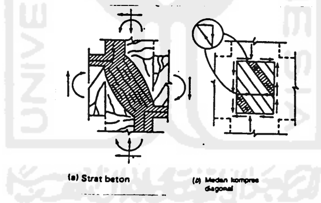
Gambar 4.36. Mekanisme tahanan geser pada titik buhul balok kolom
