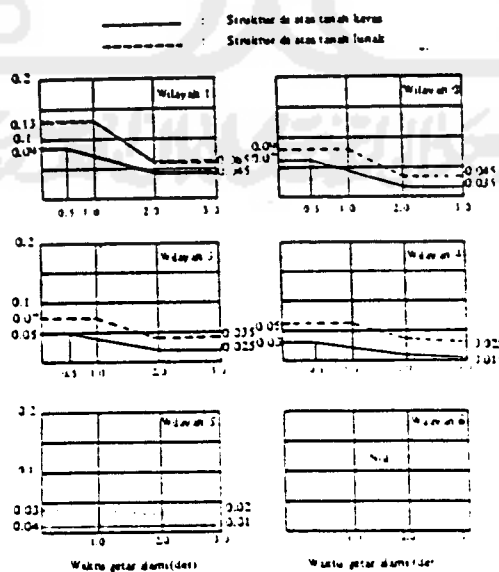
Gambar 2.4. Koefisien gempa dasar untuk berbagai wilayah gempa
