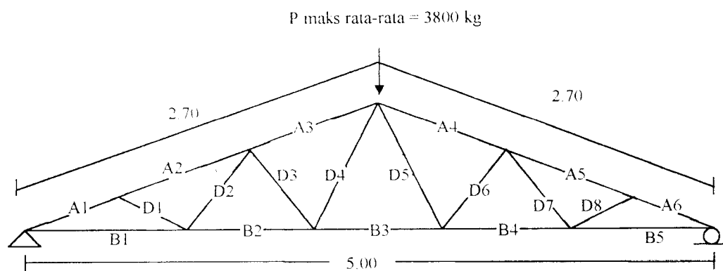
Gambar 5.3 Model Kuda-Kuda Papan Dengan Alat Sambung Claw Nailplate
