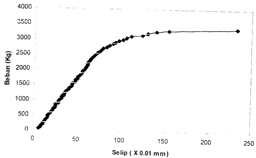
Gambar Grafik Hubungan Beban – Selip alat sambung Claw Nailplate 6 C 3
