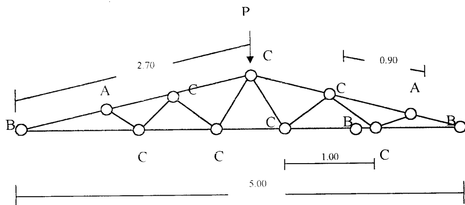
Gambar 4.14 Benda Uji
