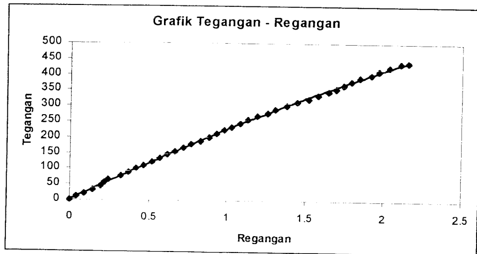
Gambar Grafik Tegangan – Regangan hasil uji desak kayu // serat Sampel 3
