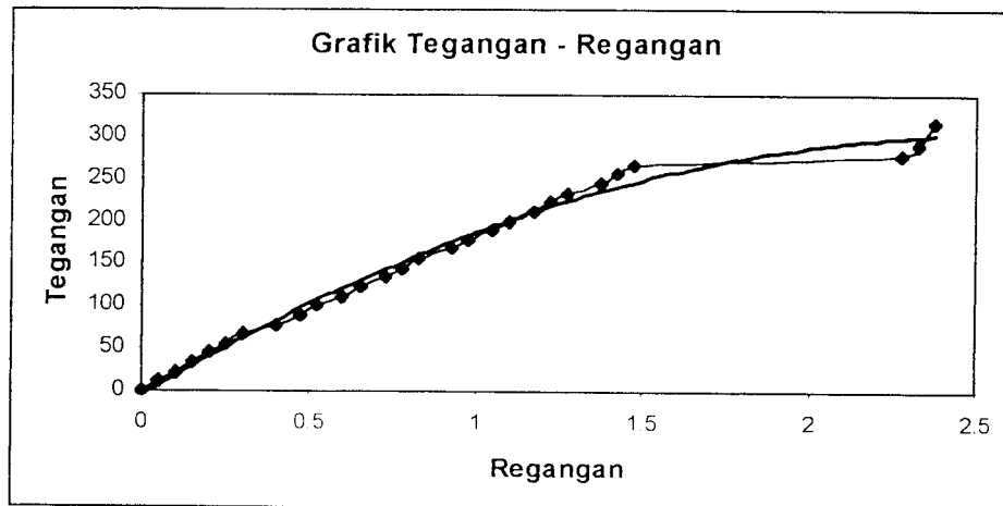
Gambar Grafik Tegangan – Regangan hasil uji desak kayu // serat Sampel 1
