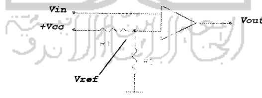
Gambar 2.10 Rangkaian pemanding
