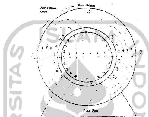
Gambar 2.2 Medan stator pada motor AC
