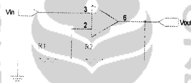
Gambar 2.9 Penguat tidak – membalik
