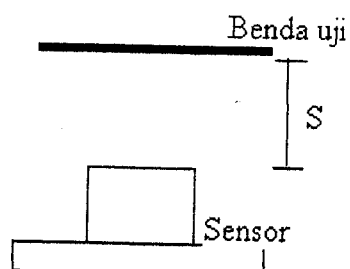
Gambar 4.8 Pengujian jarak sensor ultrasonik
