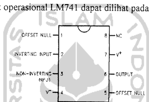
Gambar 2.11 IC LM741
