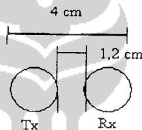
Gambar 4.6 Jarak pemasangan sensor ultrasonik
