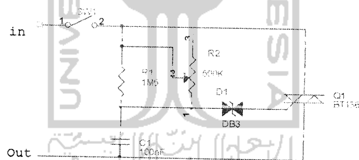
Gambar 3.3 Rangkaian Dimmer
