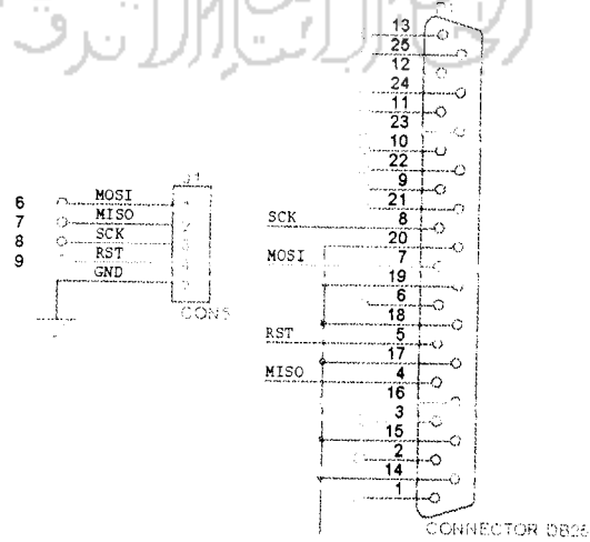
Gambar 3.10 Rangkaian downloader mikrokontroler ATmega16
