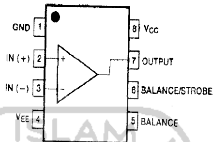
Gambar 2.12 IC LM311.
