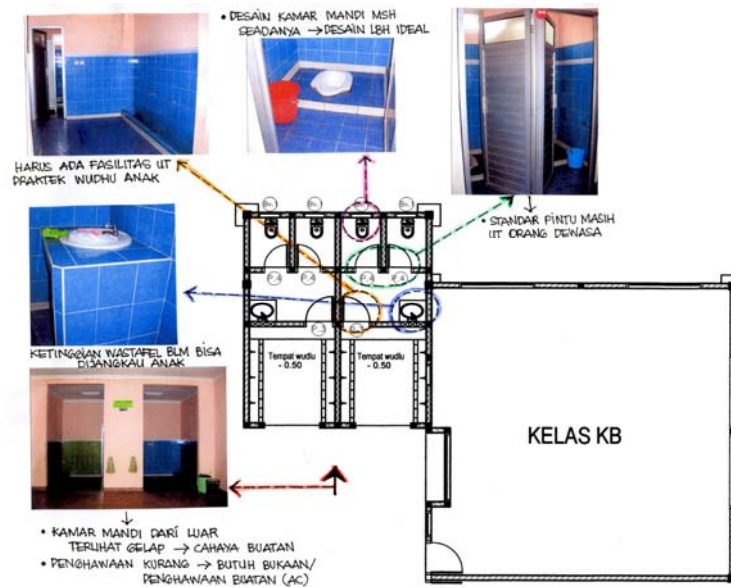
Gb 3.8. Analisa Kamar Mandi Anak
