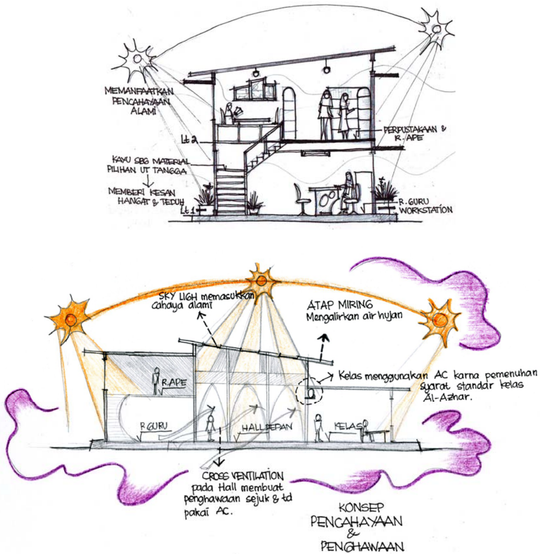
Gb 4.6. Konsep Pncahayaayan dan Penghawaan
