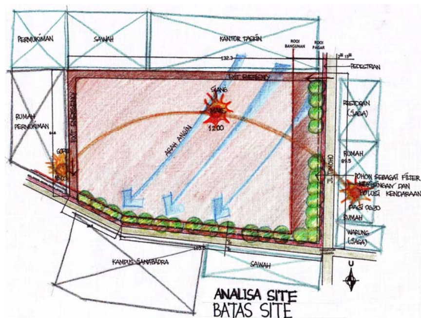
Gb 3.4. Analisa Batas Site
