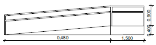
TAMPAK RAMP SKALA 1:50
