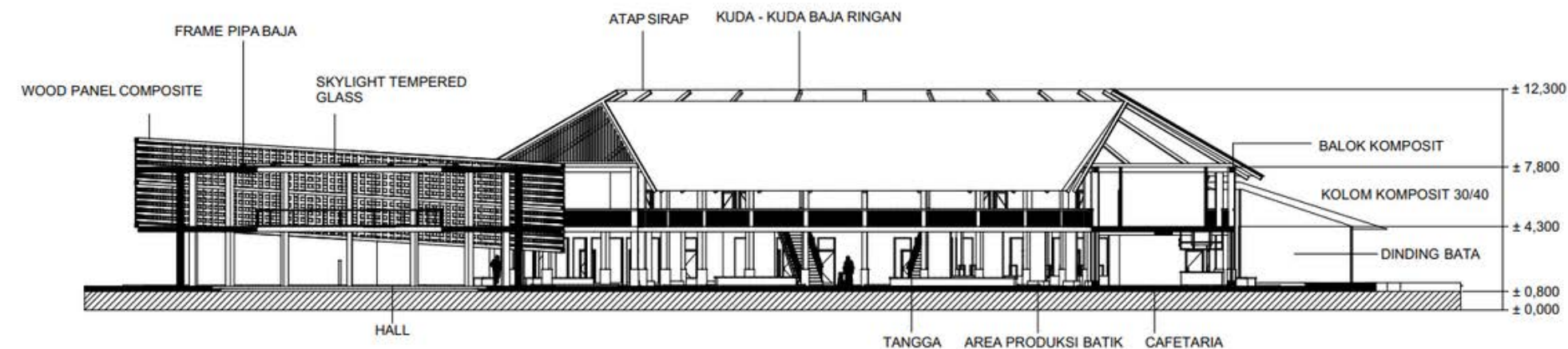
POTONGAN A-A SKALA 1:200
