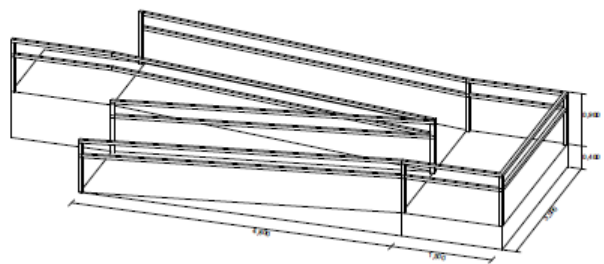
PERSPEKTIF RAMP SKALA 1:50
