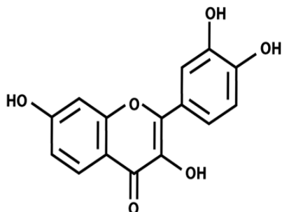
Gambar 4. Struktur Flavonoid
