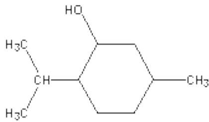
Gambar 10. Struktur Mentol
