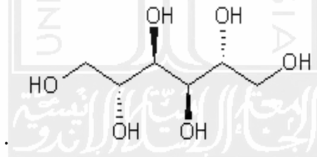
Gambar 7. Struktur Manitol
