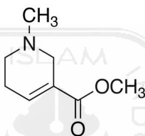
Gambar 3. Struktur Arecoline
